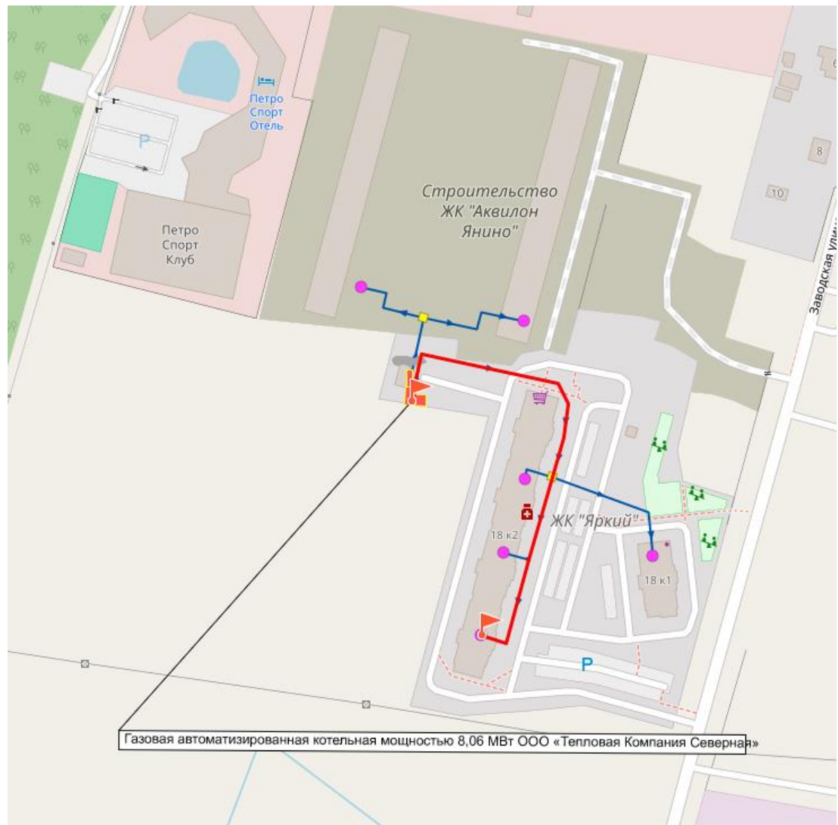
Рисунок 52. . Путь построения пьезометрического графика от котельной от котельной 8,06 МВт ООО «ТК Северная»
