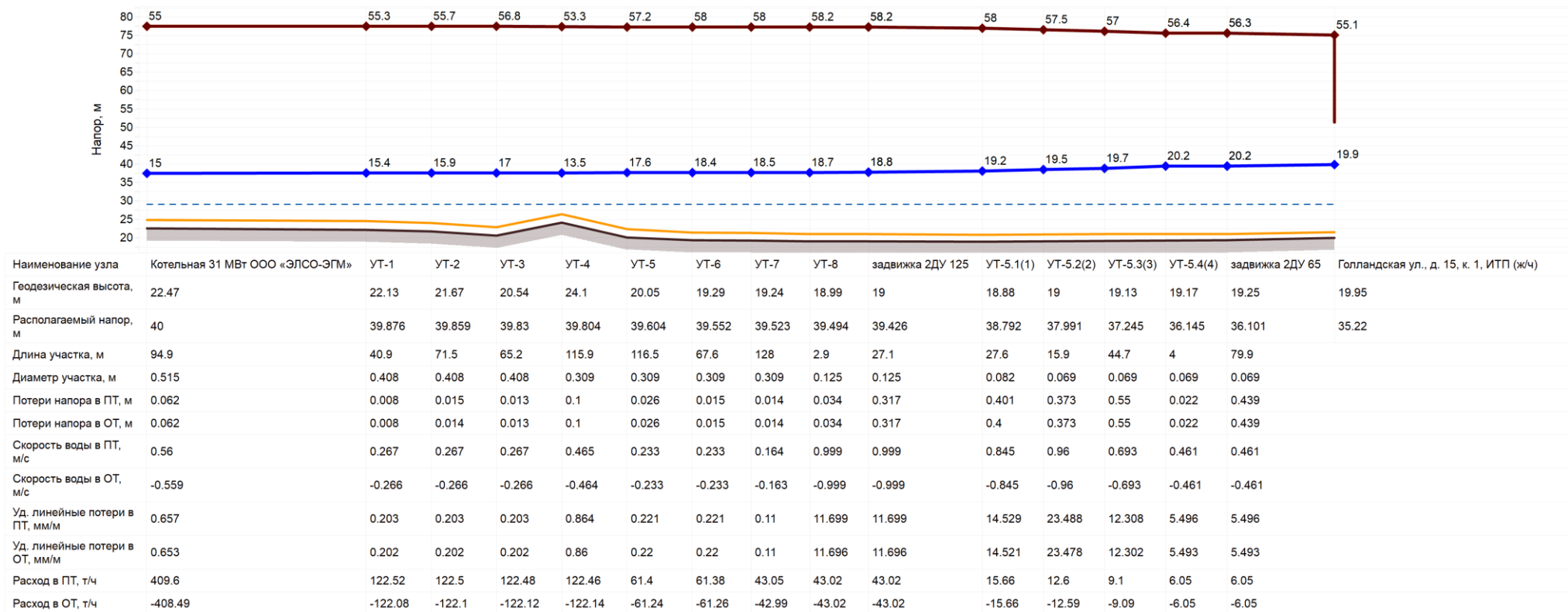
Рисунок 45. Пьезометрический график от котельной 31 МВт ООО «ЭЛСО-ЭГМ»
