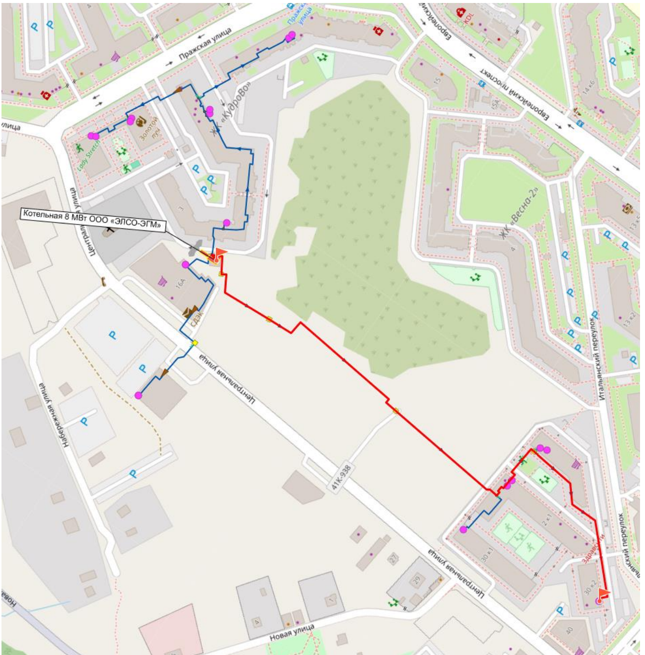
Рисунок 42. Путь построения пьезометрического графика от котельной 8 МВт ООО «ЭЛСО-ЭГМ»
