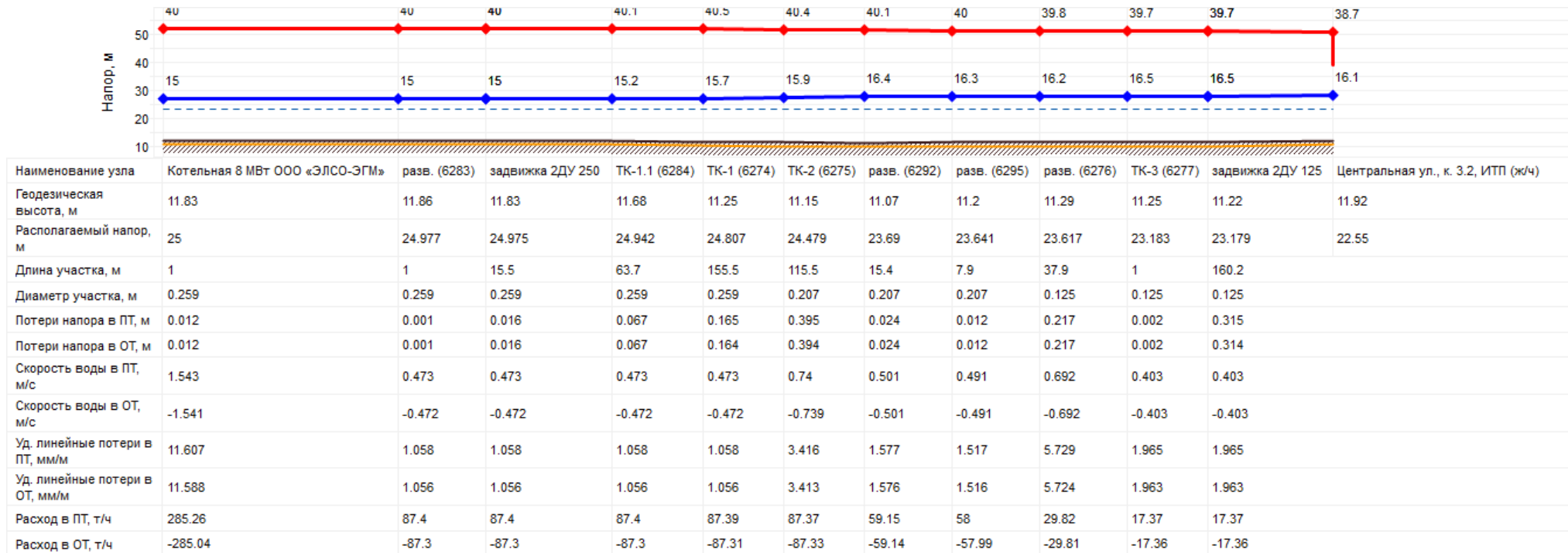
Рисунок 43. Пьезометрический график от котельной 8 МВт ООО «ЭЛСО-ЭГМ»
