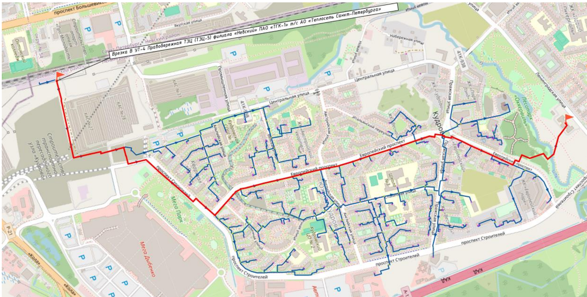
Рисунок 28. Путь построения пьезометрического графика от Правобережной ТЭЦ-5
