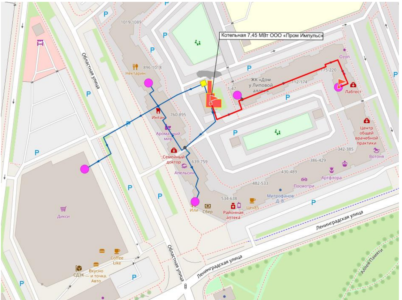
Рисунок 40. Путь построения пьезометрического графика от котельной 7,45 МВт
