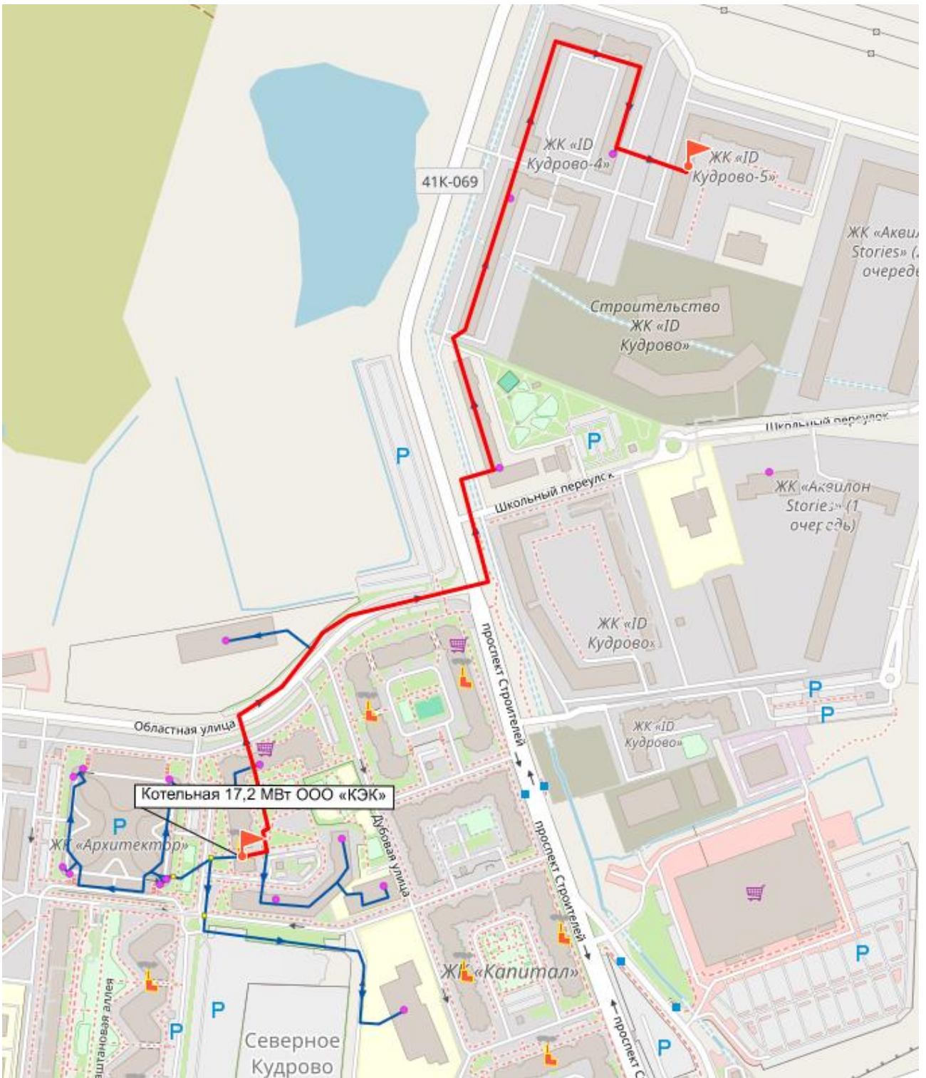
Рисунок 34. Путь построения пьезометрического графика от котельной 17,2 МВт ООО «КЭК».
