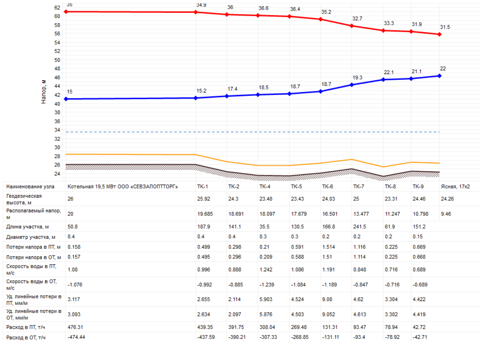
Рисунок 49. . Пьезометрический график от котельной от котельной 19,5 МВт ООО «СЕВЗАПОПТТОРГ»
