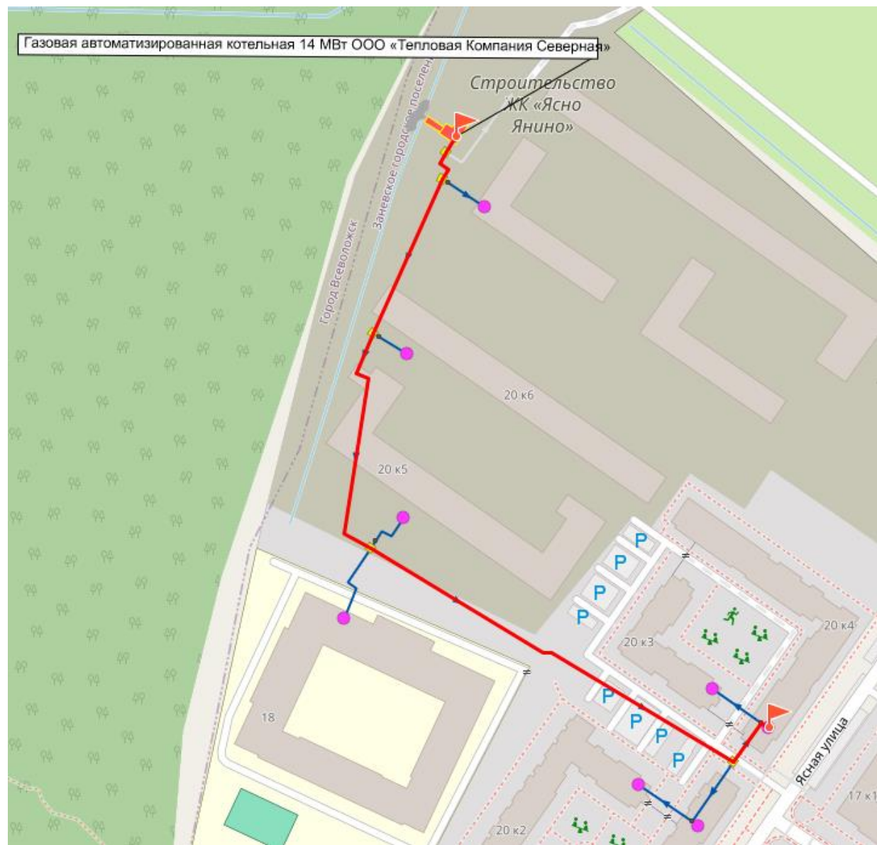
Рисунок 50. Путь построения пьезометрического графика от котельной от котельной 14 МВт ООО «ТК Северная»
