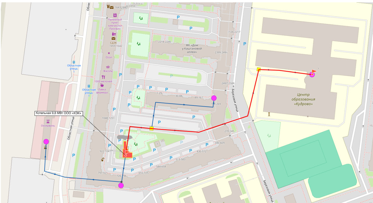
Рисунок 32. Путь построения пьезометрического графика от котельной 9,8 МВт ООО «КЭК».
