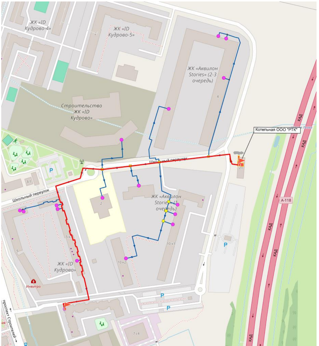
Рисунок 46. Путь построения пьезометрического графика от котельной ООО «РТК»
