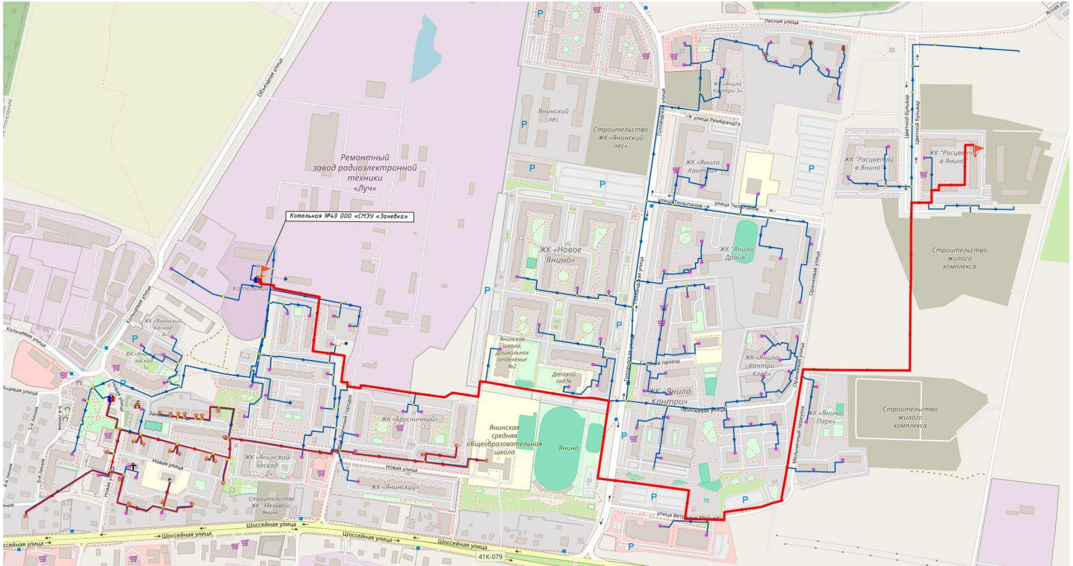
Рисунок 26. Путь построения пьезометрического графика от котельной 40 ООО «СМЭУ «Заневка» система 110/70 °С
