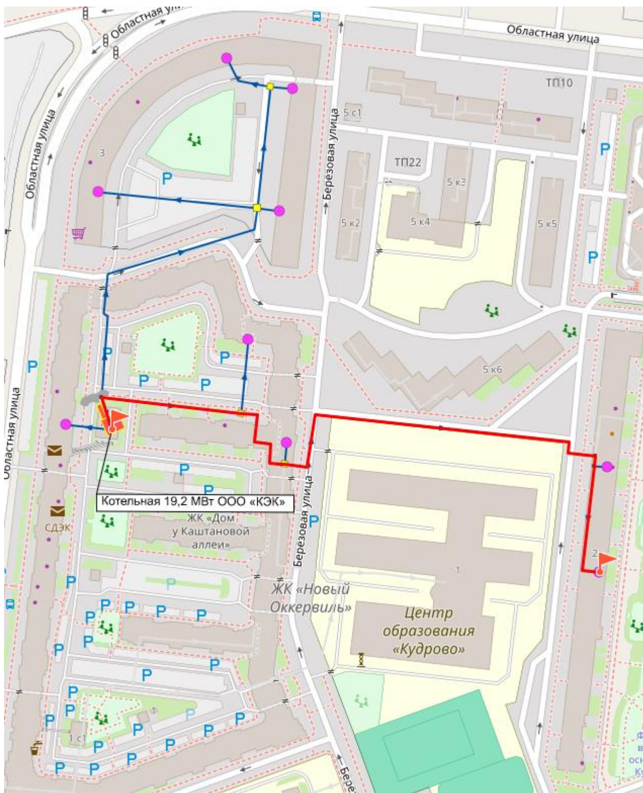
Рисунок 36. Путь построения пьезометрического графика от котельной 19,2 МВт ООО «КЭК»
