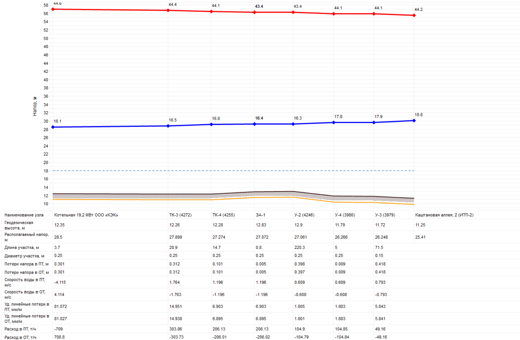
Рисунок 37. Пьезометрический график от котельной 19,2 МВт ООО «КЭК»
