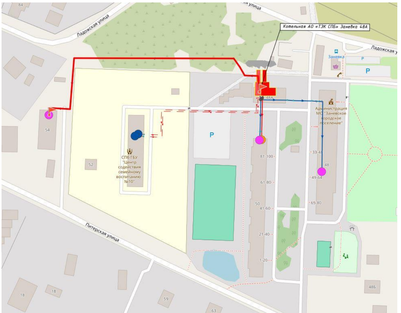
Рисунок 30. Путь построения пьезометрического графика от котельной АО «ТЭК СПб» Заневка 48А.
