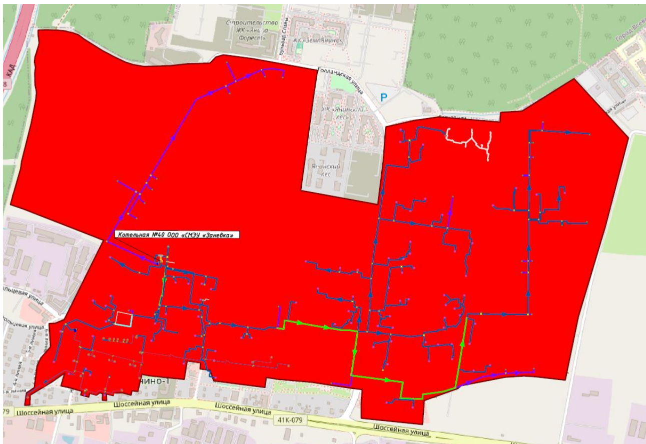
Рисунок 16. Перспективная зона действия котельной № 40 ООО «СМЭУ «Заневка»
