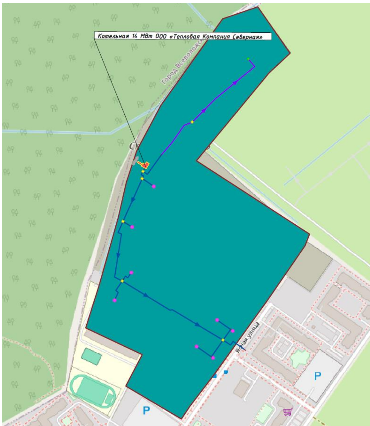
Рисунок 33. Перспективная зона действия новой котельной 14 МВт ООО «ТК Северная»
