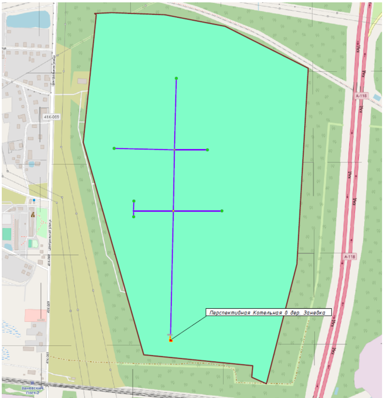
Рисунок 30. Перспективная зона действия котельной в дер. Заневка
