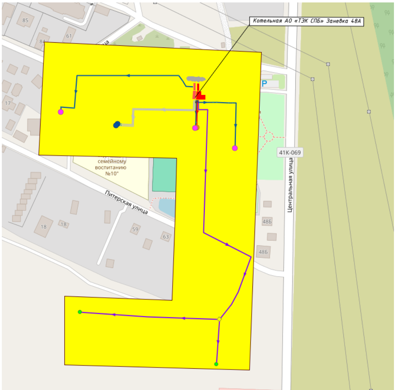
Рисунок 18. Перспективная зона действия котельной АО «ТЭК СПб»
