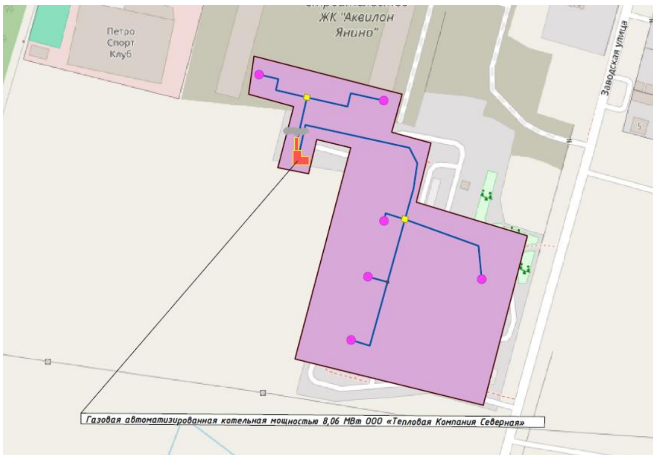
Рисунок 15. Зона действия и тепловые сети котельной ООО «Тепловая Компания Северная»
