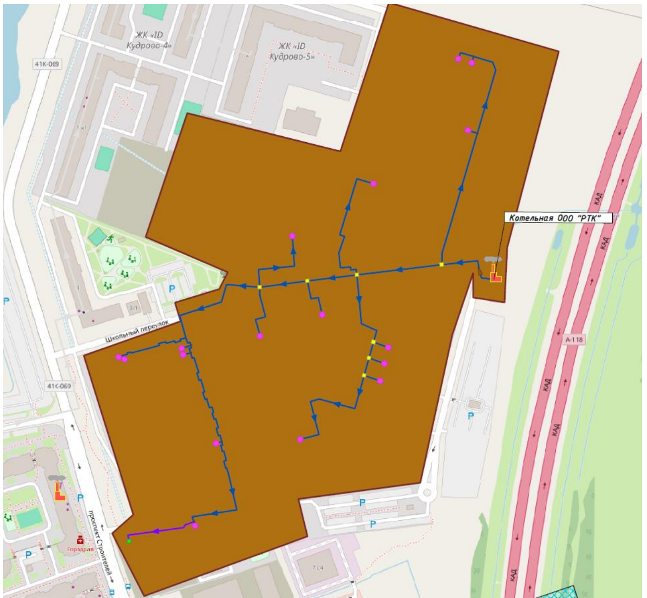
Рисунок 29. Перспективная зона действия котельной ООО «РТК»
