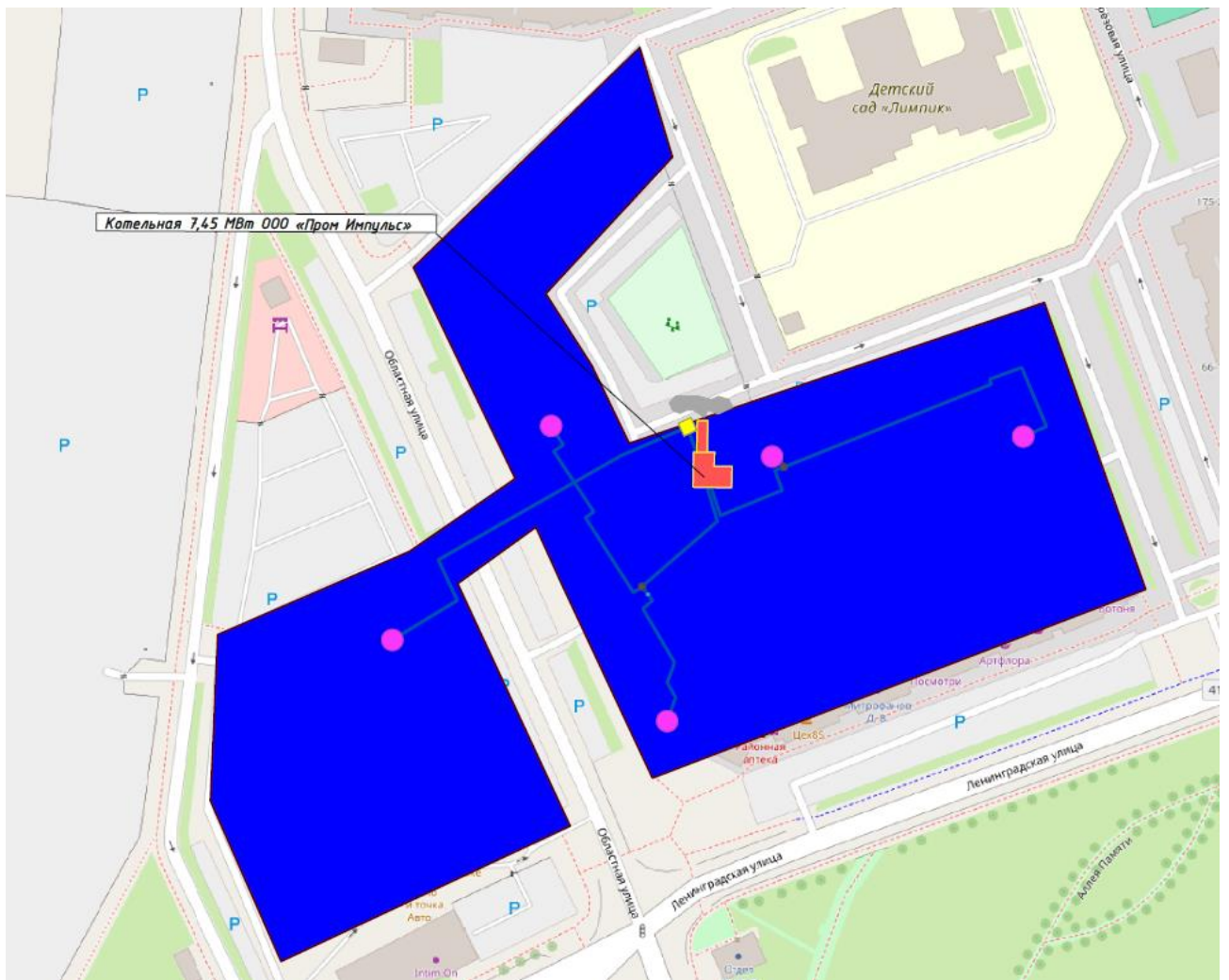
Рисунок 13. Зона действия и тепловые сети котельной 7,45 МВт ООО «Пром Импульс»
