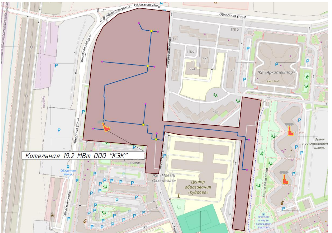
Рисунок 25. Перспективная зона действия котельной 19,2 МВт ООО «КЭК»
