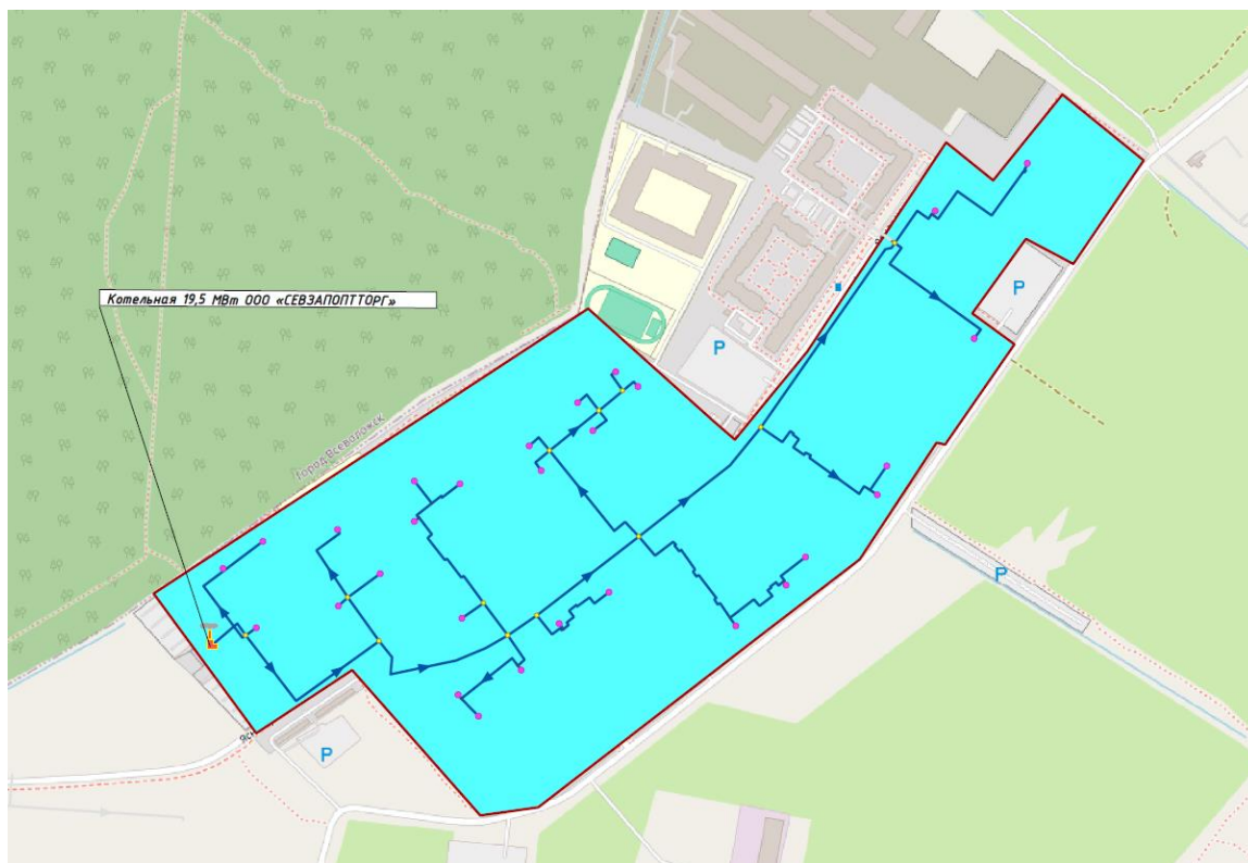
Рисунок 21. Перспективная зона действия новой котельной 19,5 МВт ООО «СЕВЗАПОПТТОРГ»
