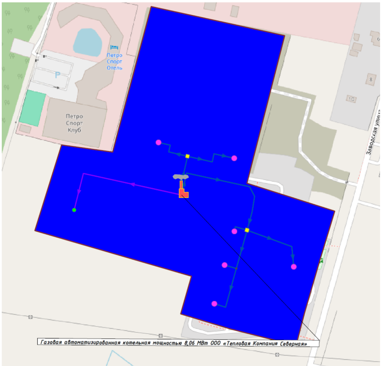
Рисунок 23. Перспективная зона действия котельной 8,06 МВт ООО «Тепловая Компания Северная»
