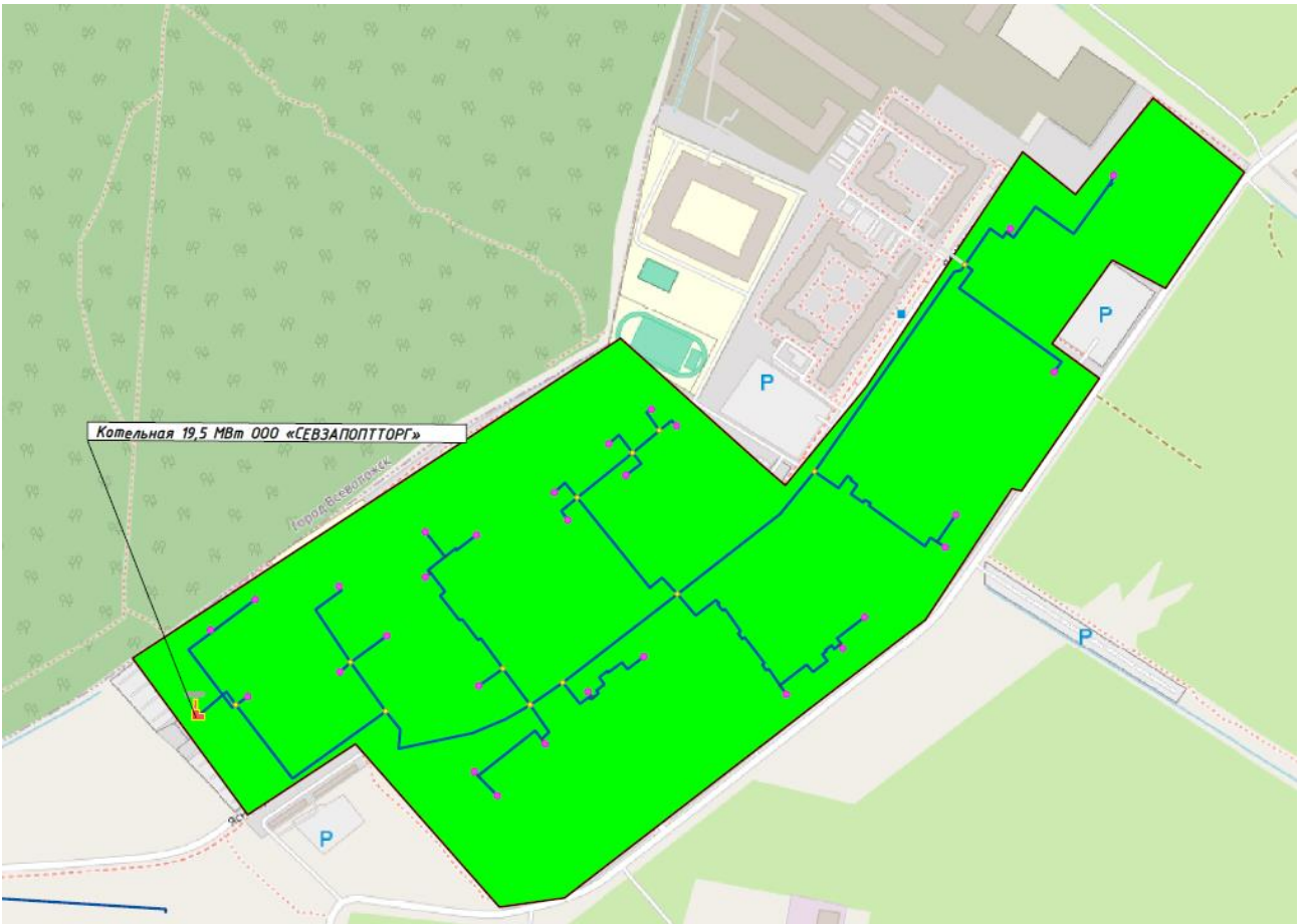
Рисунок 9. Зона действия и тепловые сети котельной 19,5 ООО «СЕВЗАПОПТТОРГ»
