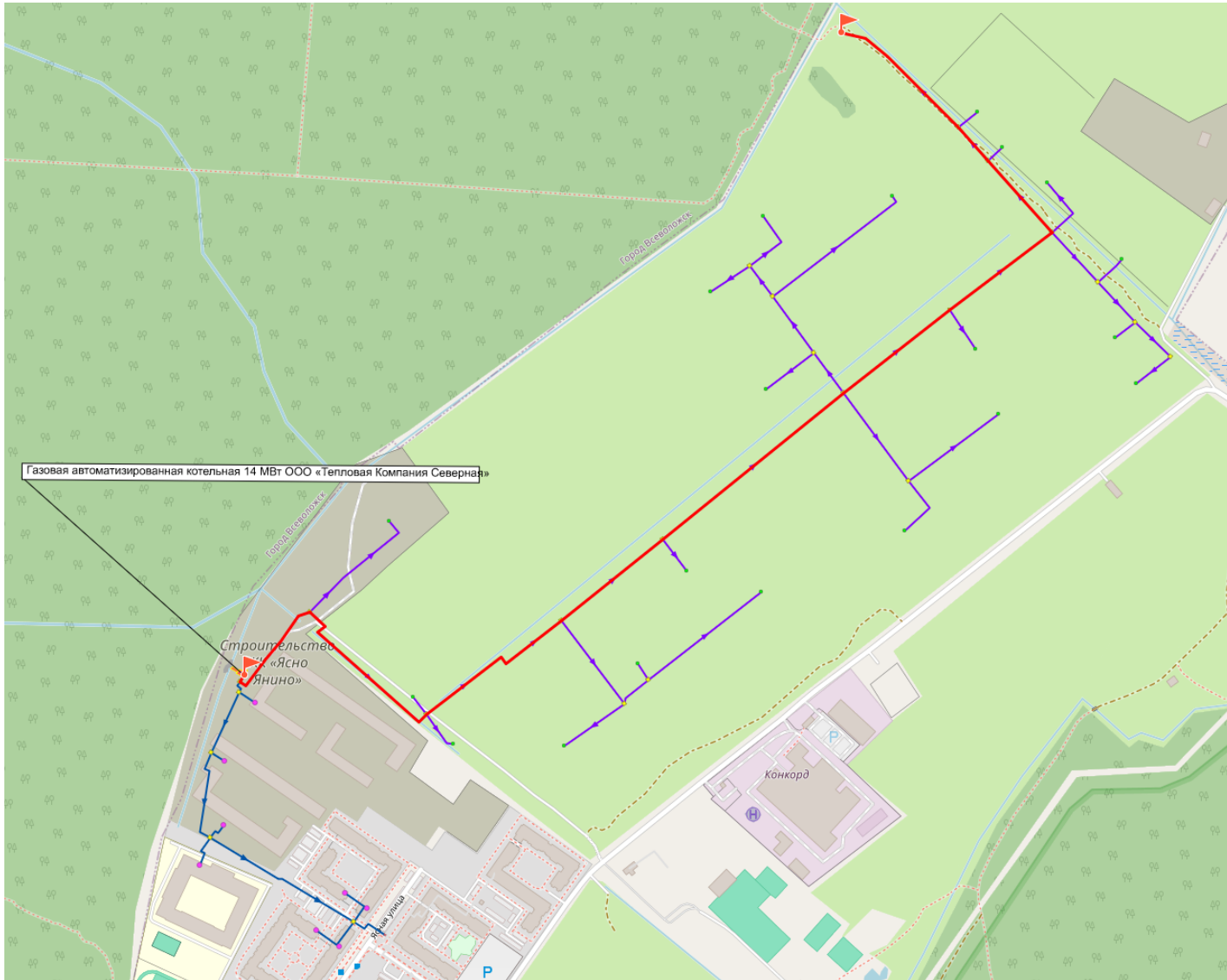
Рисунок 10. Путь построения пьезометрического графика от котельной 14 МВт ООО «ТК Северная» до потребителя Объект продажи товаров (сценарий №1а)
