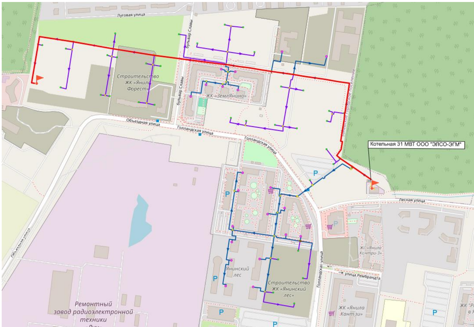
Рисунок 4. Путь построения пьезометрического графика от котельной 31 МВт ООО «ЭЛСО-ЭГМ» до потребителя 12-я оч.,
