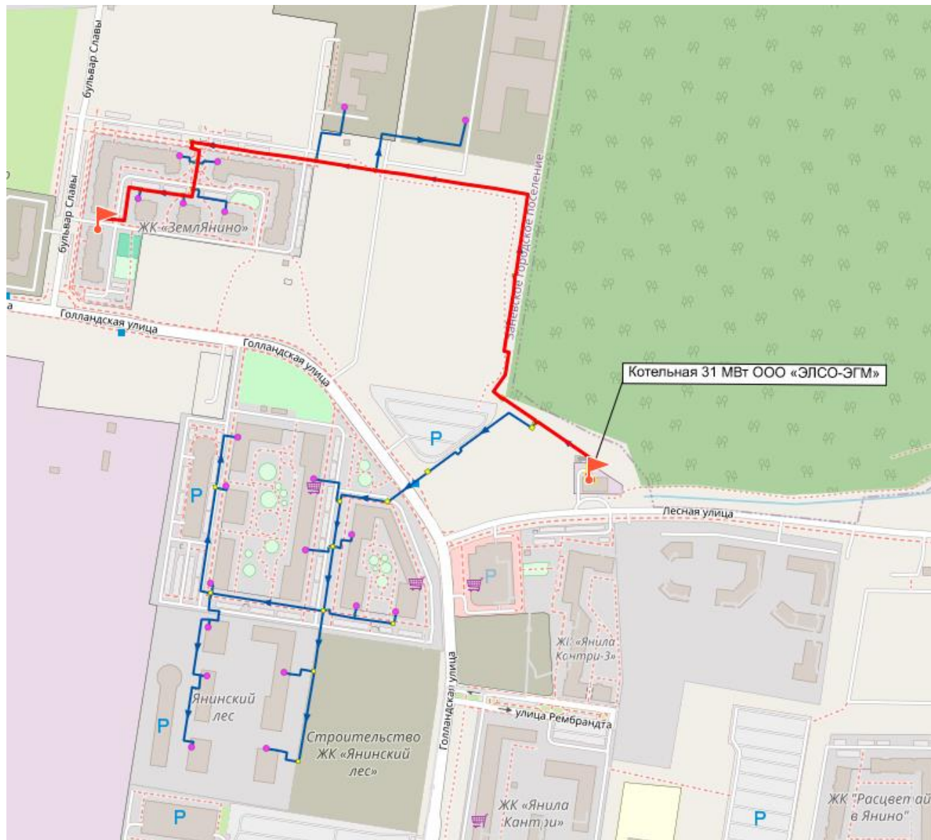
Рисунок 45. Пьезометрический график от котельной 31 МВт ООО «ЭЛСО-ЭГМ»
