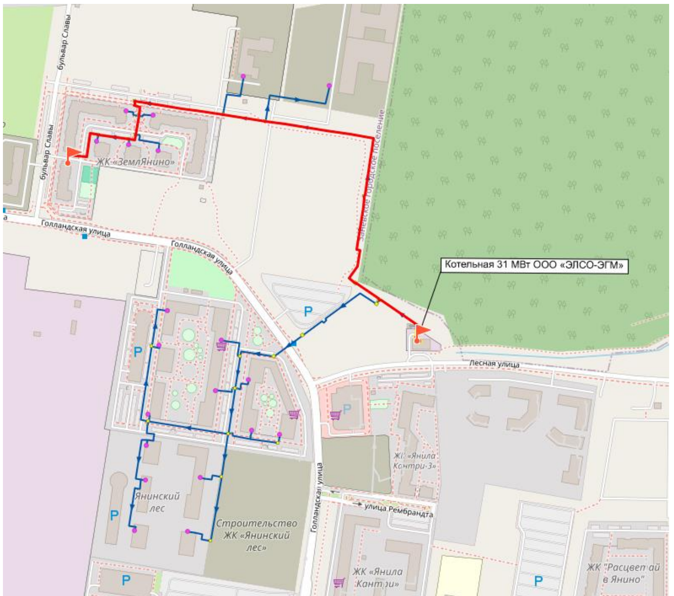
Рисунок 44. Путь построения пьезометрического графика от котельной 31 МВт ООО «ЭЛСО-ЭГМ»
