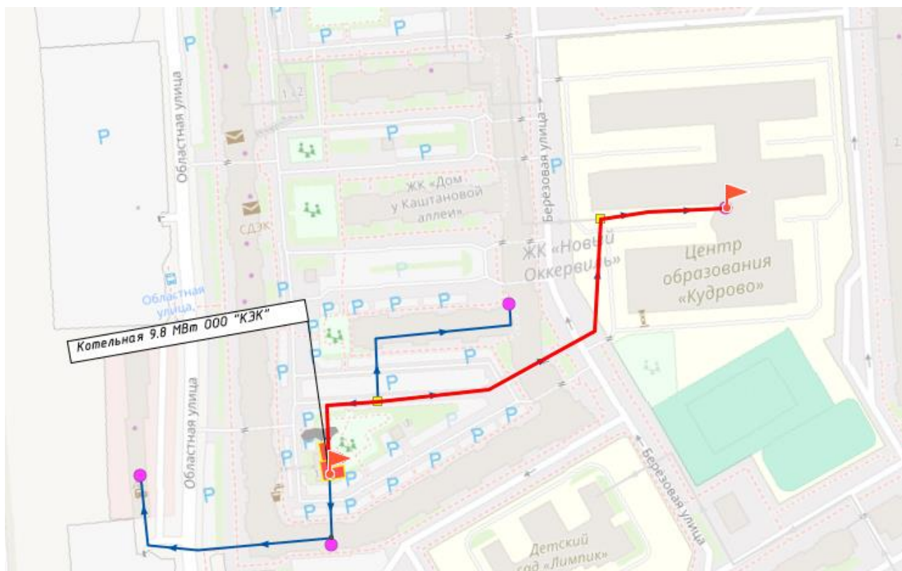
Рисунок 32. Путь построения пьезометрического графика от котельной 9,8 МВт ООО «КЭК».
