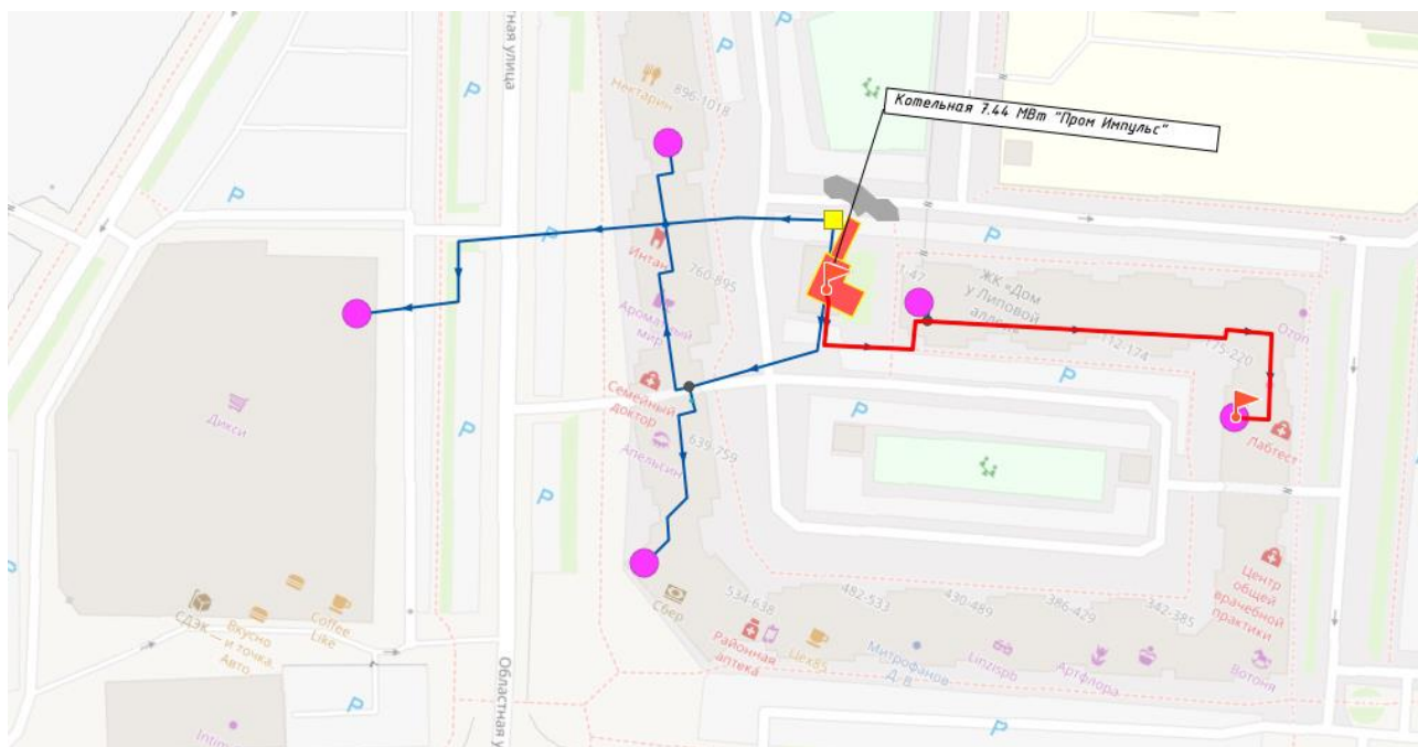
Рисунок 40. Путь построения пьезометрического графика от котельной 7,44 МВт
