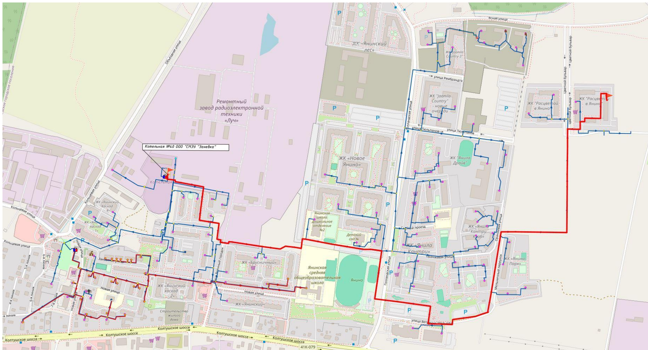
Рисунок 26. Путь построения пьезометрического графика от котельной 40 ООО «СМЭУ «Заневка» система 110/70 °С
