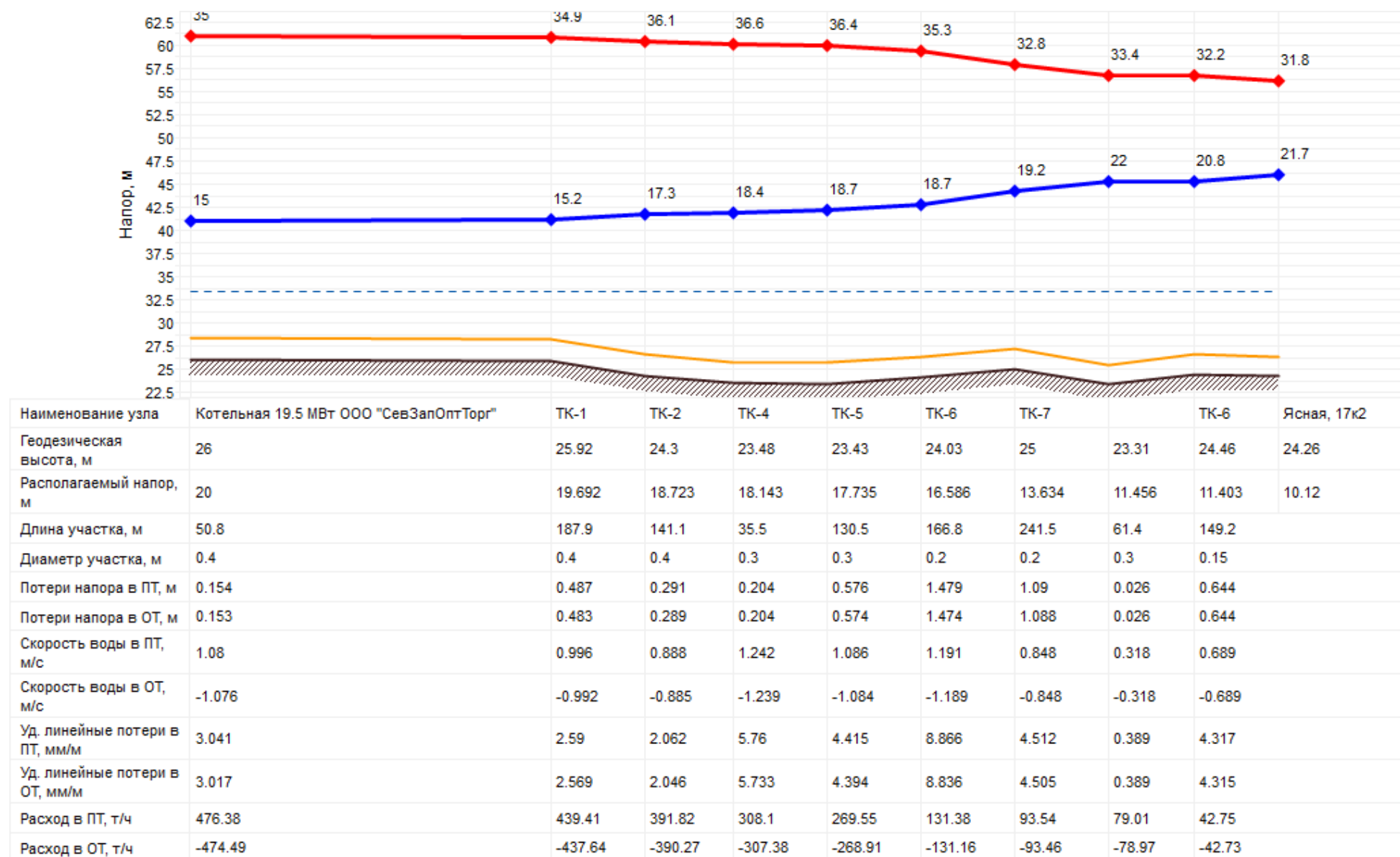
Рисунок 49. . Пьезометрический график от котельной от котельной 19,5 МВт ООО «СЕВЗАПОПТТОРГ»
