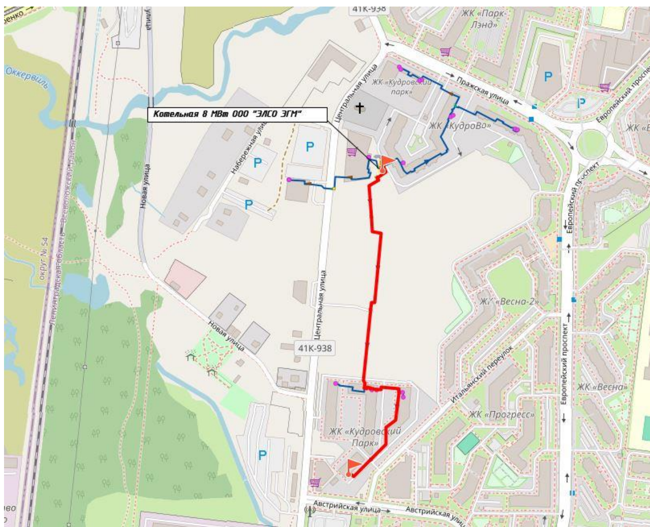
Рисунок 42. Путь построения пьезометрического графика от котельной 8 МВт ООО «ЭЛСО-ЭГМ»
