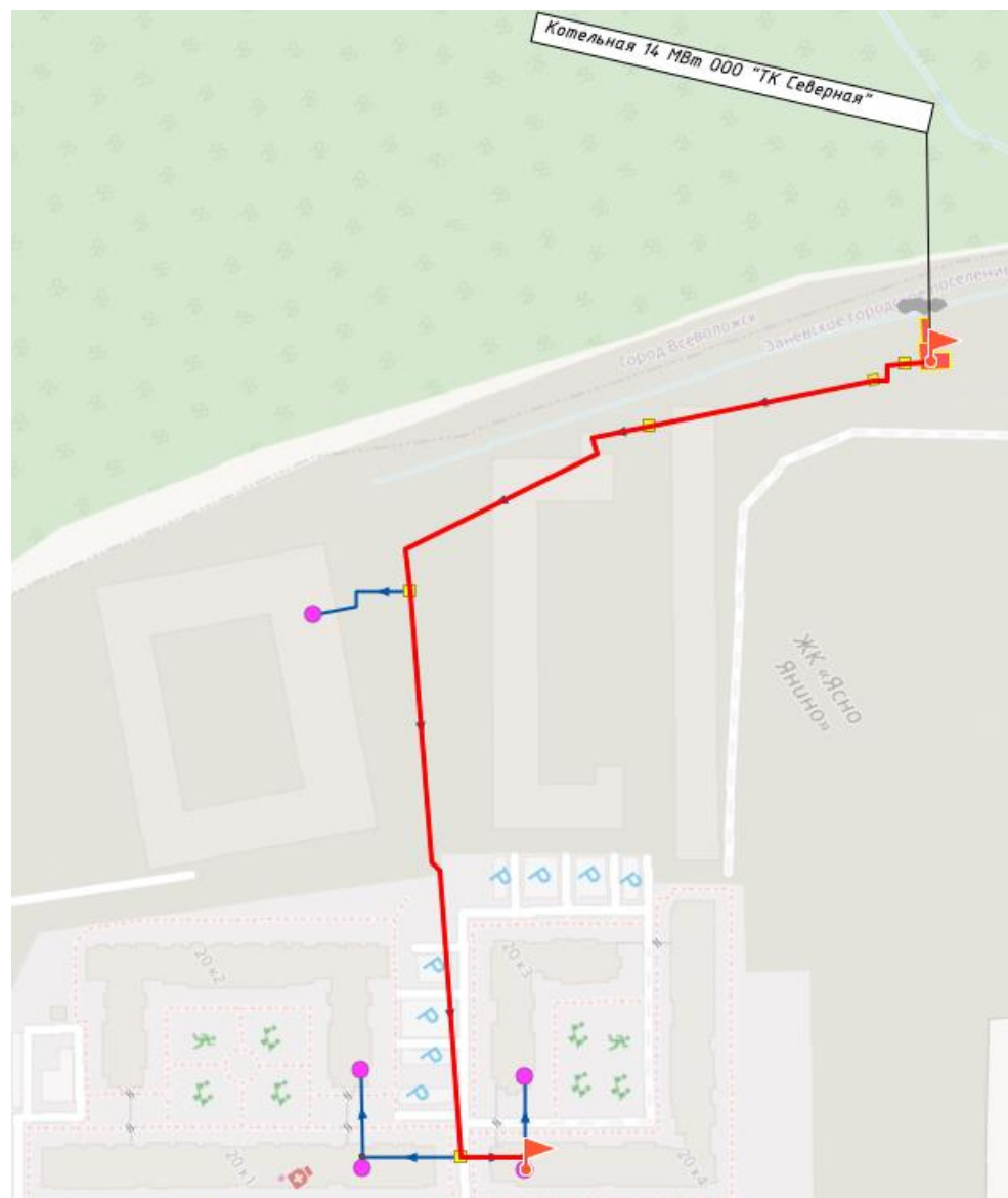
Рисунок 50. . Путь построения пьезометрического графика от котельной от котельной 14 МВт ООО «ТК Северная»
