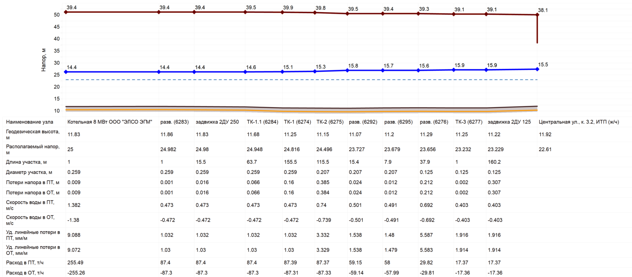
Рисунок 43. Пьезометрический график от котельной 8 МВт ООО «ЭЛСО-ЭГМ»
