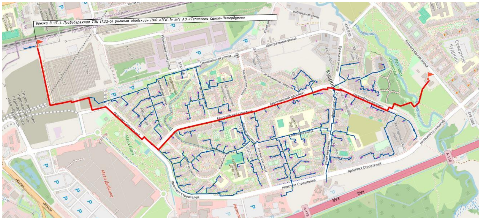
Рисунок 28. Путь построения пьезометрического графика от Правобережной ТЭЦ-5.
