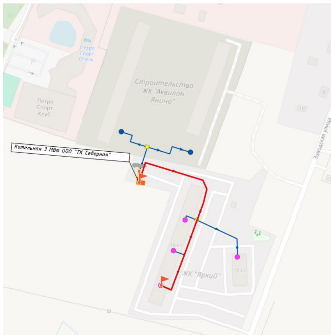
Рисунок 52. . Путь построения пьезометрического графика от котельной от котельной 3 МВт ООО «ТК Северная»
