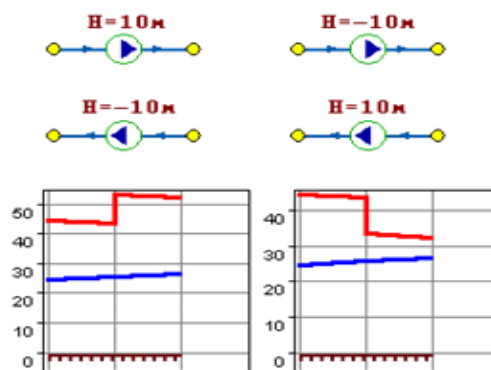
Рисунок 16. Пьезометрические графики
