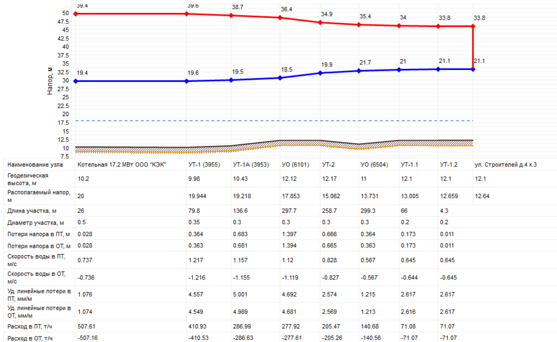
Рисунок 35. Пьезометрический график от котельной 17,2 МВт ООО «КЭК»
