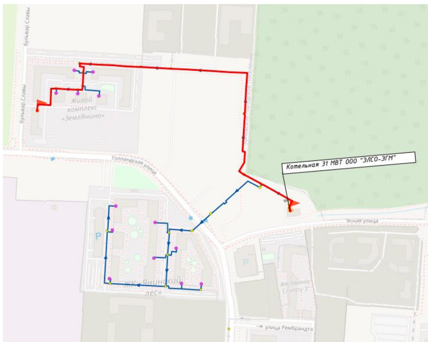
Рисунок 44. Путь построения пьезометрического графика от котельной 31 МВт ООО «ЭЛСО-ЭГМ»
