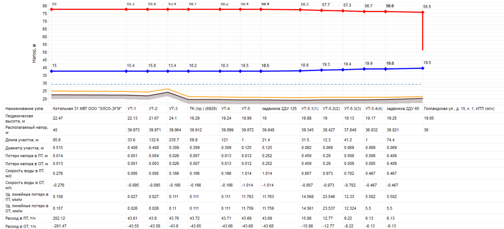
Рисунок 45. Пьезометрический график от котельной 31 МВт ООО «ЭЛСО-ЭГМ»
