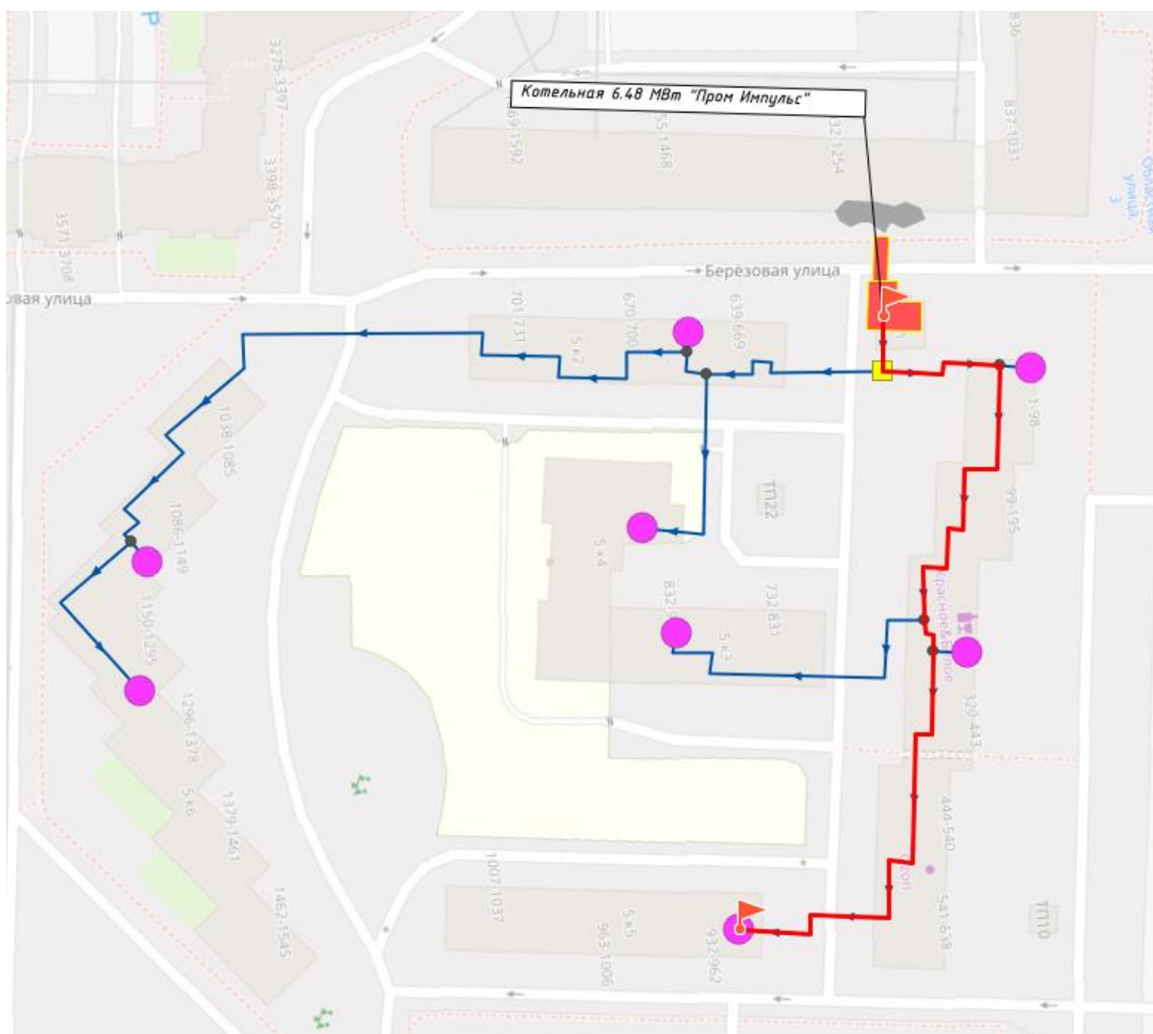
Рисунок 38. Путь построения пьезометрического графика от котельной 6,48 МВт ООО «Пром Импульс»
