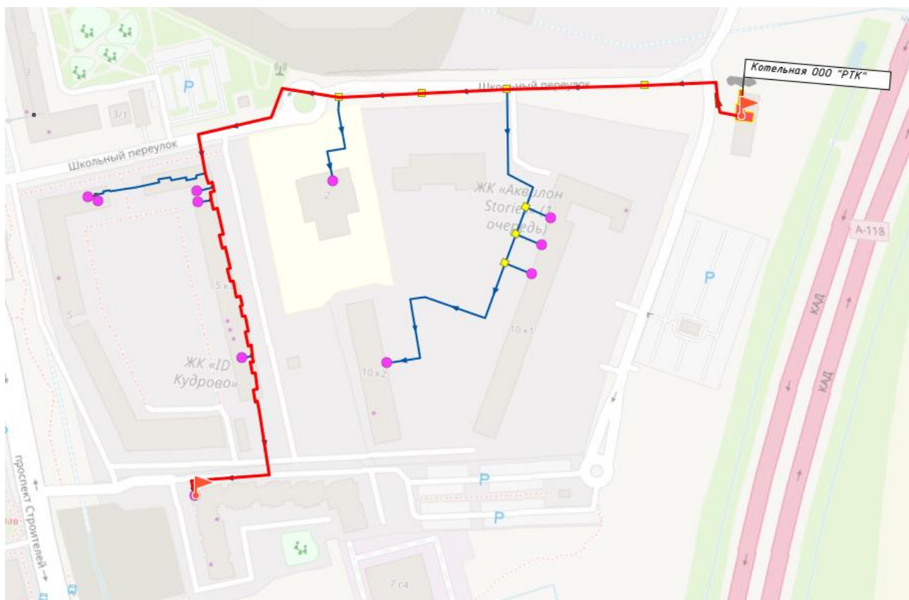
Рисунок 46. Путь построения пьезометрического графика от котельной ООО «РТК»
