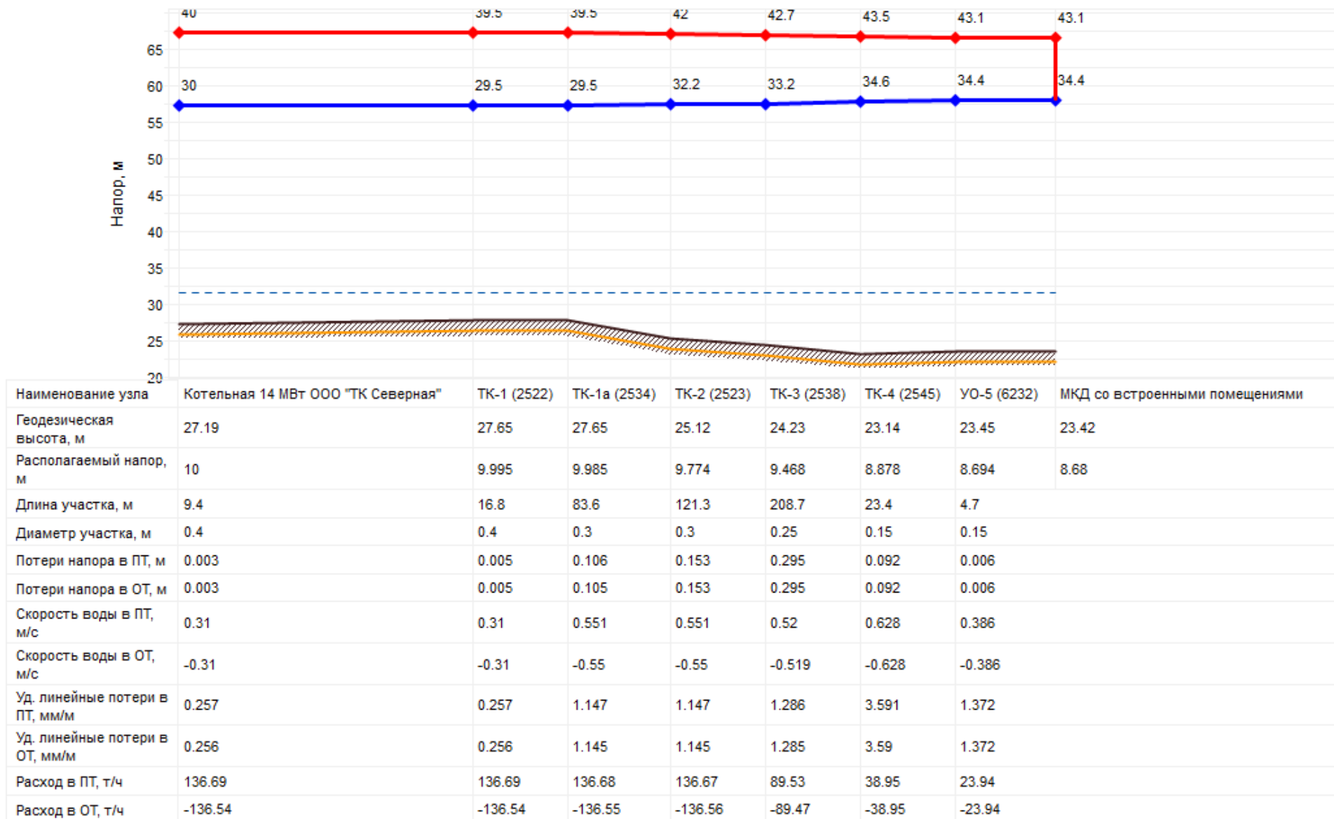
Рисунок 51. . Пьезометрический график от котельной от котельной 14 МВт ООО «ТК Северная»
