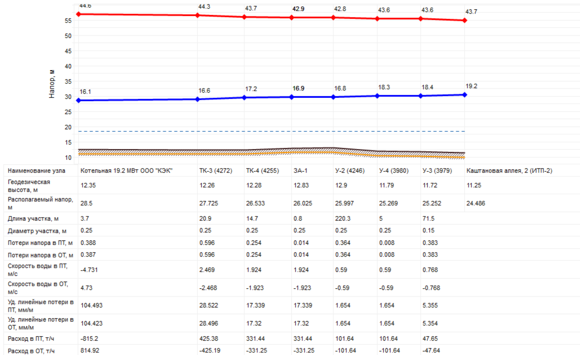
Рисунок 37. Пьезометрический график от котельной 19,2 МВт ООО «КЭК»
