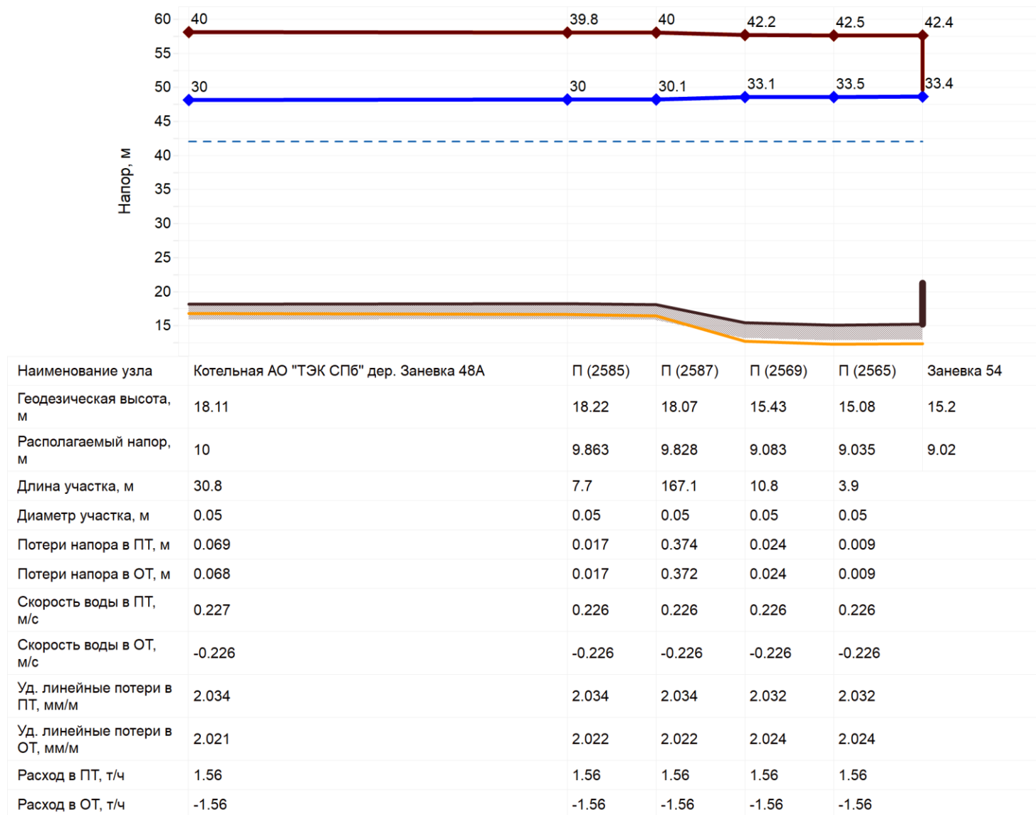
Рисунок 31. Пьезометрический график от котельной АО «ТЭК СПб» Заневка 48А до потребителя Заневка 54.
