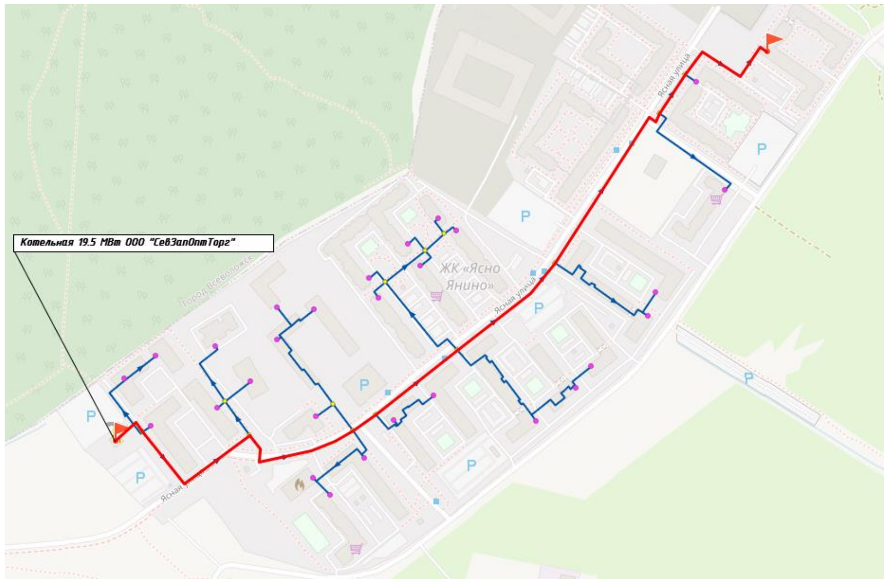
Рисунок 48. Путь построения пьезометрического графика от котельной 19,5 МВт ООО «СЕВЗАПОПТТОРГ»
