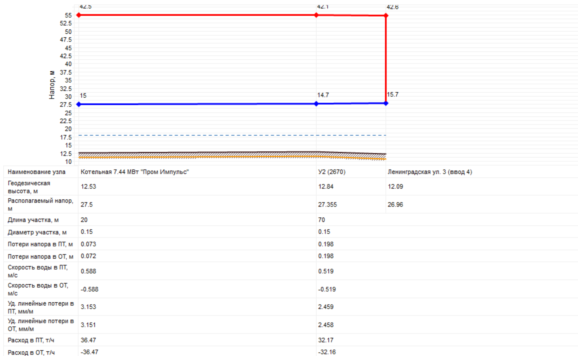
Рисунок 41. Пьезометрический график от котельной 7,44 МВт ООО «Пром Импульс»
