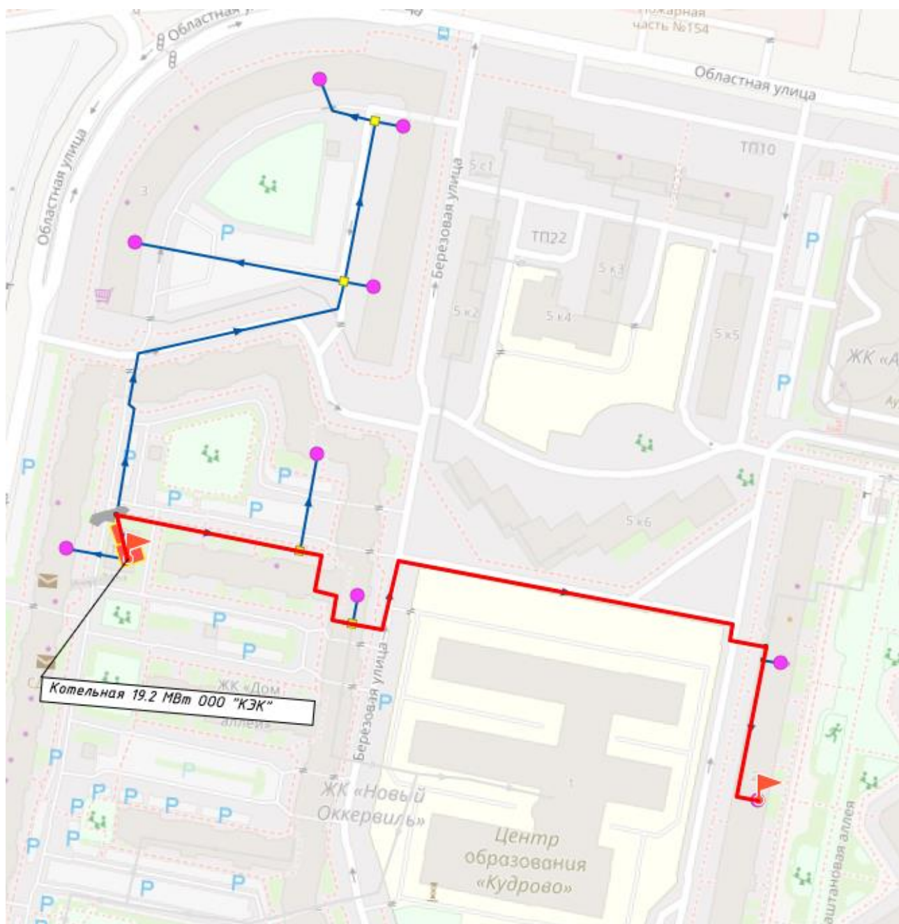
Рисунок 36. Путь построения пьезометрического графика от котельной 19,2 МВт ООО «КЭК»
