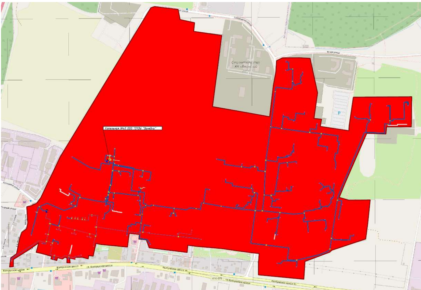
Рисунок 23. Зона действия и тепловые сети котельной № 40 «СМЭУ «Заневка»
