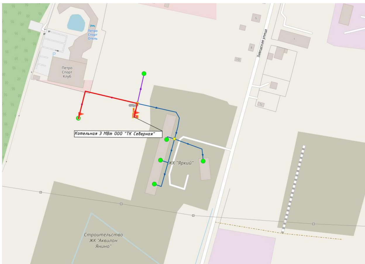
Рисунок 25. Путь построения пьезометрического графика от котельной в 3 МВт ООО «Тепловая Компания Северная»
