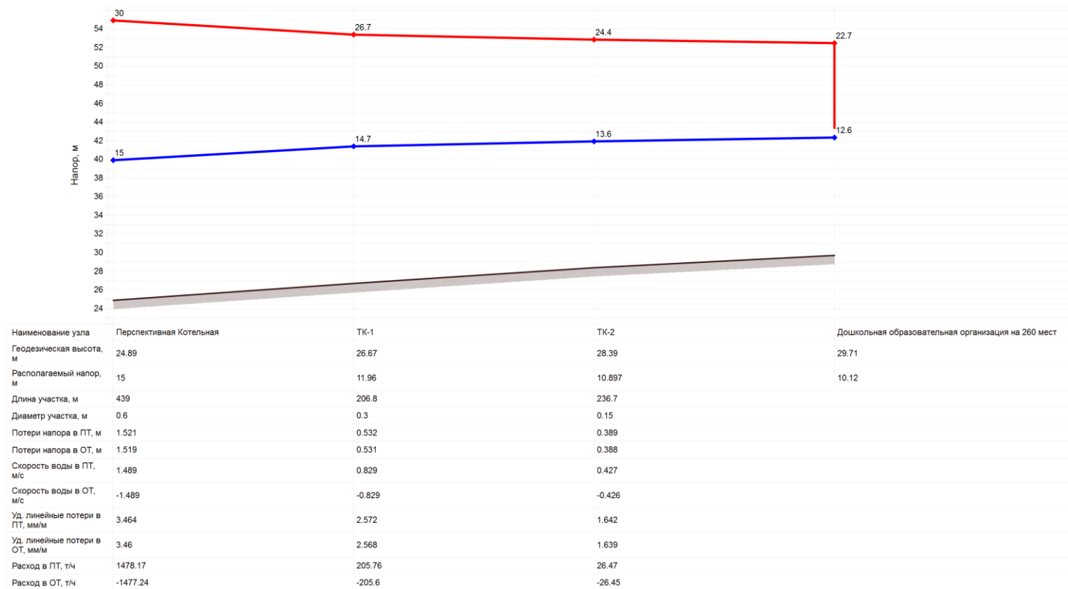
Рисунок 12. Пьезометрический график от новой котельной в дер. Заневка
