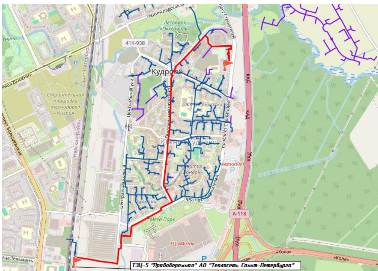
Рисунок 14. Путь построения пьезометрического графика от УТ-4 в системе теплоснабжения АО «Теплосеть Санкт-Петербурга»
