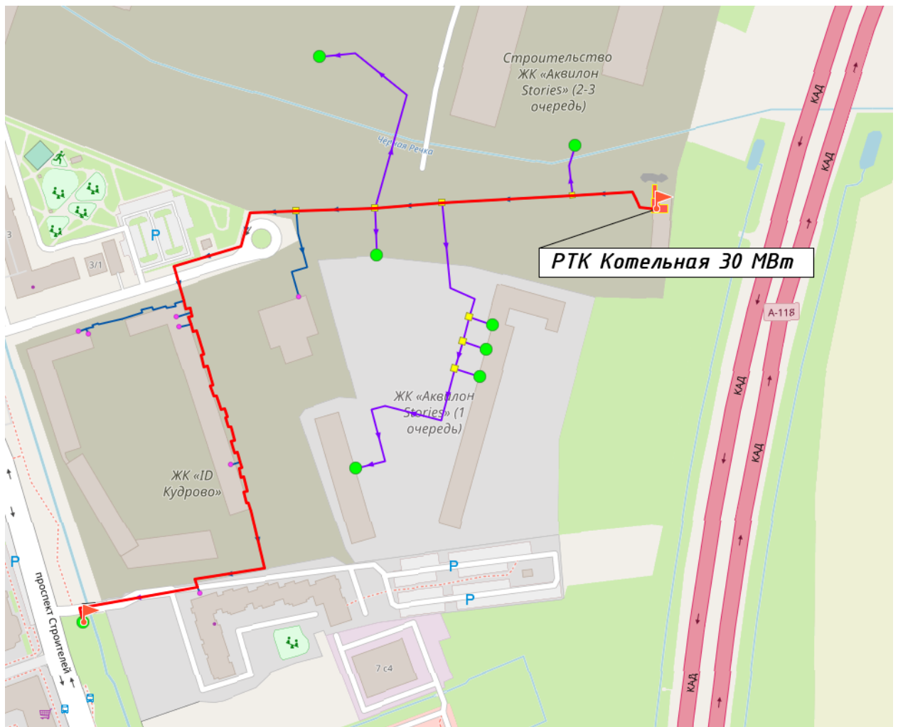
Рисунок 22. Путь построения пьезометрического графика от котельной ООО «РТК»
