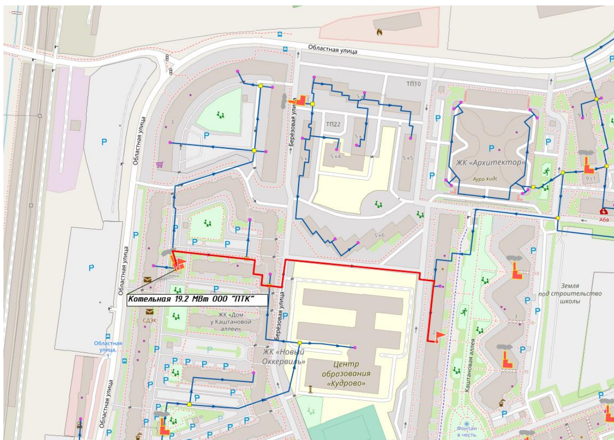
Рисунок 17. Путь построения пьезометрического графика от котельной 19,2 МВт ООО «ПТК»
