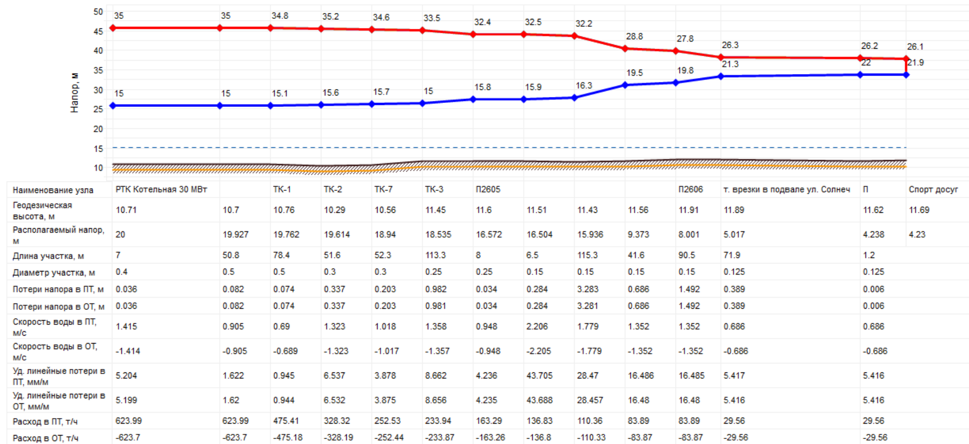
Рисунок 11. Пьезометрический график от котельной ООО «РТК»
