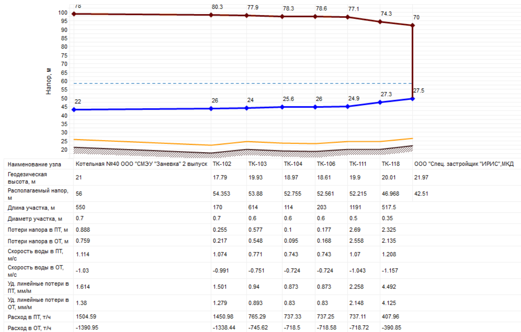
Рисунок 1. Пьезометрический график от котельной № 40 ООО «СМЭУ «Заневка»
