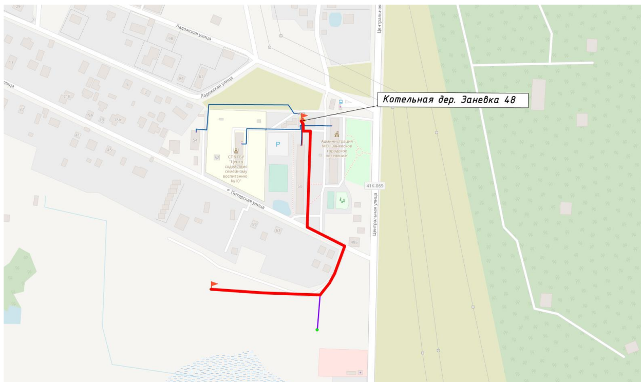
Рисунок 15. Путь построения пьезометрического графика от котельной ГУП «ТЭК СПб» Заневка 48
