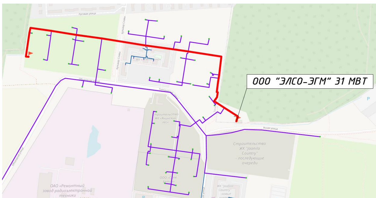
Рисунок 20. Путь построения №2 пьезометрического графика от котельной ООО «ЭЛСО-ЭГМ» 31 МВт
