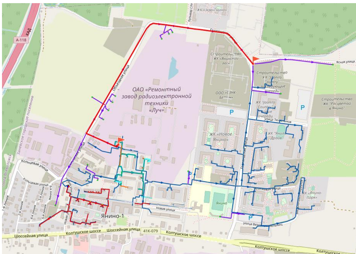
Рисунок 13. Путь построения пьезометрического графика от котельной №40 ООО «СМЭУ «Заневка»
