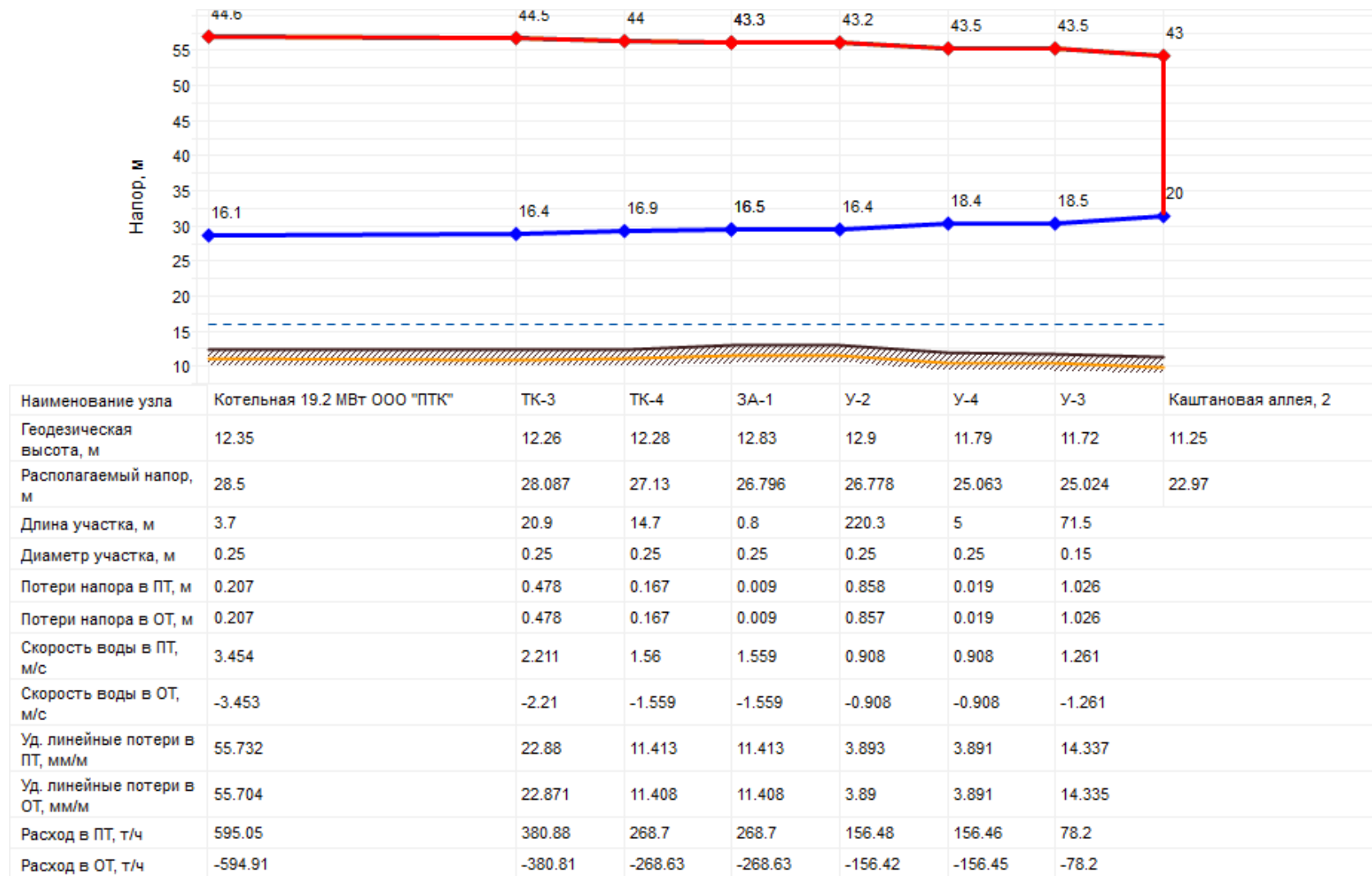
Рисунок 6. Пьезометрический график от котельной 19,2 МВт ООО «ПТК»
