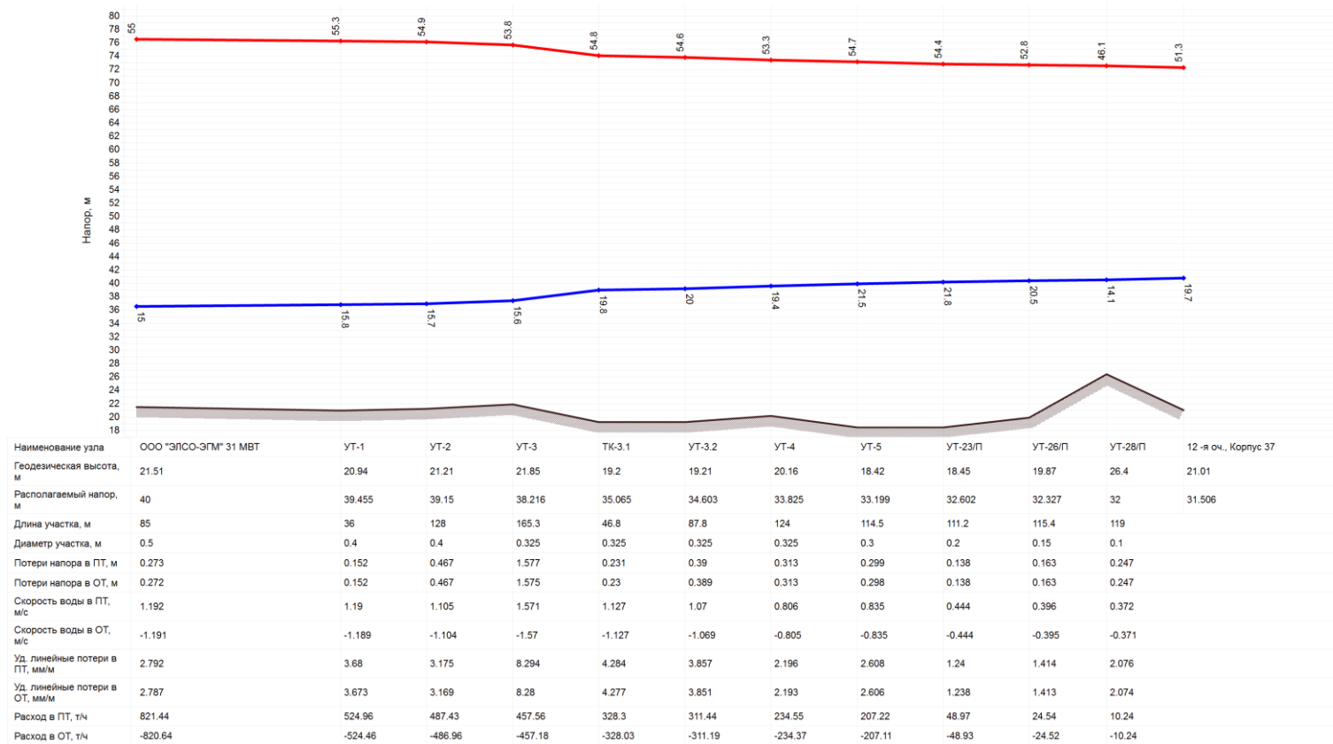
Рисунок 8. Пьезометрический график №1 от котельной ООО «ЭЛСО-ЭГМ» 31 МВт
