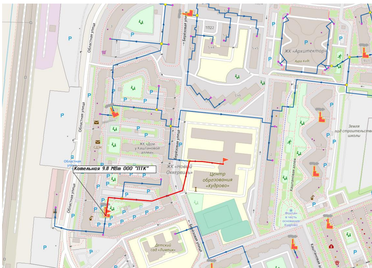
Рисунок 16. Путь построения пьезометрического графика от котельной 9,8 МВт ООО «ПТК»
