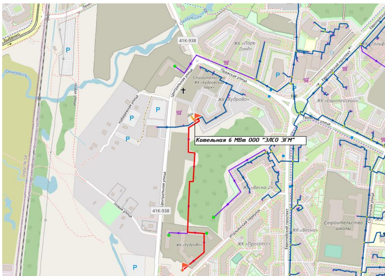
Рисунок 21. Путь построения пьезометрического графика от котельной ООО «ЭЛСО-ЭГМ» 6 МВт
