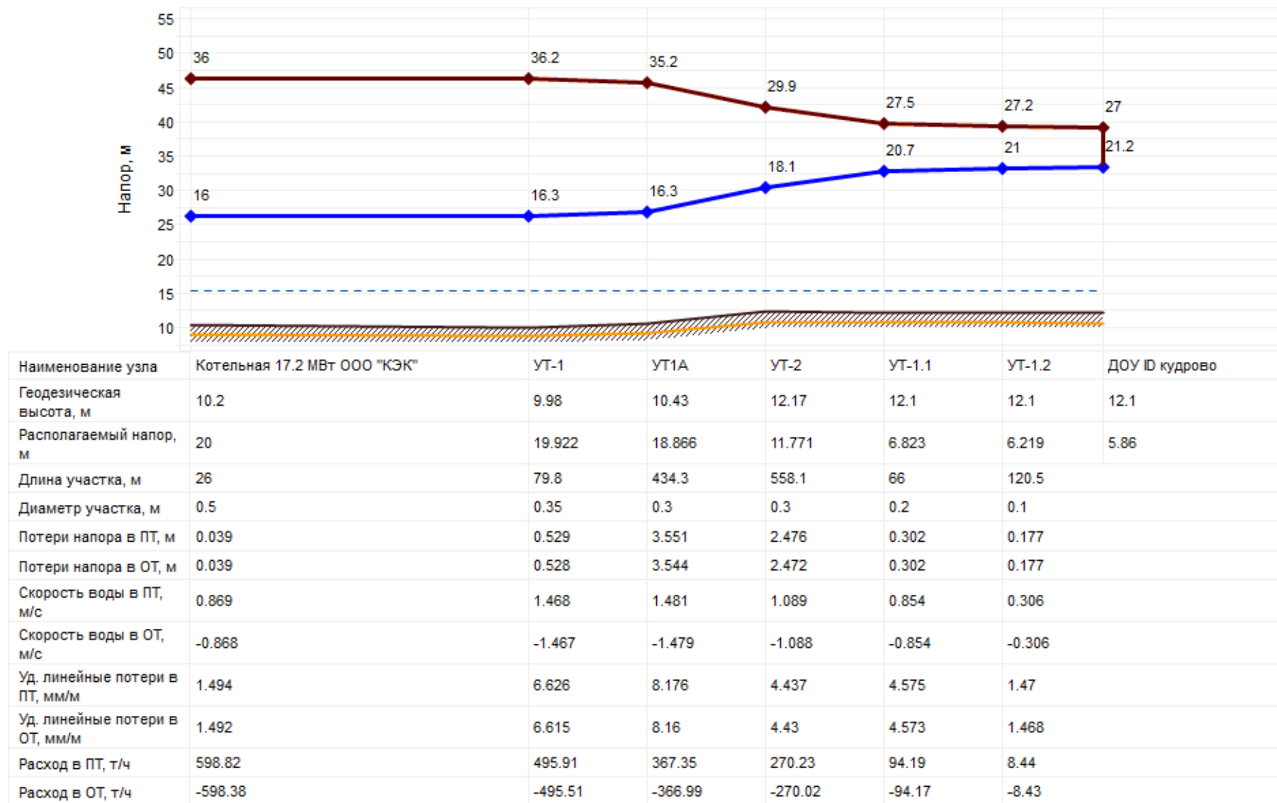
Рисунок 7. Пьезометрический график от котельной 17,2 МВт ООО «КЭК»
