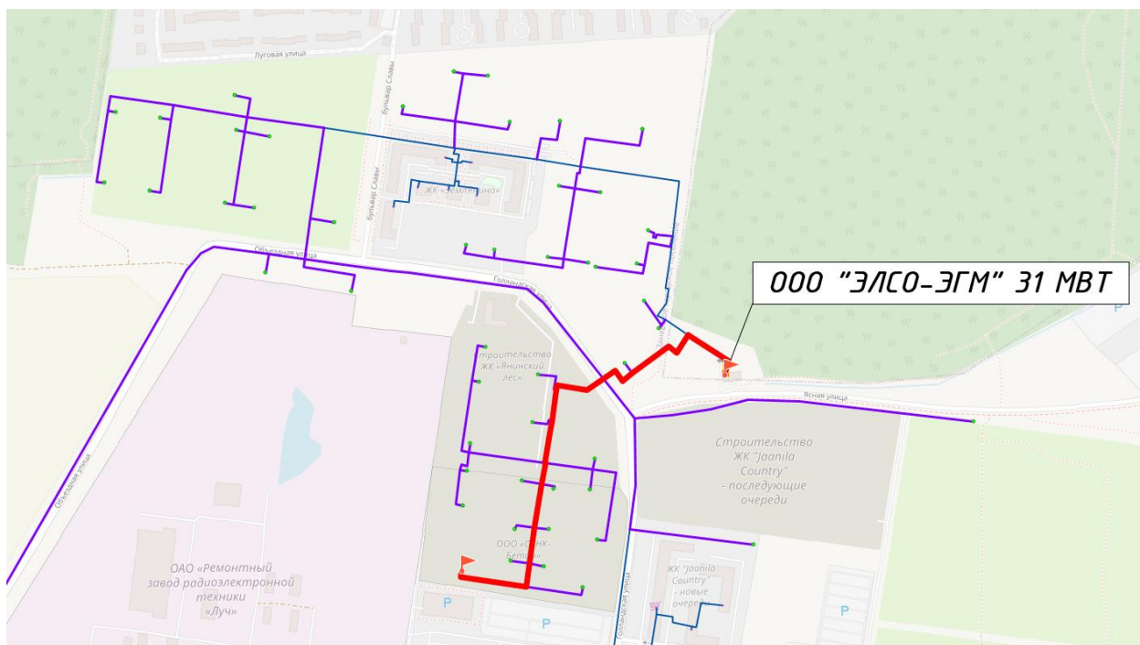
Рисунок 19. Путь построения №1 пьезометрического графика от котельной ООО «ЭЛСО-ЭГМ» 31 МВт
