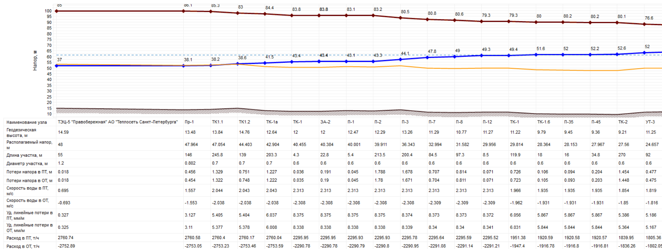
Рисунок 2. Пьезометрический график от УТ-4 ТЭЦ-5 Правобережная (часть 1)
