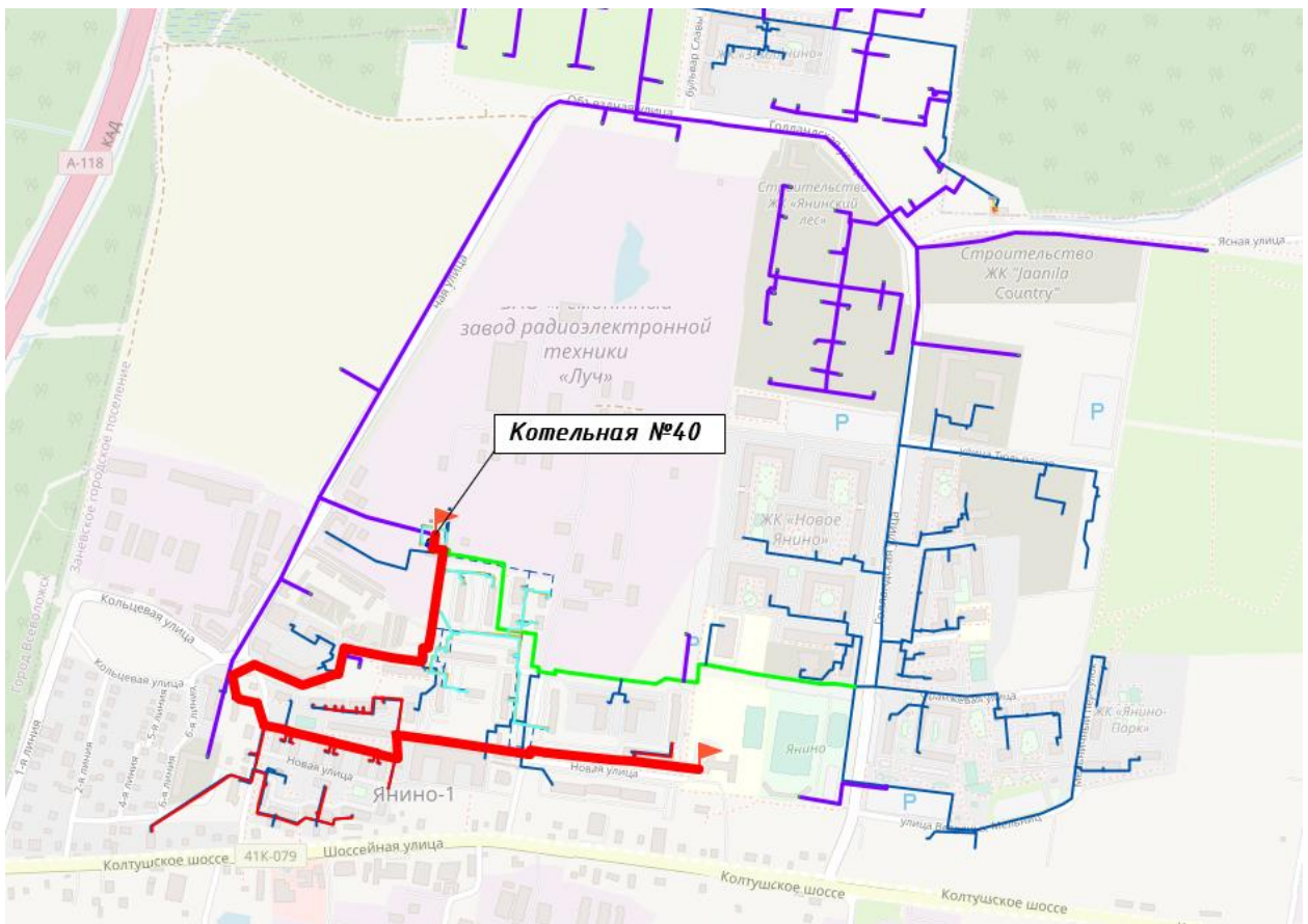
Рисунок 15. Путь построения №1 пьезометрического графика от котельной №40 ООО «СМЭУ «Заневка» до потребителя школа
