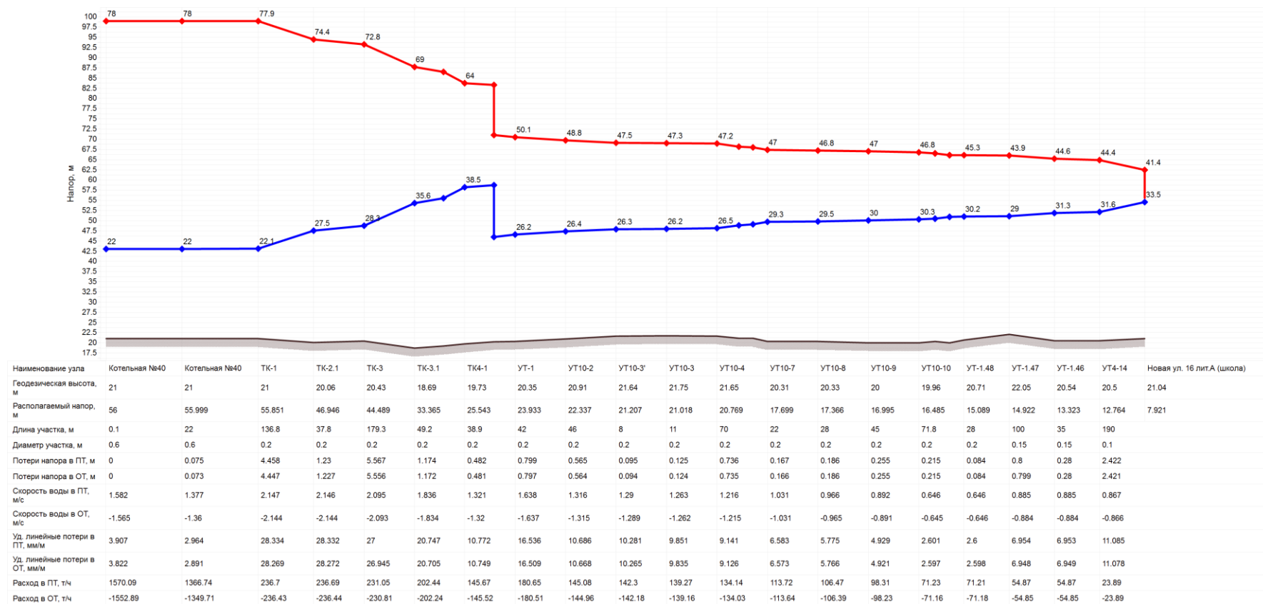
Рисунок 1. Пьезометрический график №1 от котельной № 40 ООО «СМЭУ «Заневка»
