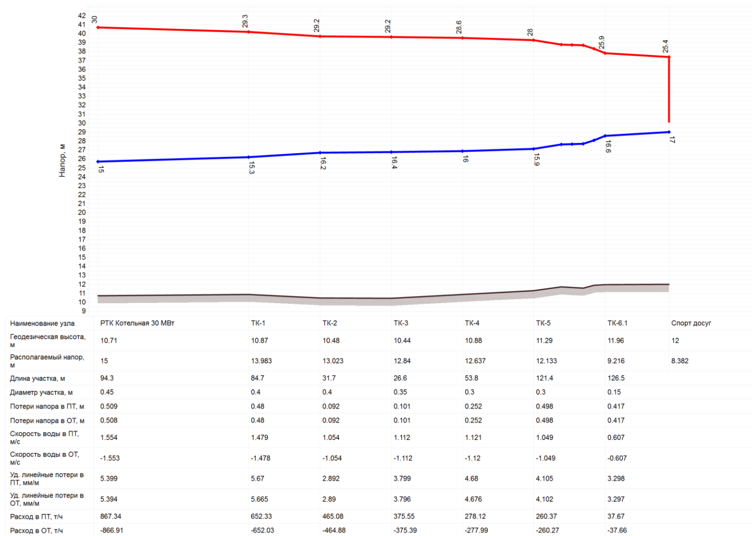
Рисунок 13. Пьезометрический график от новой котельной 30 МВт ООО «РТК»
