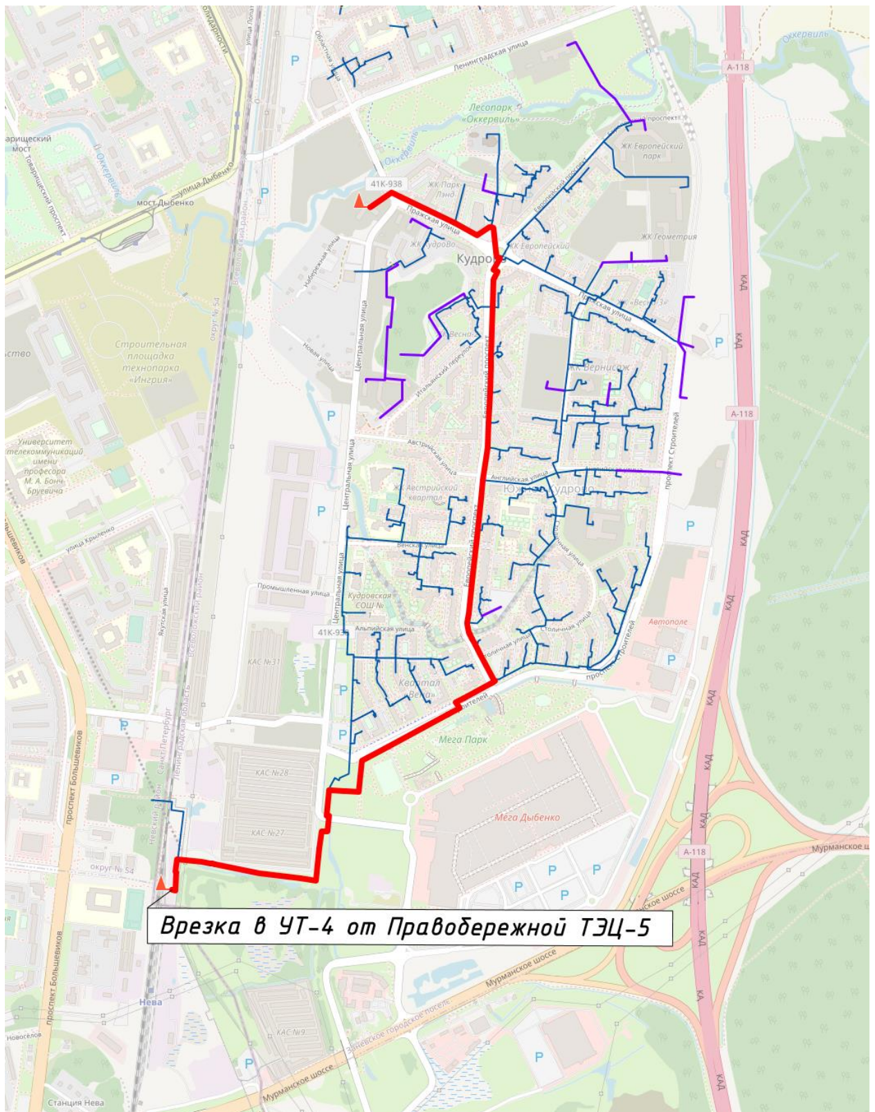
Рисунок 18. Путь построения №2 пьезометрического графика от УТ-4 в системе теплоснабжения АО «Теплосеть Санкт-Петербурга»
