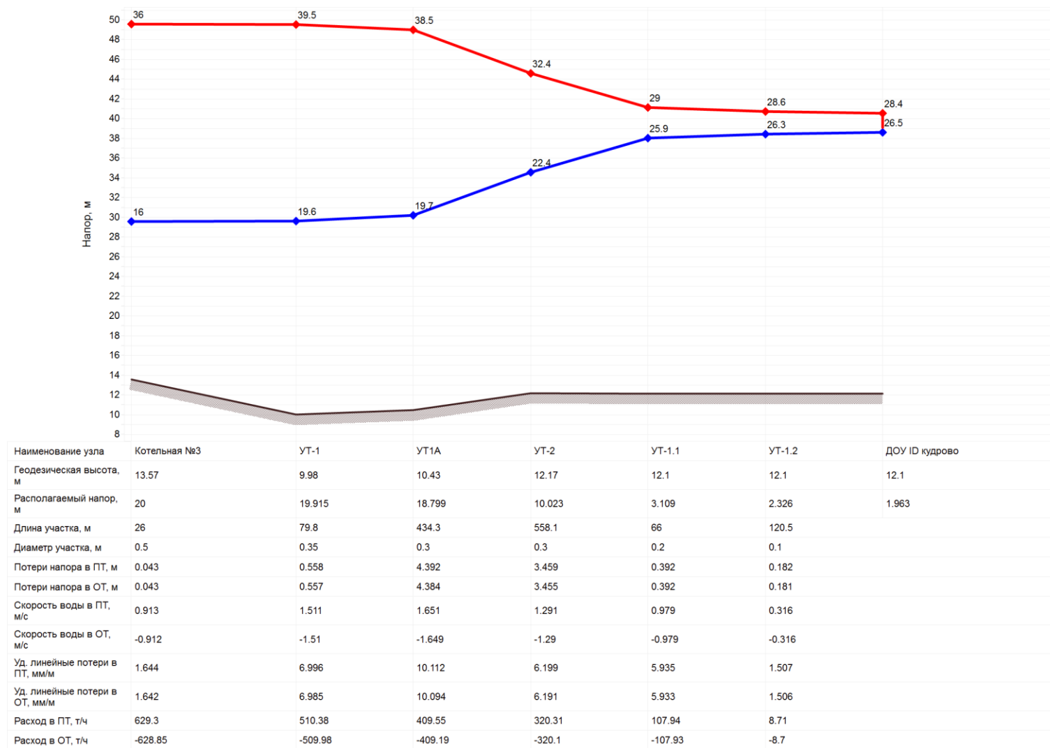
Рисунок 7. Пьезометрический график от котельной №3 ООО «Энергия»
