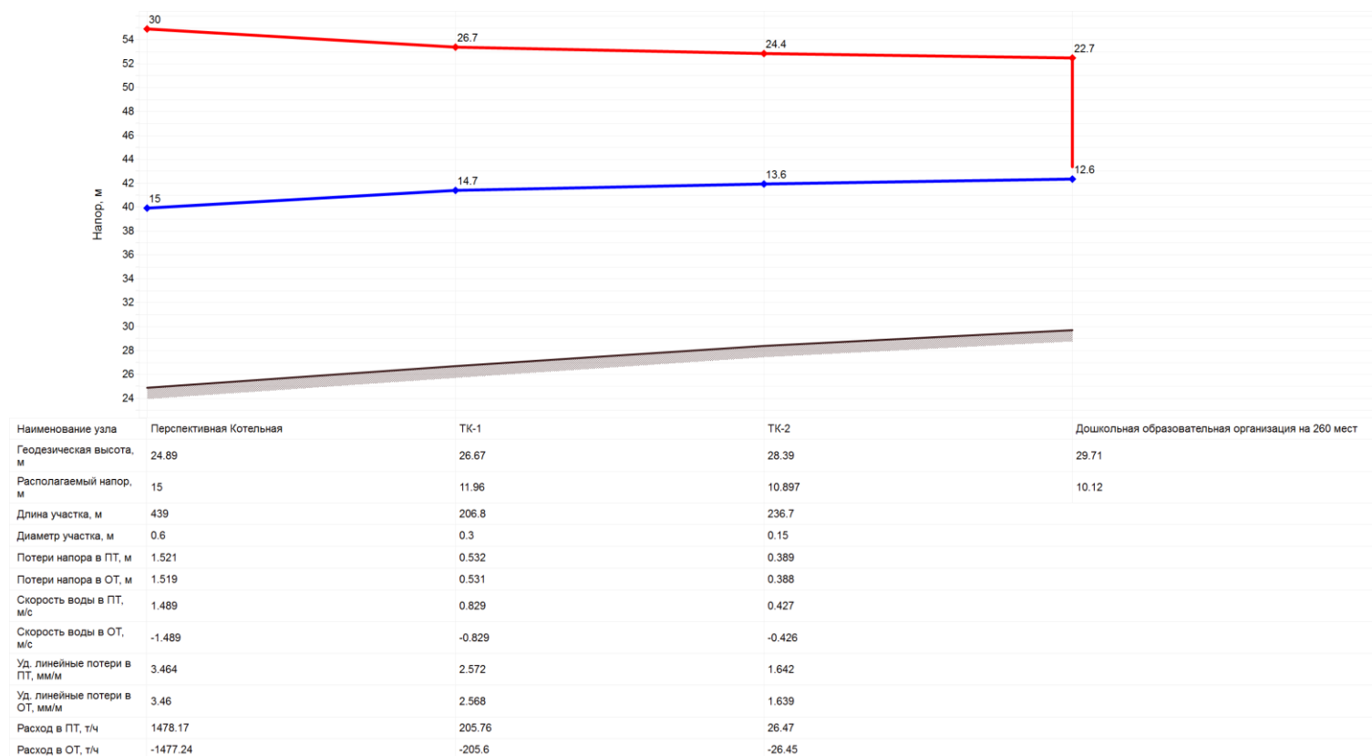
Рисунок 14. Пьезометрический график от новой котельной в дер. Заневка
