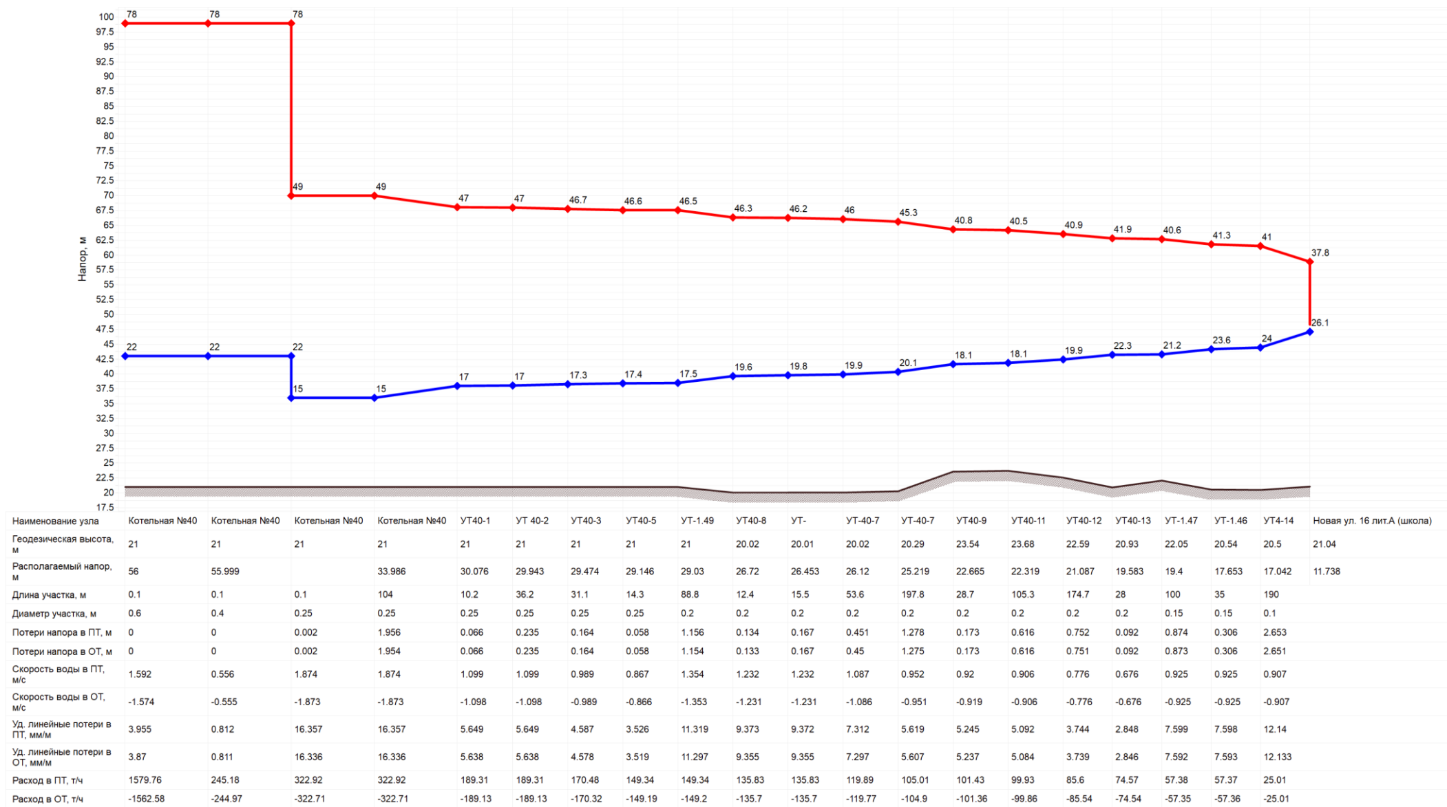
Рисунок 1. Пьезометрический график №1 от котельной № 40 ООО «СМЭУ «Заневка»
