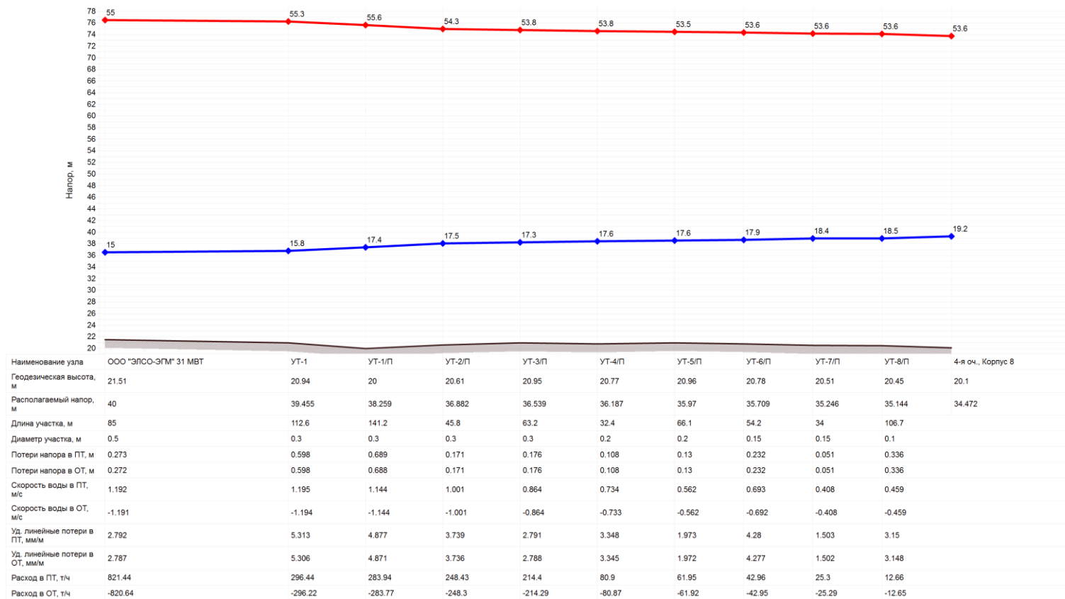
Рисунок 11. Пьезометрический график №2 от котельной ООО «ЭЛСО-ЭГМ» 31 МВт
