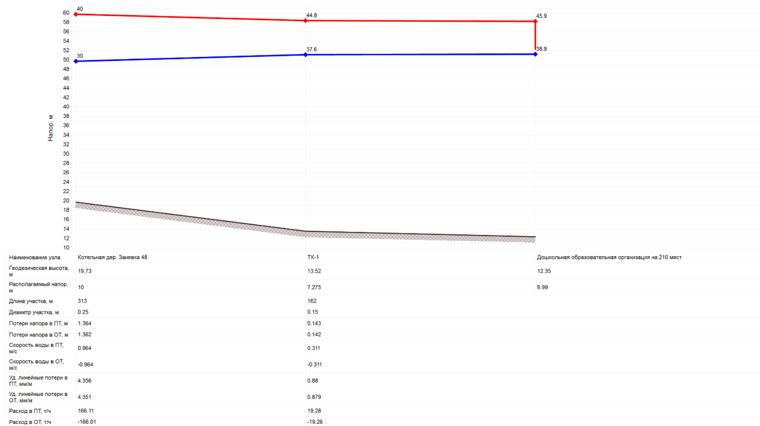
Рисунок 6. Пьезометрический график от котельной ГУП «ТЭК СПб» Заневка 48
