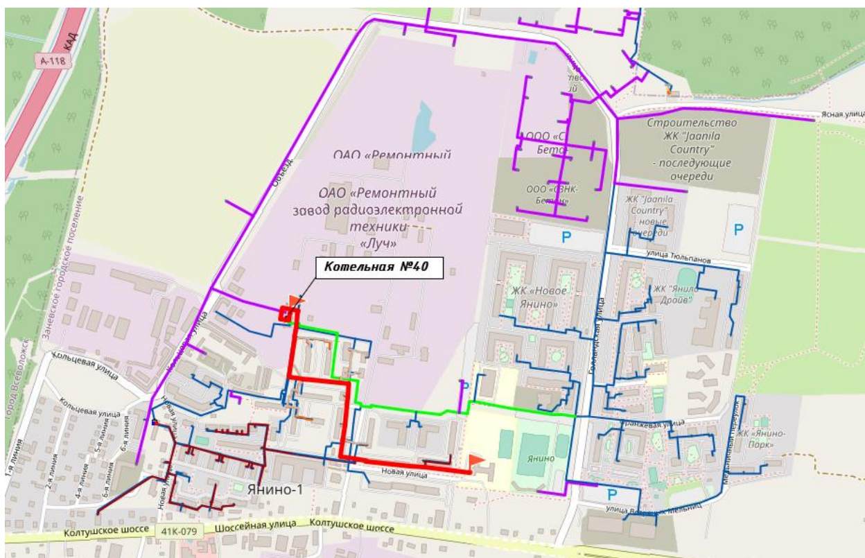
Рисунок 15. Путь построения №1 пьезометрического графика от котельной №40 ООО «СМЭУ «Заневка» до потребителя школа
