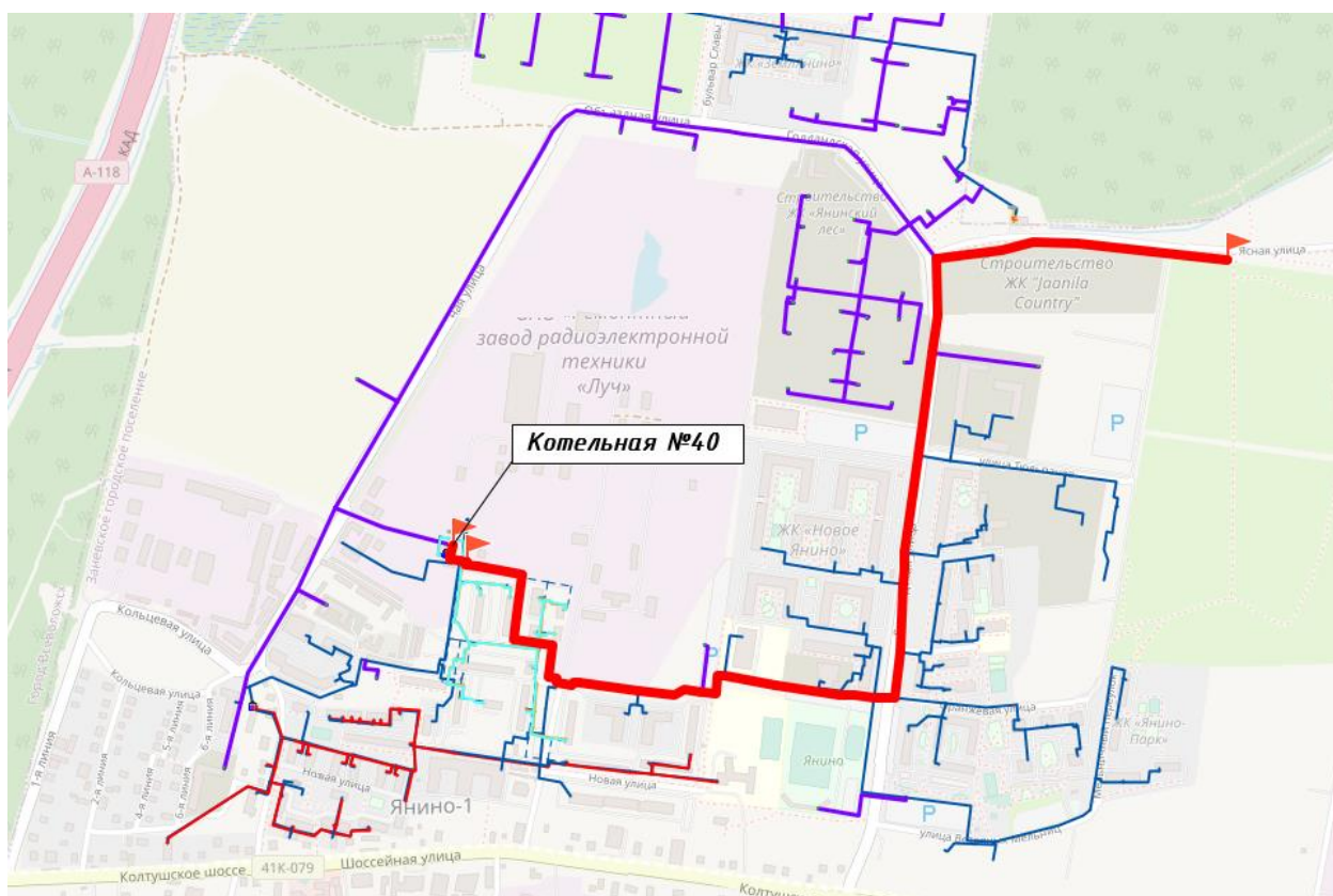
Рисунок 16. Путь построения №2 пьезометрического графика от котельной №40 ООО «СМЭУ «Заневка» до потребителя «ИРИС» , МКД
