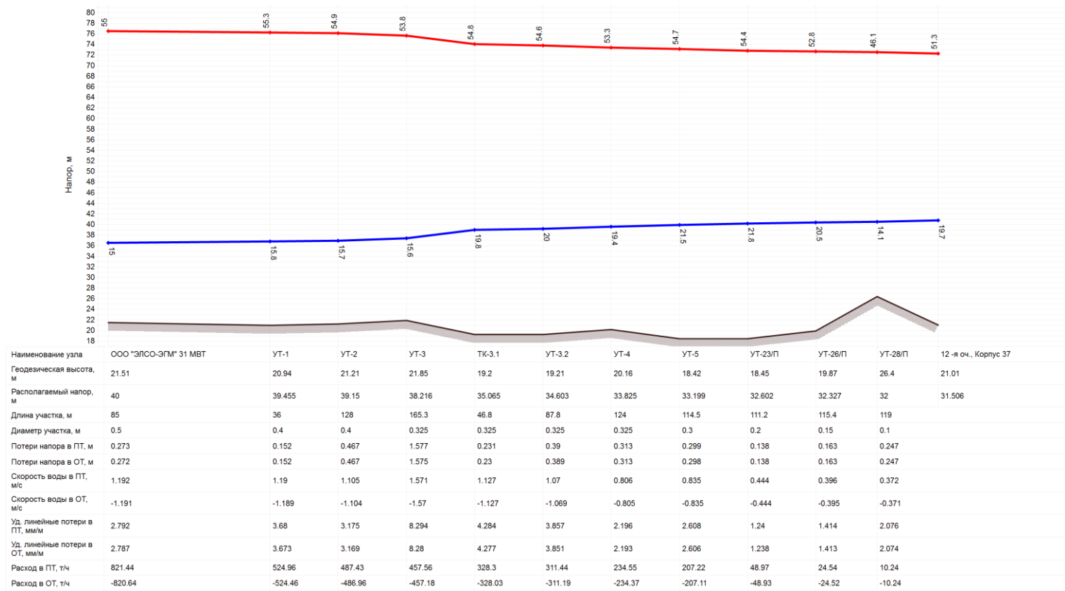
Рисунок 10. Пьезометрический график №1 от котельной ООО «ЭЛСО-ЭГМ» 31 МВт
