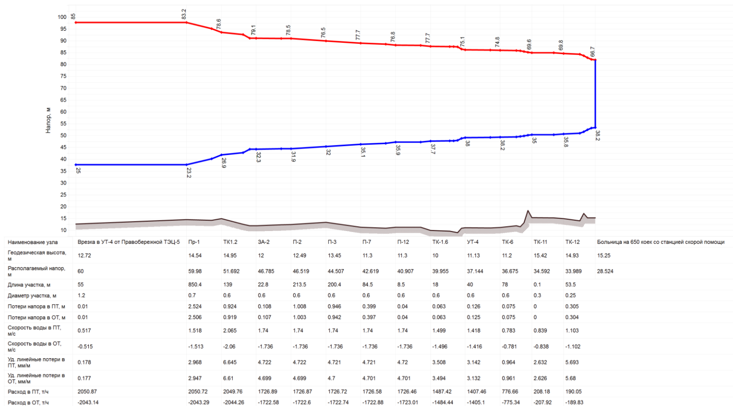
Рисунок 3. Пьезометрический график №1 от УТ-4 ТЭЦ-5 Правобережная
