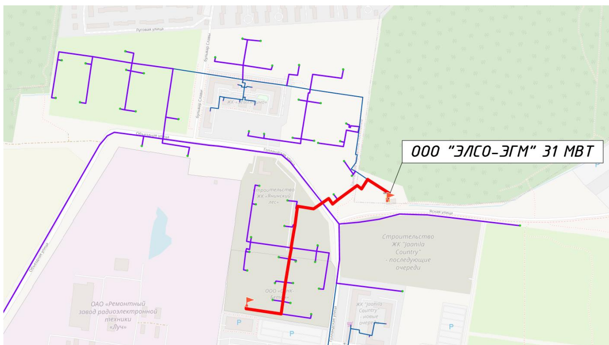
Рисунок 24. Путь построения №1 пьезометрического графика от котельной ООО «ЭЛСО-ЭГМ» 31 МВт
