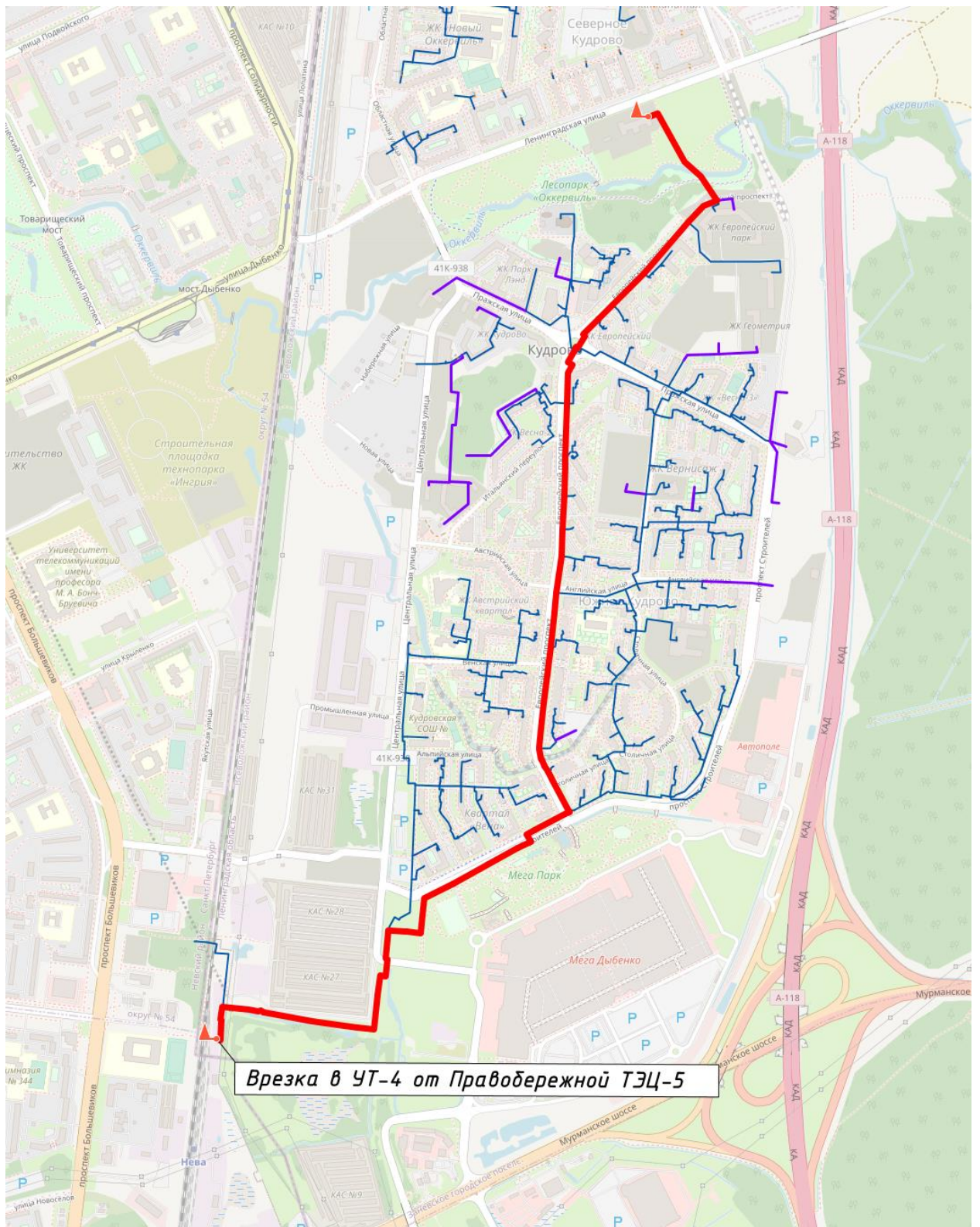
Рисунок 17. Путь построения №1 пьезометрического графика от УТ-4 в системе теплоснабжения АО «Теплосеть Санкт-Петербурга»
