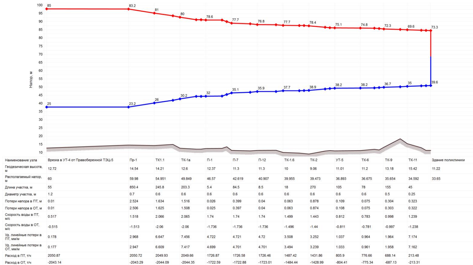
Рисунок 4. Пьезометрический график № 2от УТ-4 ТЭЦ-5 Правобережная
