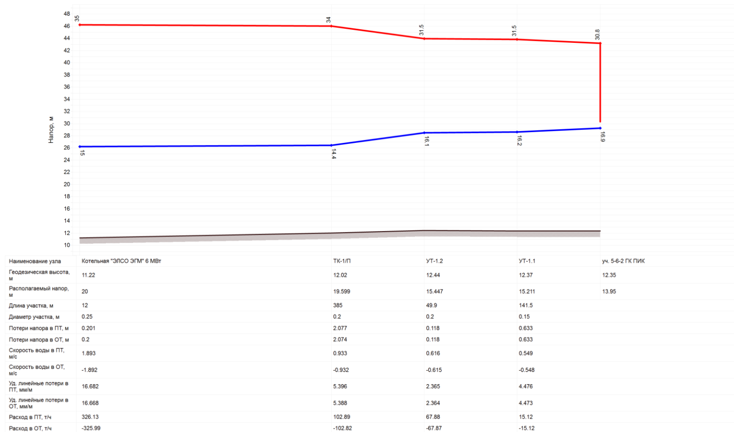
Рисунок 12. Пьезометрический график от котельной ООО «ЭЛСО-ЭГМ» 6 МВт
