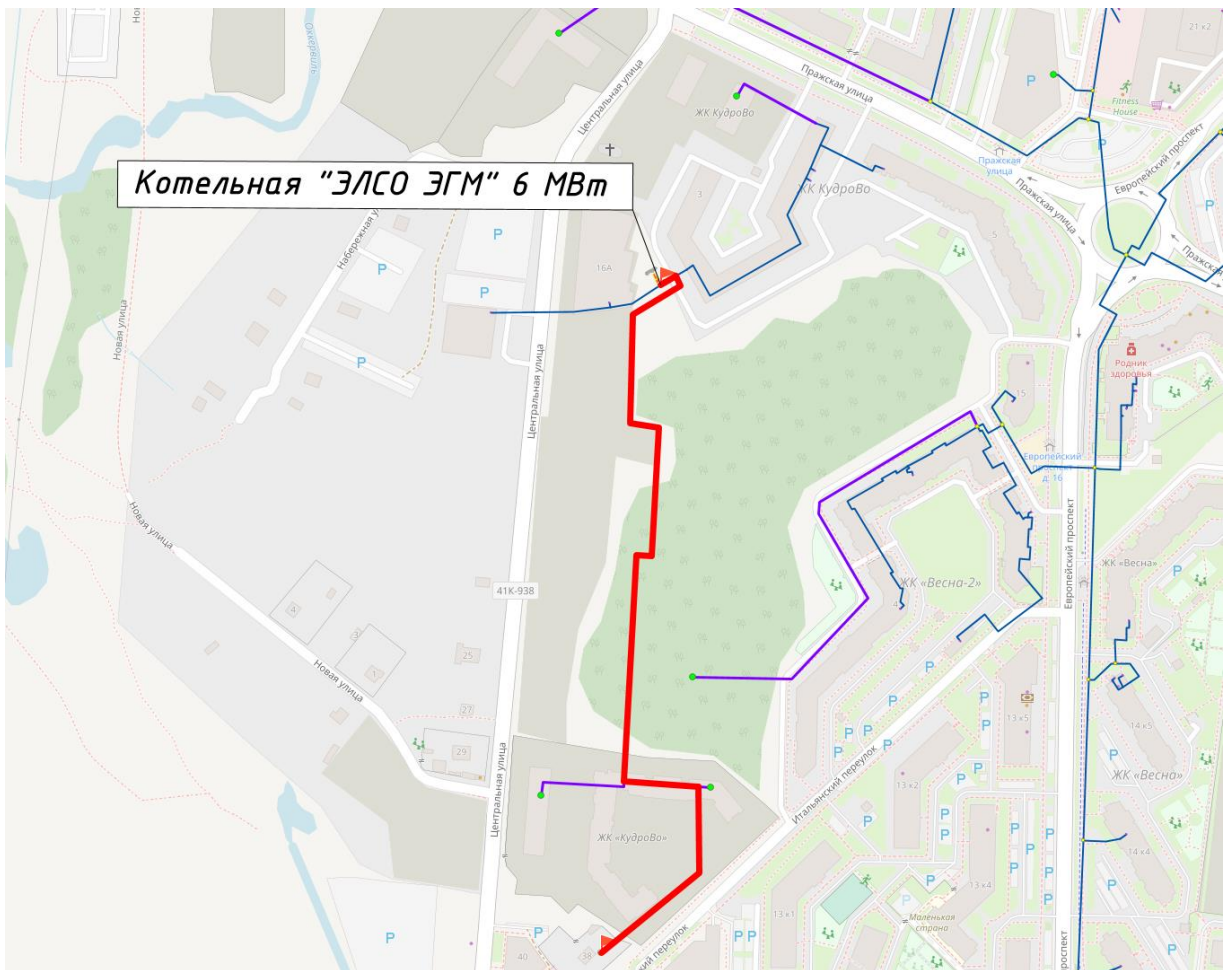
Рисунок 26. Путь построения пьезометрического графика от котельной ООО «ЭЛСО-ЭГМ» 6 МВт
