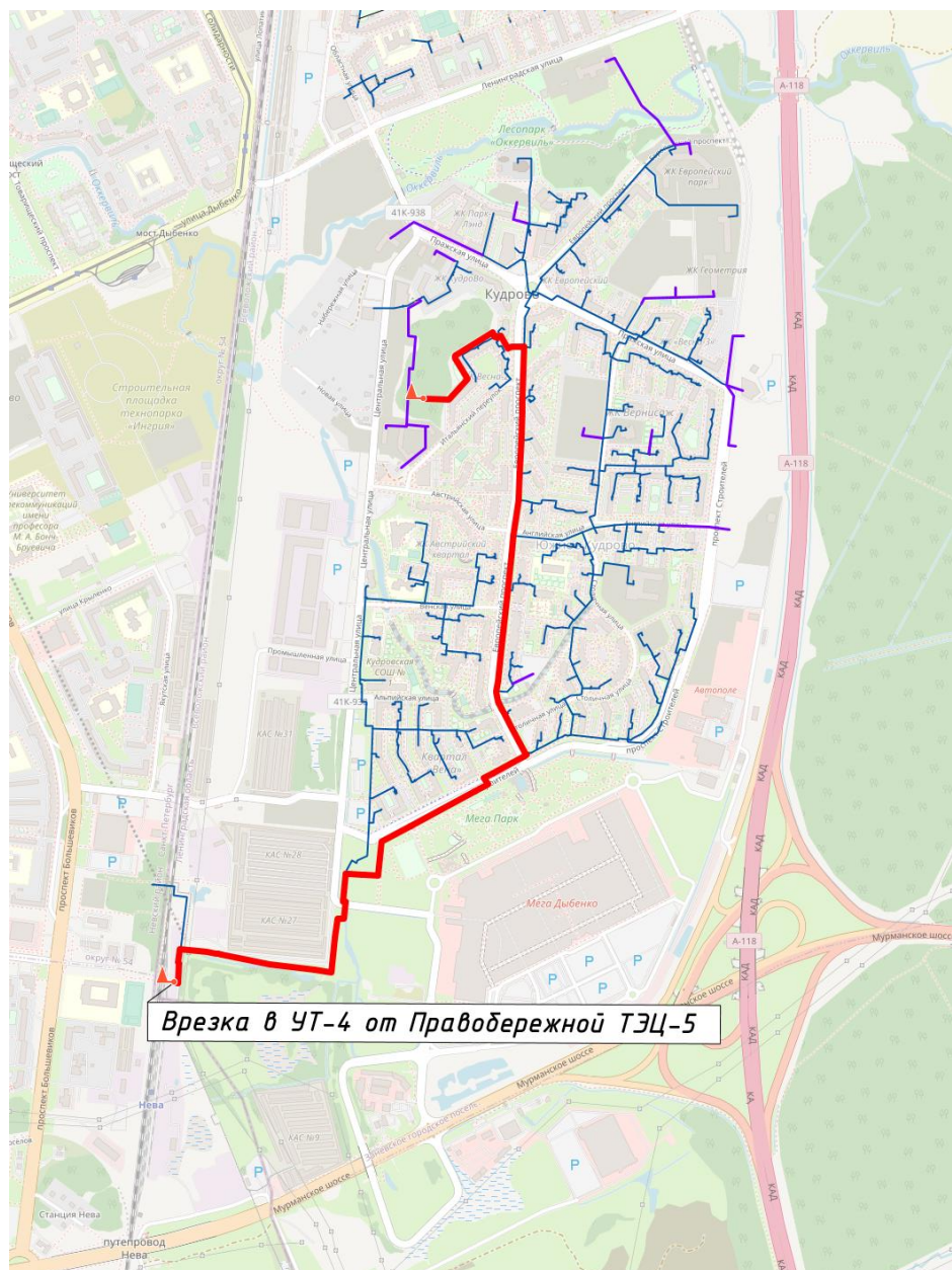
Рисунок 19. Путь построения №3 пьезометрического графика от УТ-4 в системе теплоснабжения АО «Теплосеть Санкт-Петербурга»
