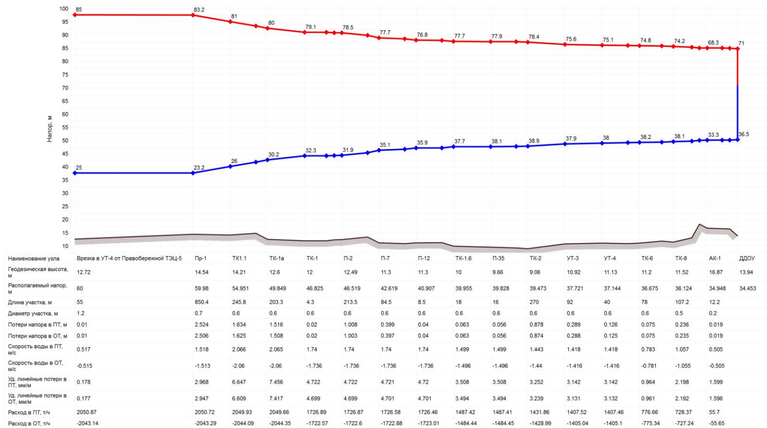
Рисунок 5. Пьезометрический график № 3 от УТ-4 ТЭЦ-5 Правобережная
