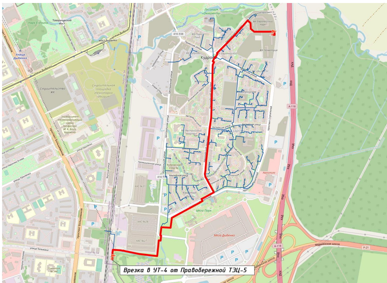
Рисунок 28. Путь построения пьезометрического графика от Правобережной ТЭЦ-5 до потребителя на уч. 2, кад. № 47:07:1044001:593.
