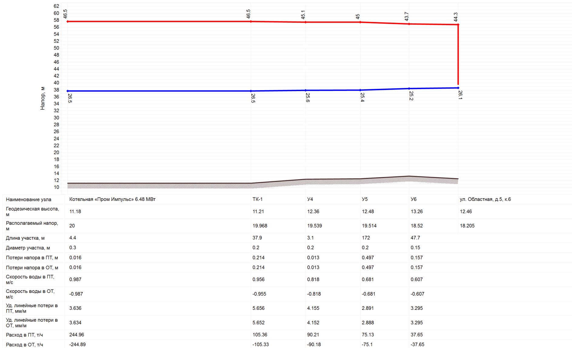
Рисунок 39. Пьезометрический график от котельной 6,48 МВт ООО «Пром Импульс» до потребителя на ул. Областной д.5
