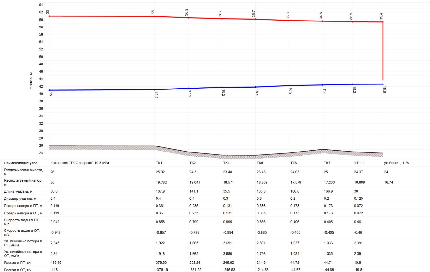
Рисунок 47. Пьезометрический график от котельной 19,5 МВт ООО «Тепловая Компания Северная» до потребителя по ул. Ясная, 11 кб
