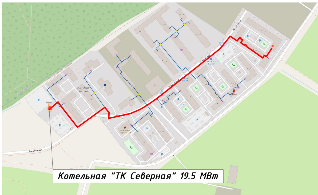
Рисунок 46. Путь построения пьезометрического графика от котельной 19,5 МВт ООО «Тепловая Компания Северная» до потребителя по ул. Ясная, 11к6
