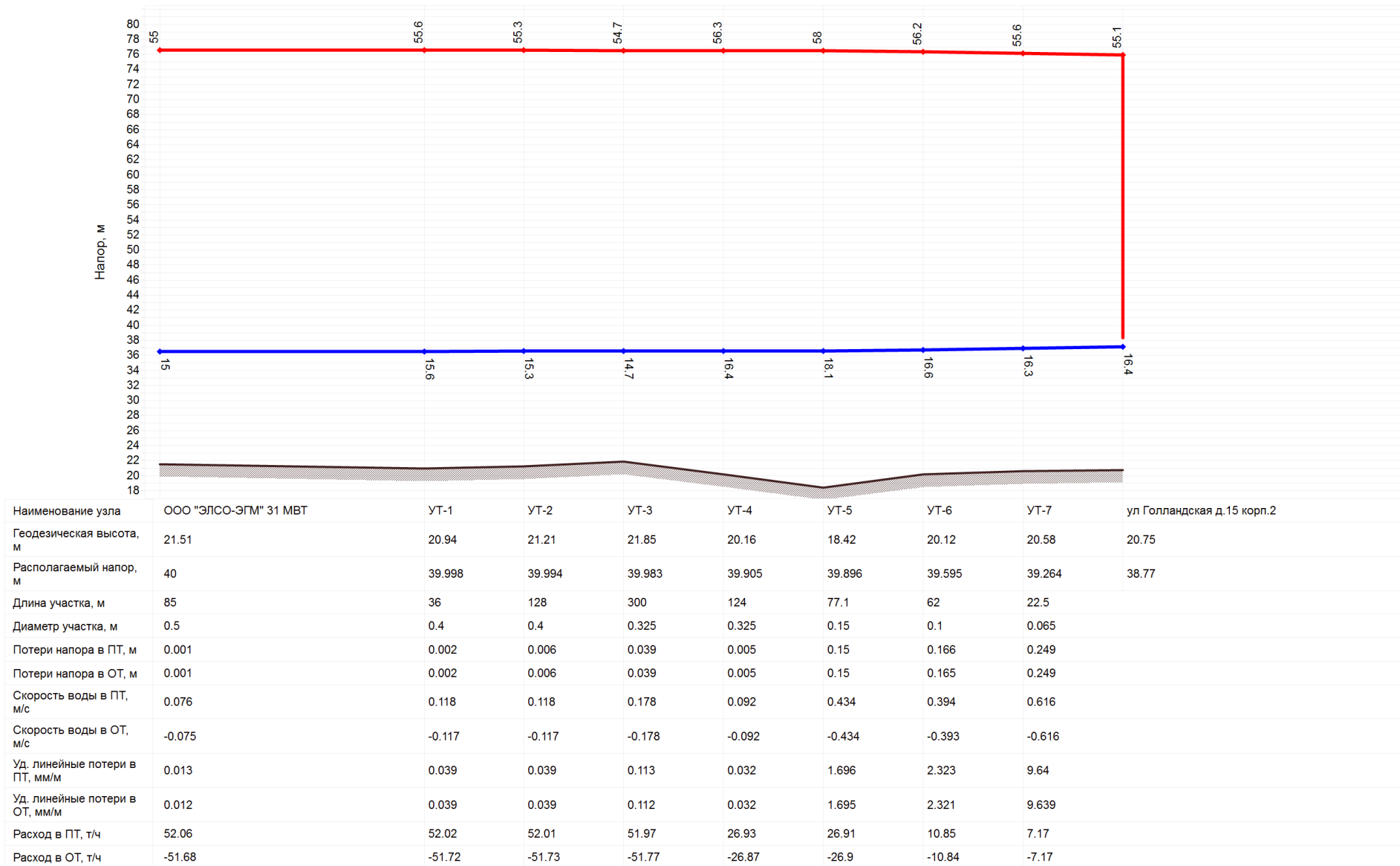
Рисунок 45. Пьезометрический график от котельной 31 МВт ООО «ЭЛСО-ЭГМ» до потребителя ЖД Голландская 15к2
