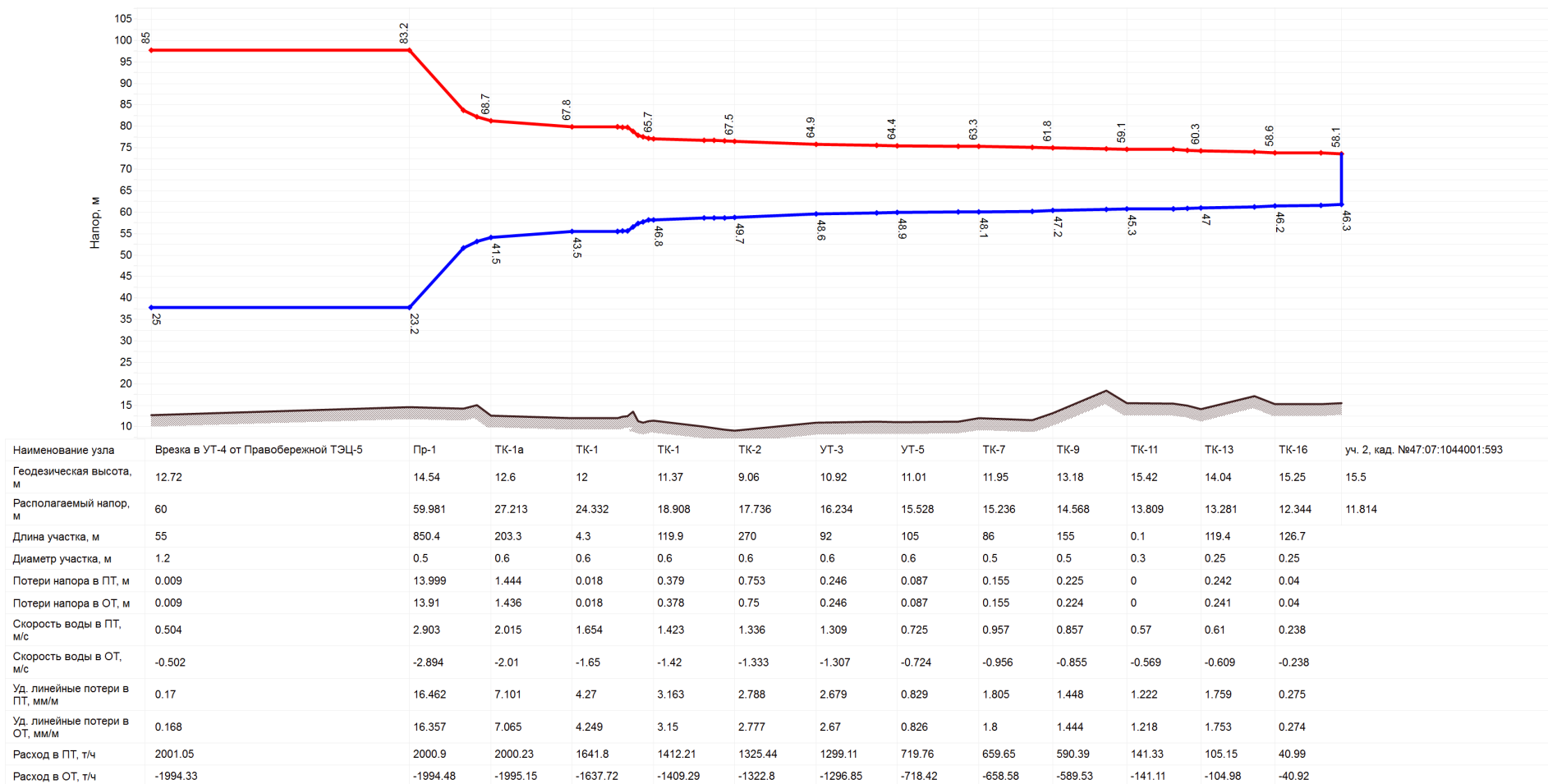
Рисунок 29. Пьезометрический график от Правобережной ТЭЦ-5 до потребителя на уч. 2, кад. № 47:07:1044001:593
