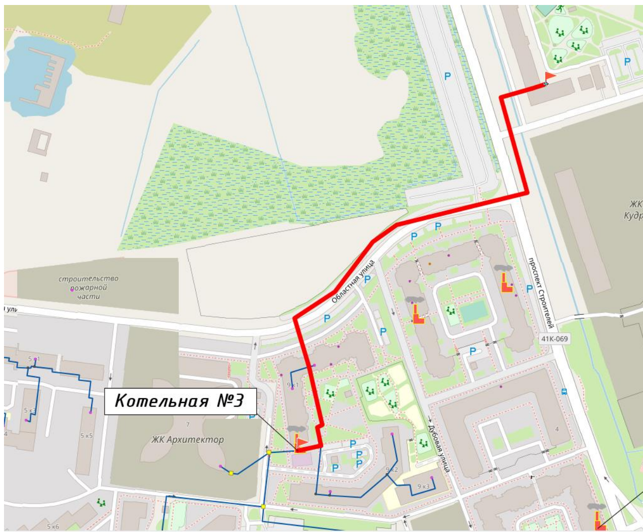
Рисунок 36. Путь построения пьезометрического графика от котельной ООО «Энергия» №3 до потребителя по ул. Строителей, 3.
