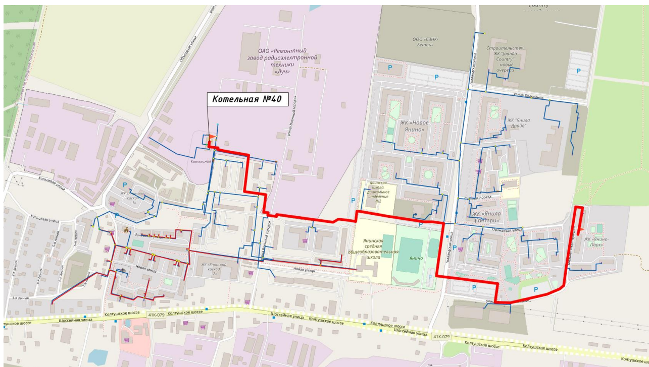
Рисунок 26. Путь построения пьезометрического графика от котельной 40 ООО «СМЭУ «Заневка» до потребителя по пер. Мельничный
