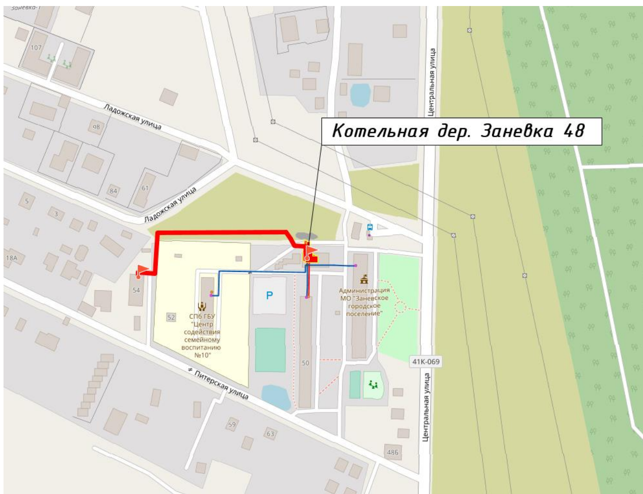
Рисунок 30. Путь построения пьезометрического графика от котельной ГУП «ТЭК СПб» Заневка 48 до потребителя Заневка 54.
