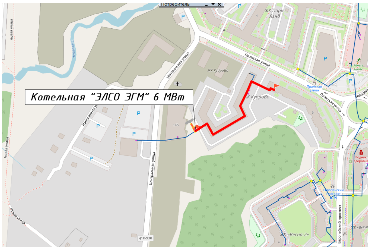
Рисунок 42. Путь построения пьезометрического графика от котельной 6 МВт ООО «ЭЛСО-ЭГМ» до потребителя по ул. Празжская 5
