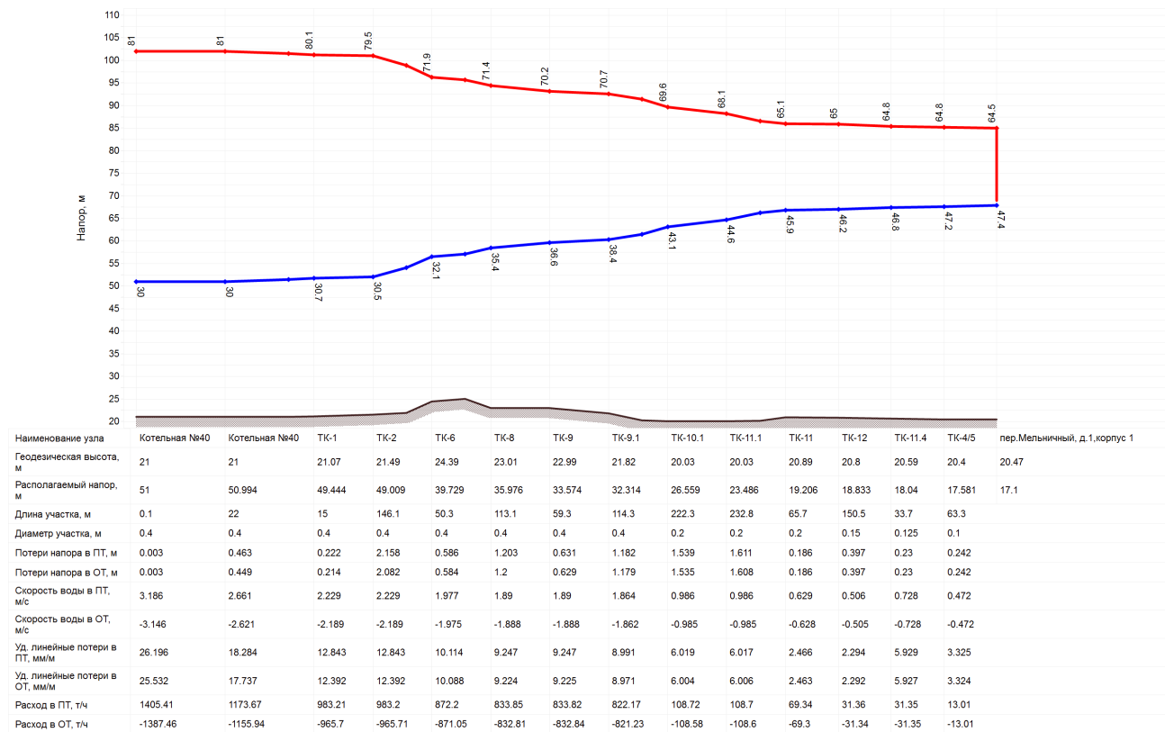
Рисунок 27. Пьезометрический график от котельной № 40 ООО «СМЭУ «Заневка» до потребителя на пер. Мельничный
