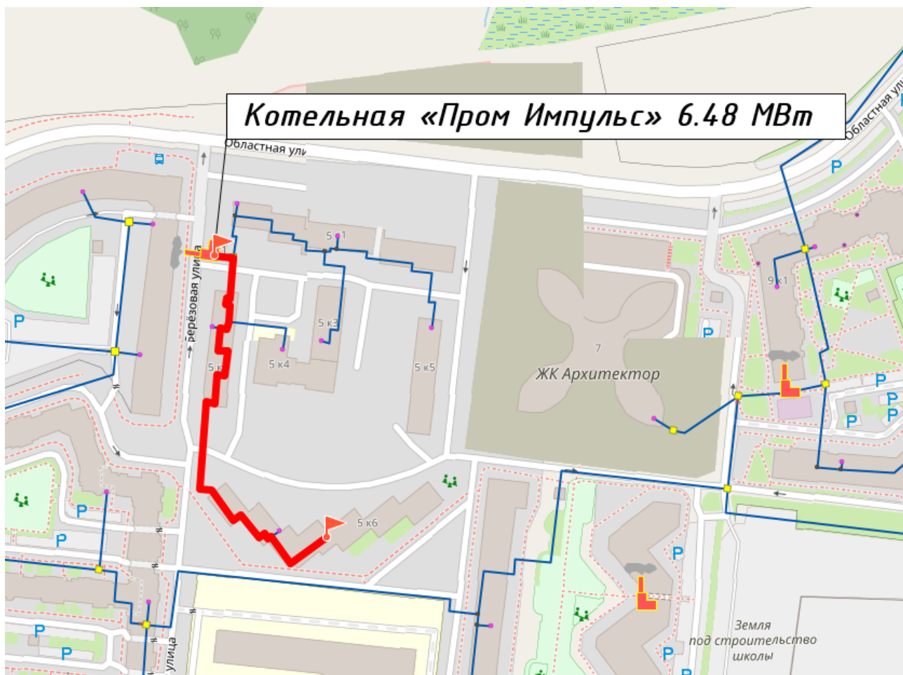
Рисунок 38. Путь построения пьезометрического графика от котельной 6,48 МВт до потребителя по ул. Областной 5
