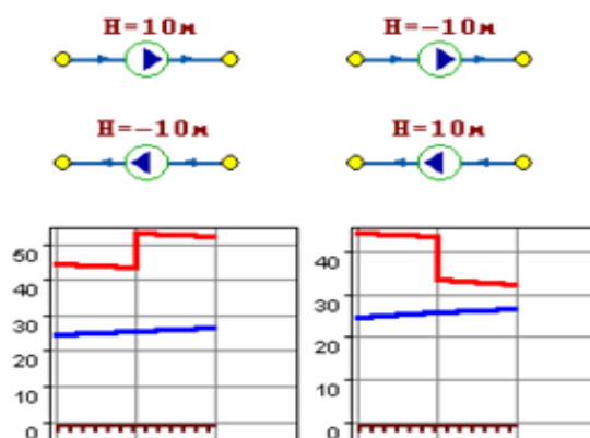
Рисунок 16. Пьезометрические графики
