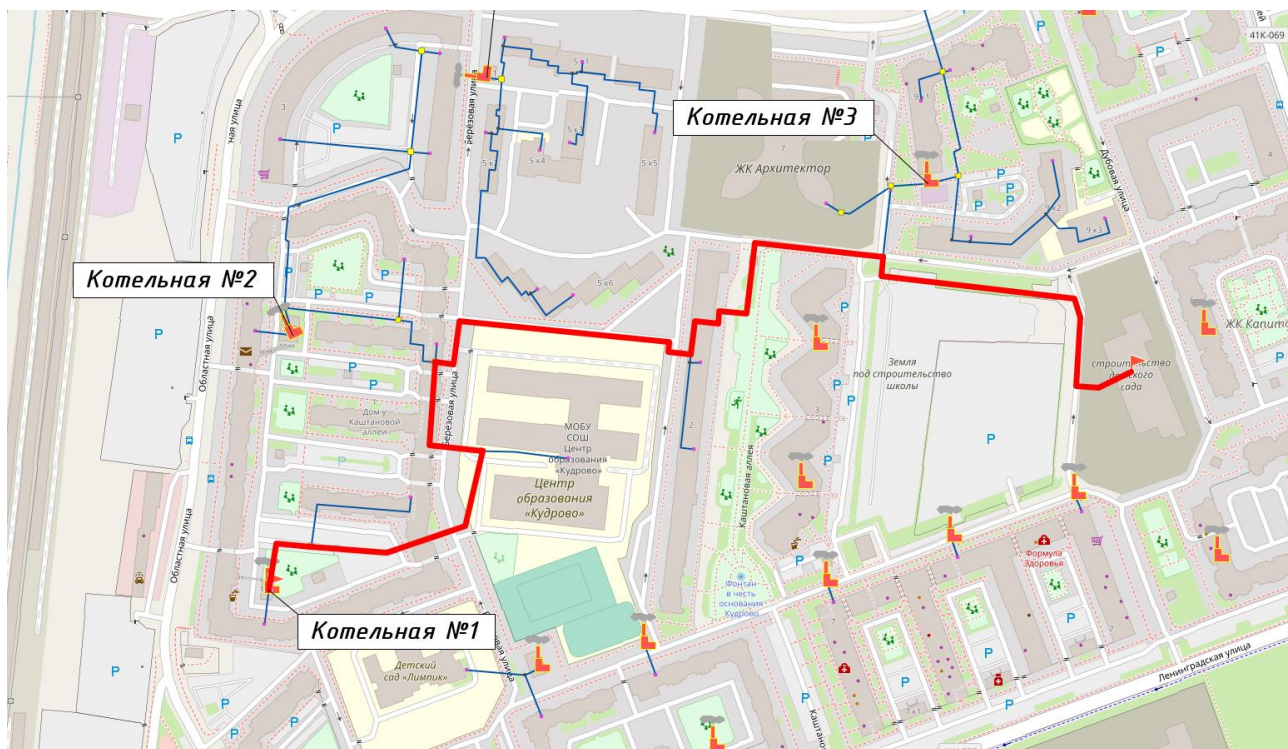
Рисунок 32. Путь построения пьезометрического графика от котельной ООО «Энергия» №1 до потребителя Кудровский ДСКВ №3.
