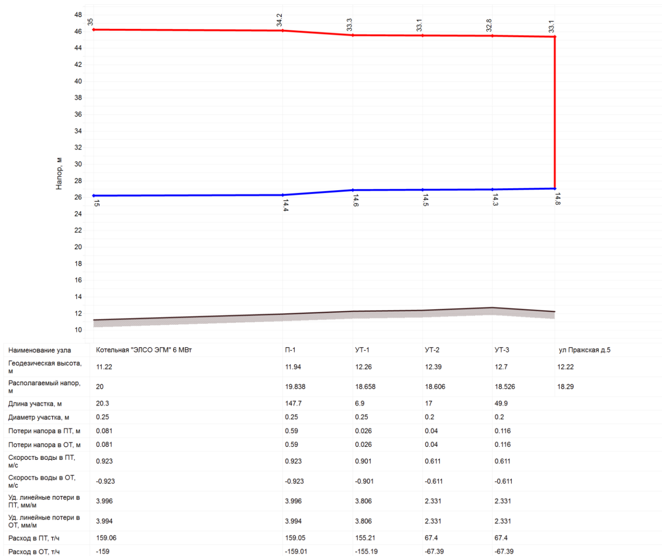
Рисунок 43. Пьезометрический график от котельной 6 МВт ООО «ЭЛСО-ЭГМ» до потребителя по ул. Пражская 5
