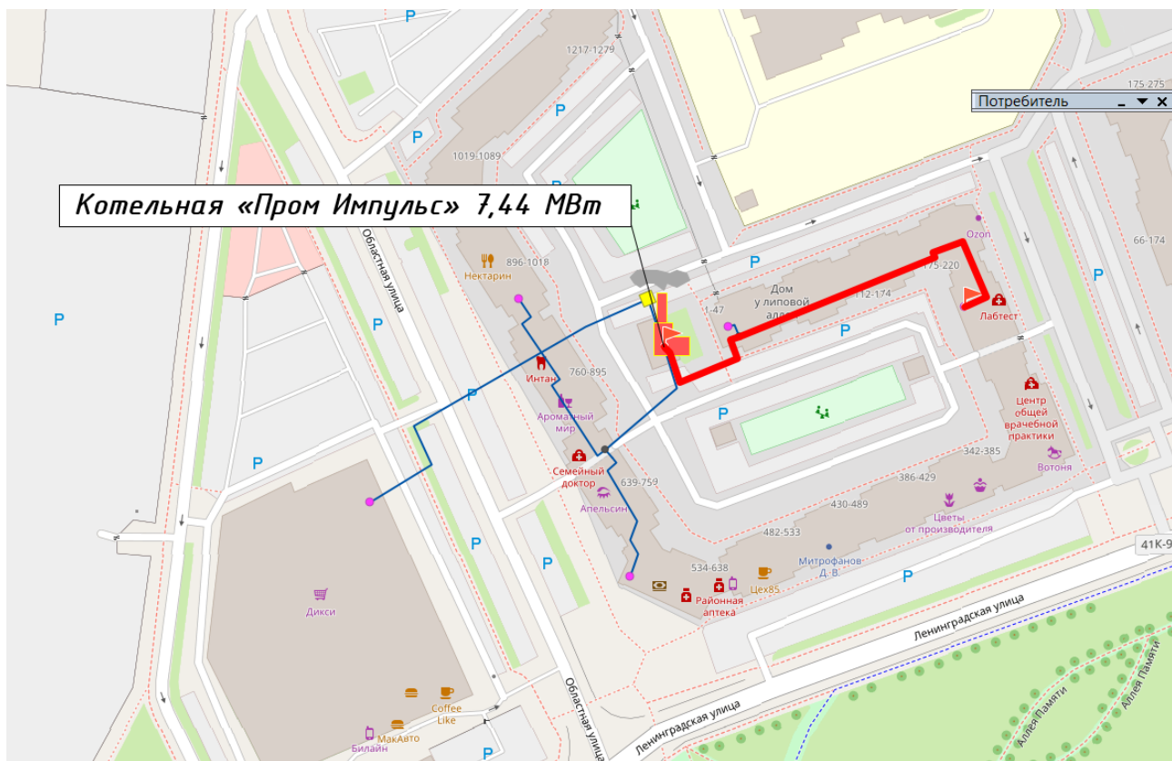
Рисунок 40. Путь построения пьезометрического графика от котельной 7,44 МВт до потребителя по ул.Ленинградской, 3
