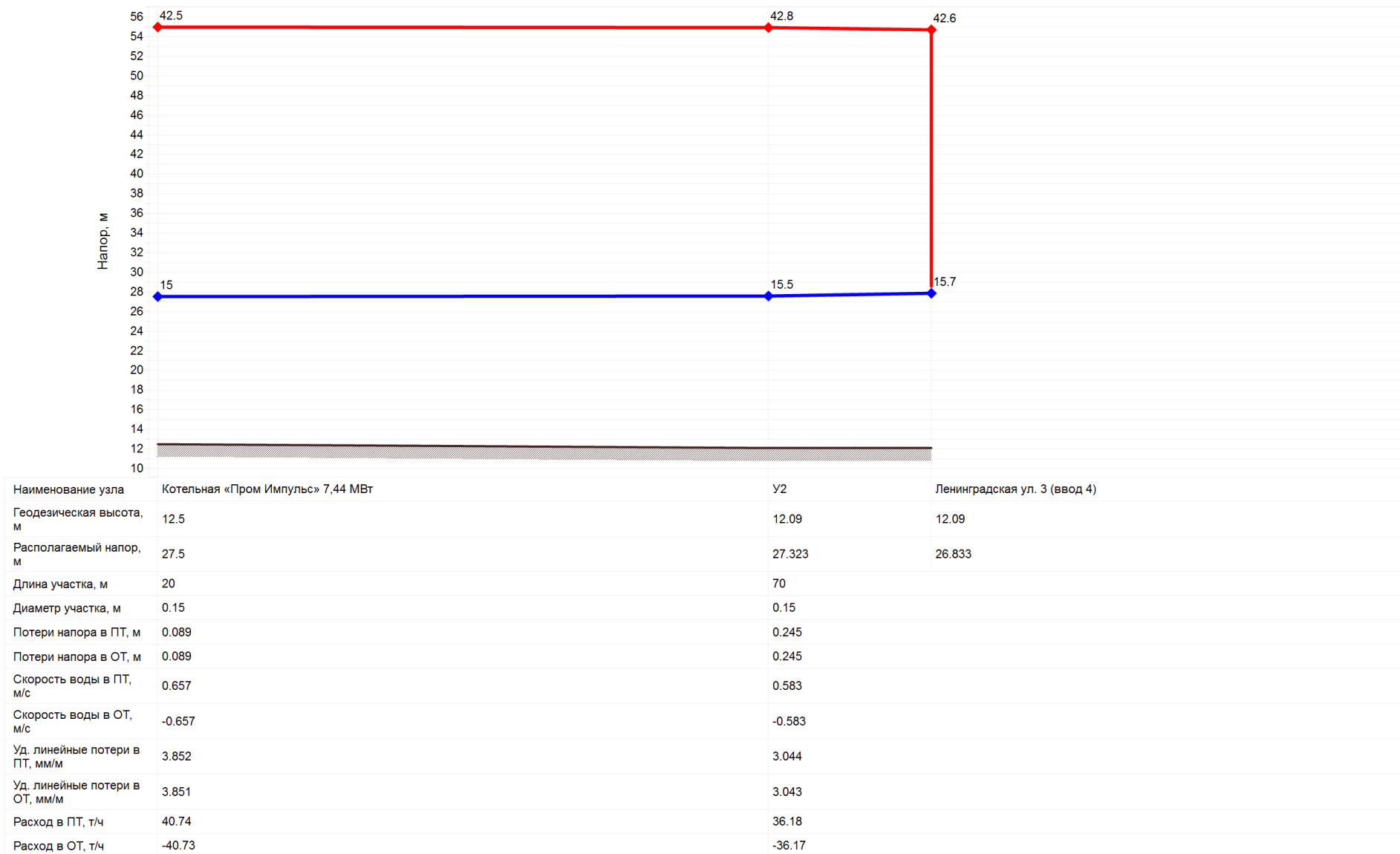
Рисунок 41. Пьезометрический график от котельной 7,44 МВт ООО «Пром Импульс» до потребителя на ул. Ленинградской,3
