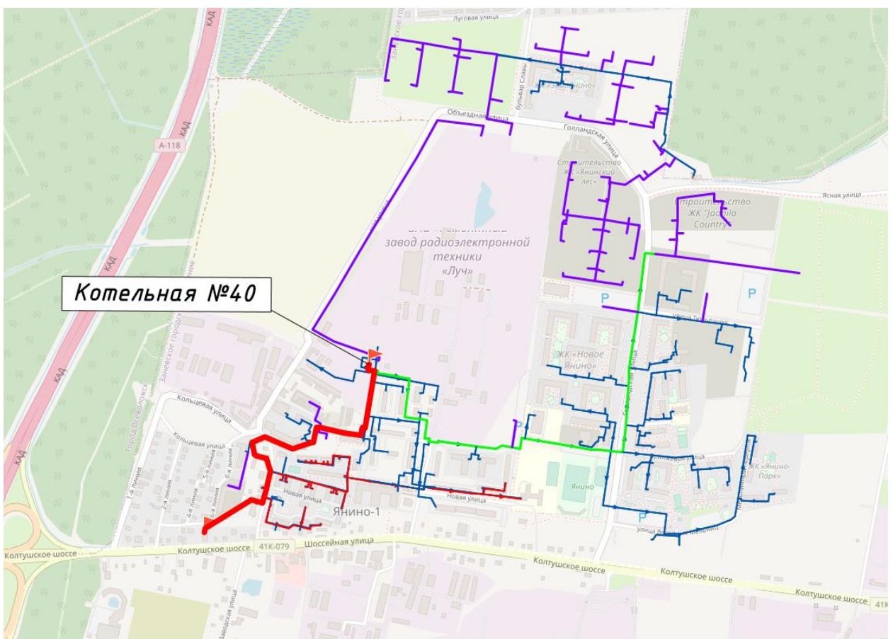
Рисунок 16. Путь построения №2 пьезометрического графика от котельной №40 ООО «СМЭУ «Заневка» до потребителя на ул. Шоссейная 15
