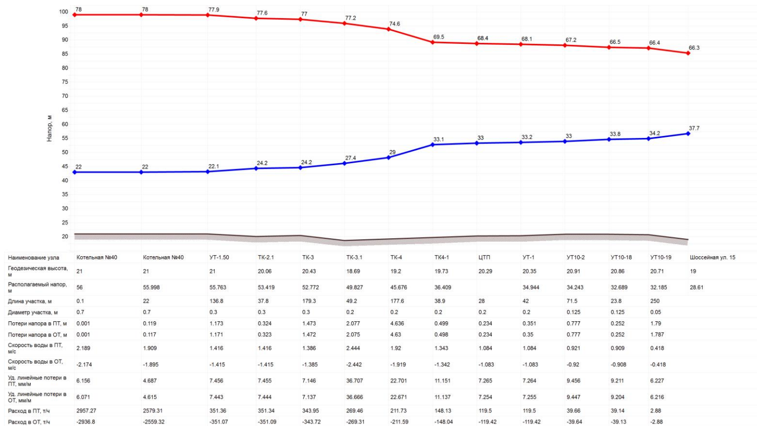
Рисунок 2. Пьезометрический график №2 от котельной № 40 ООО «СМЭУ «Заневка»
