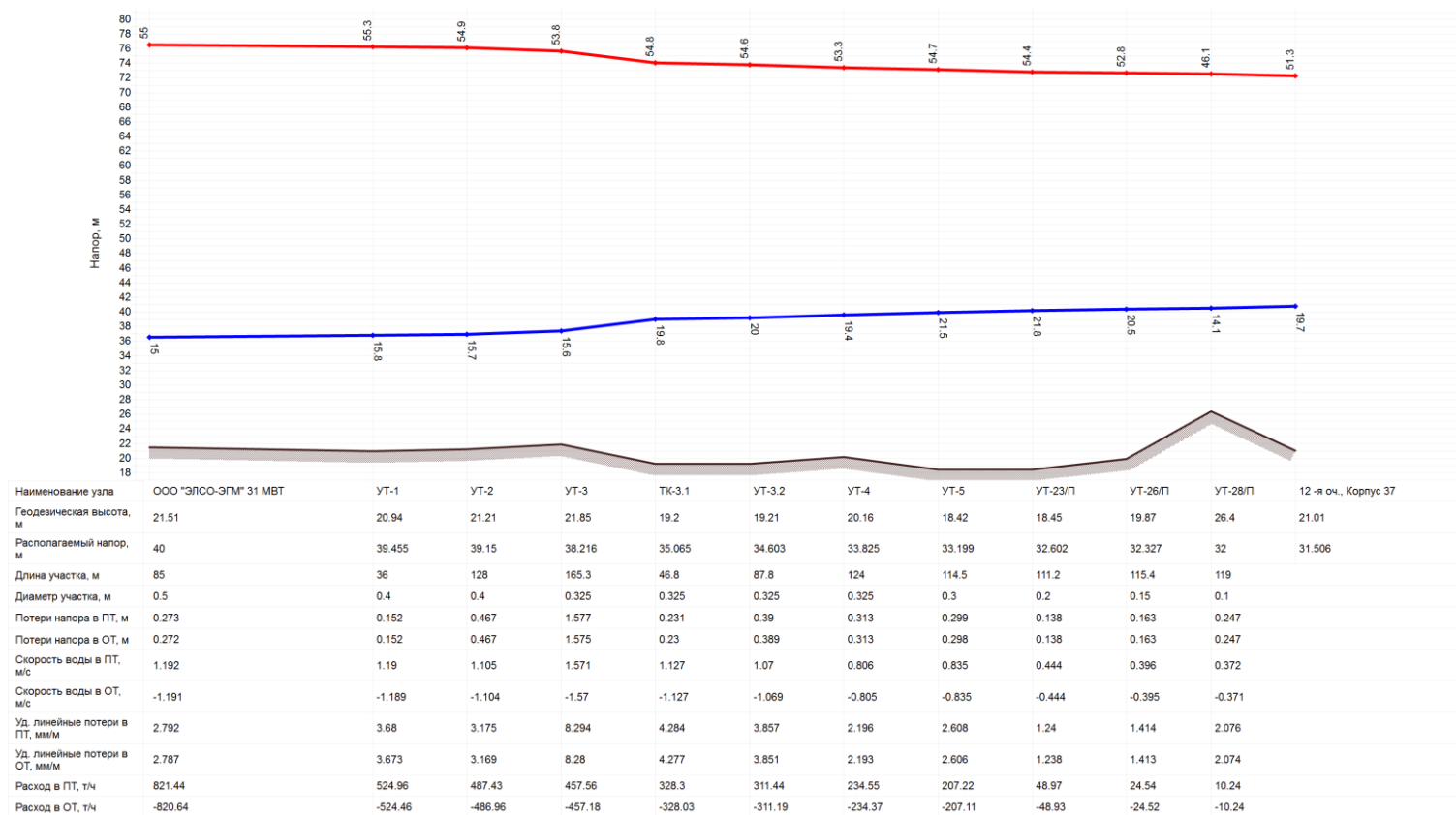
Рисунок 10. Пьезометрический график №1 от котельной ООО «ЭЛСО-ЭГМ» 31 МВт
