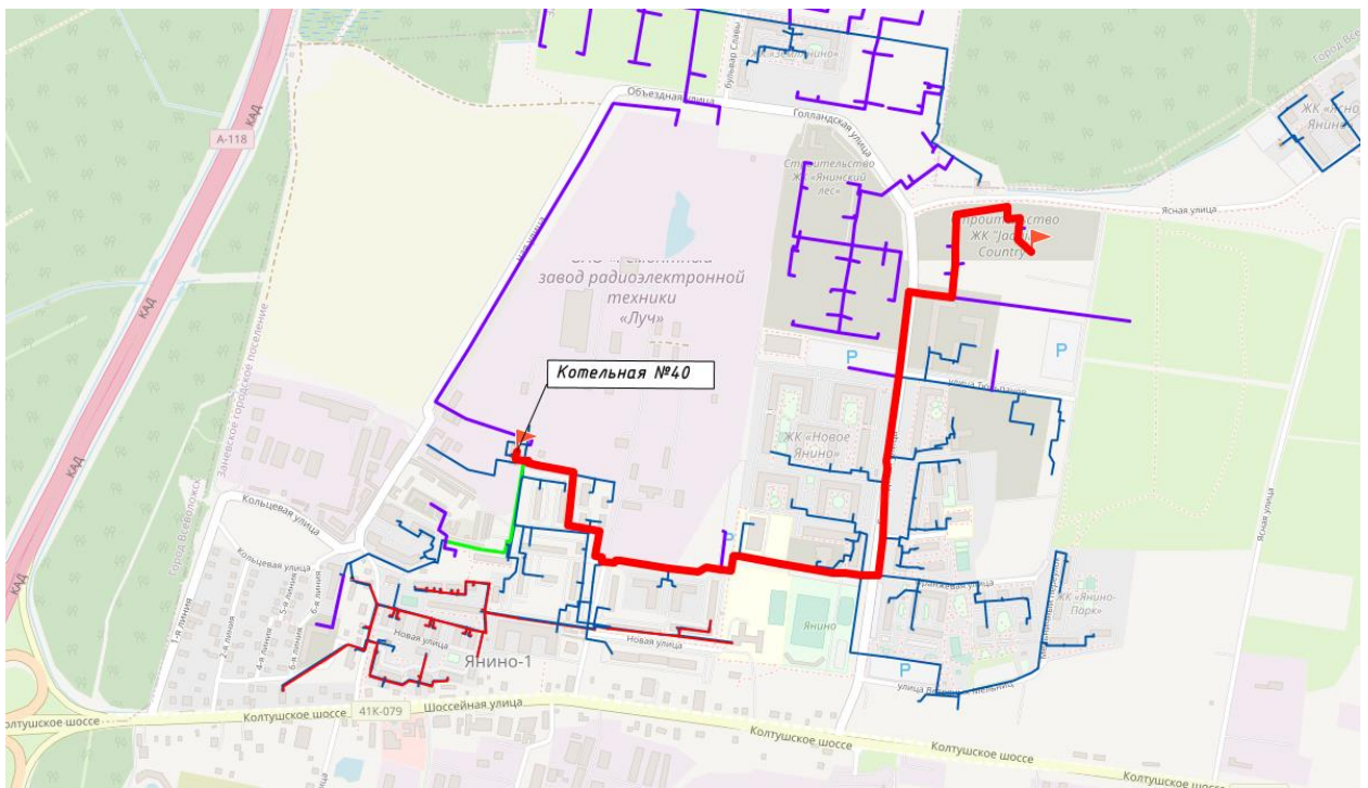
Рисунок 15. Путь построения №1 пьезометрического графика от котельной №40 ООО «СМЭУ «Заневка» до потребителя ДДОУ уч. 21
