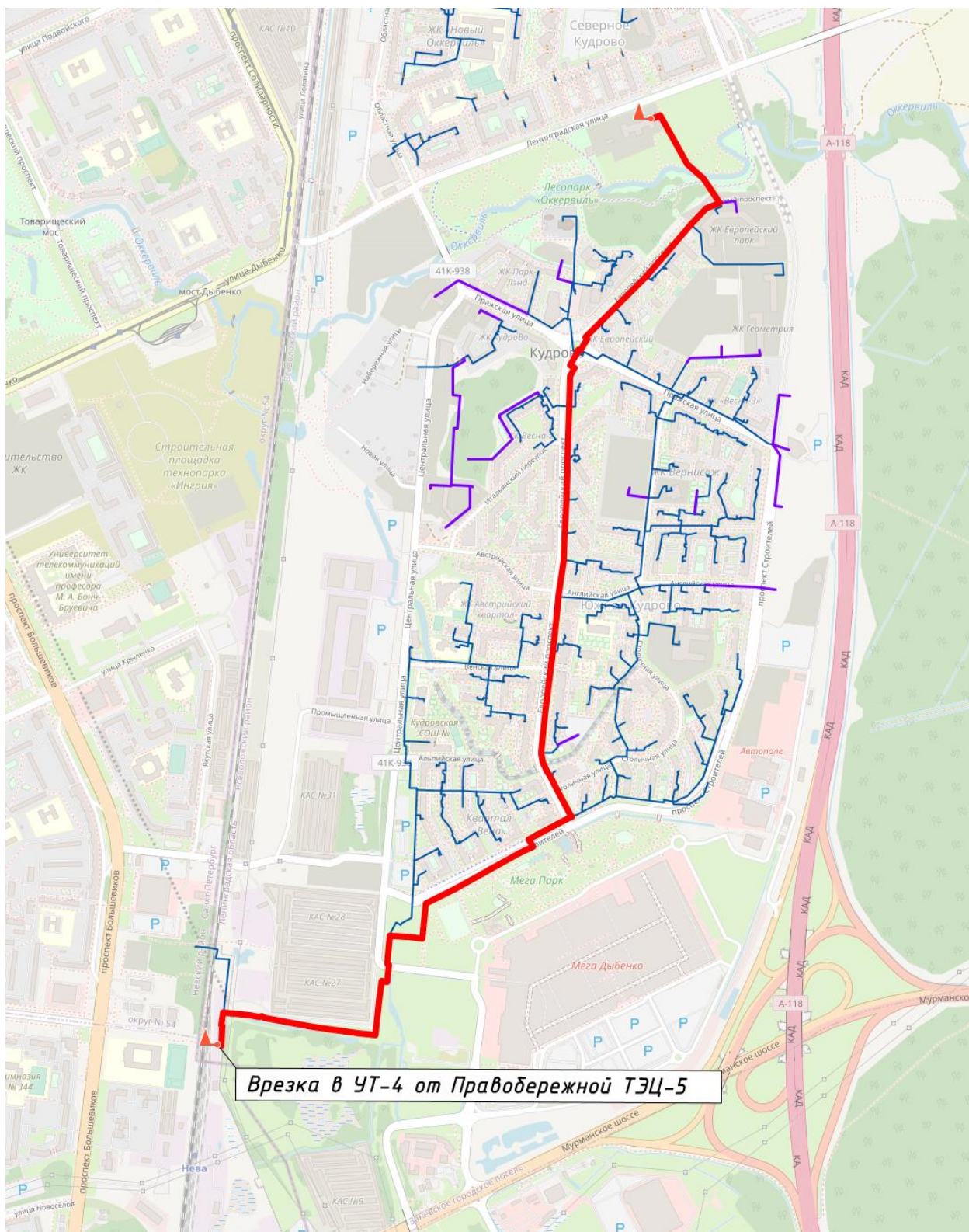
Рисунок 17. Путь построения №1 пьезометрического графика от УТ-4 в системе теплоснабжения АО «Теплосеть Санкт-Петербурга»
