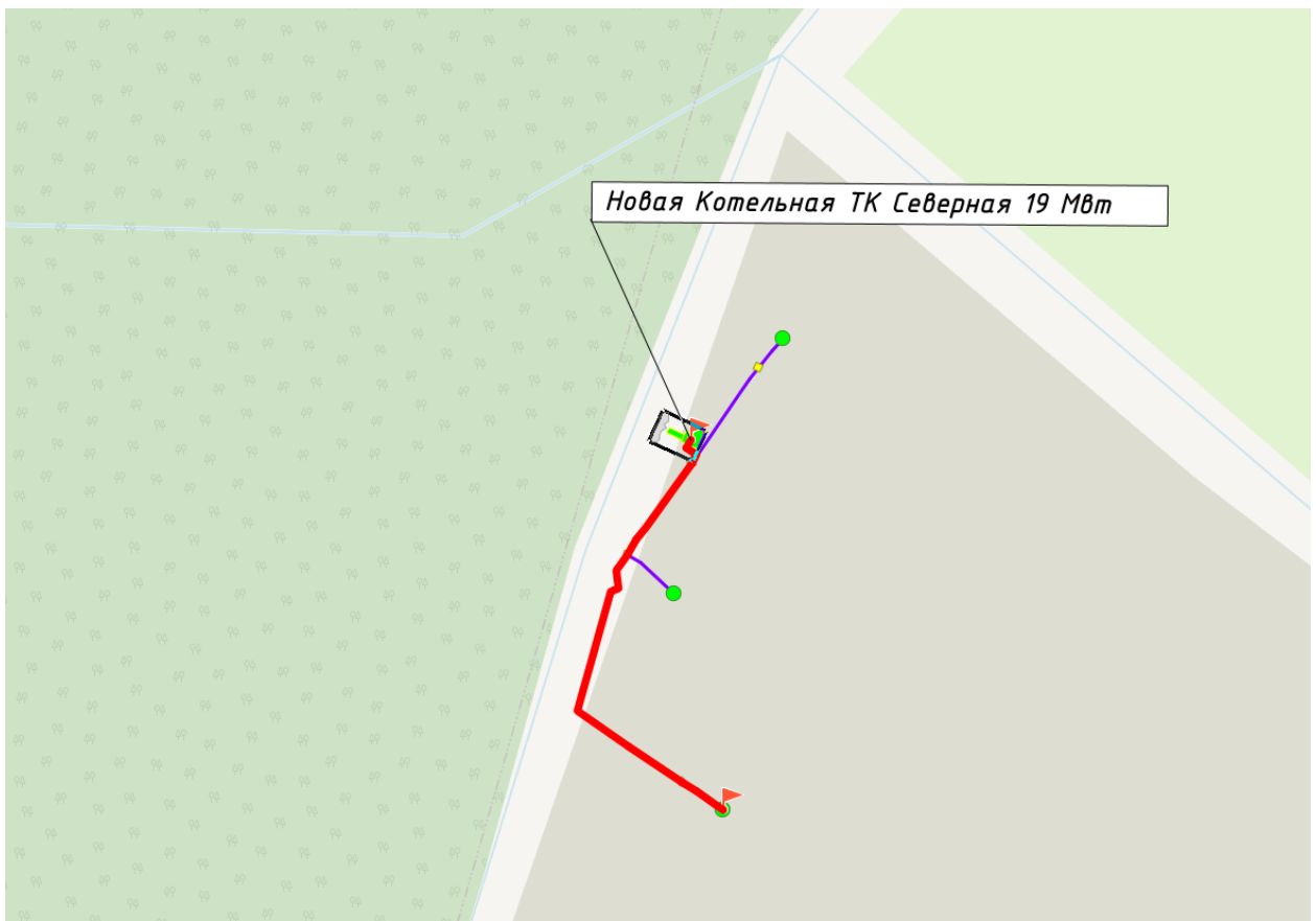
Рисунок 22. Путь построения пьезометрического графика от новой котельной 19 МВт ООО «Тепловая Компания Северная»
