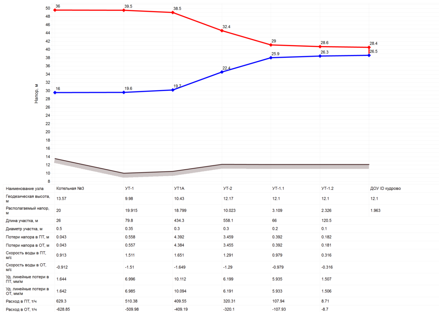
Рисунок 7. Пьезометрический график от котельной №3 ООО «Энергия»
