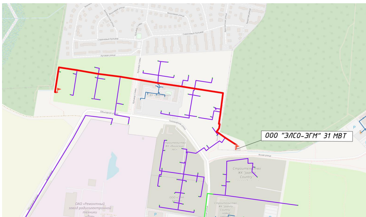
Рисунок 24. Путь построения №1 пьезометрического графика от котельной ООО «ЭЛСО-ЭГМ» 31 МВт
