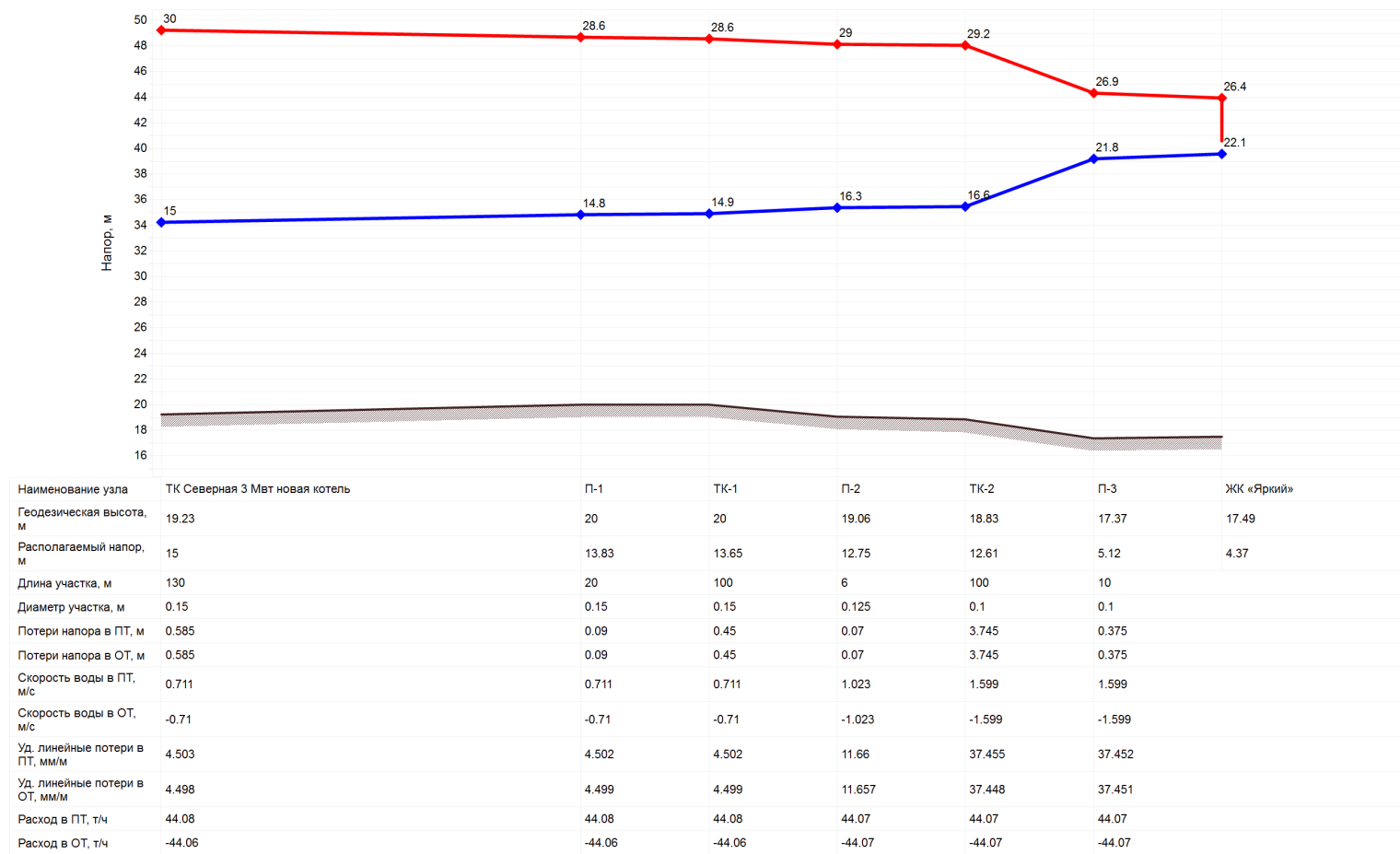
Рисунок 9. Пьезометрический график от новой котельной 3 МВт ООО «Тепловая Компания Северная»
