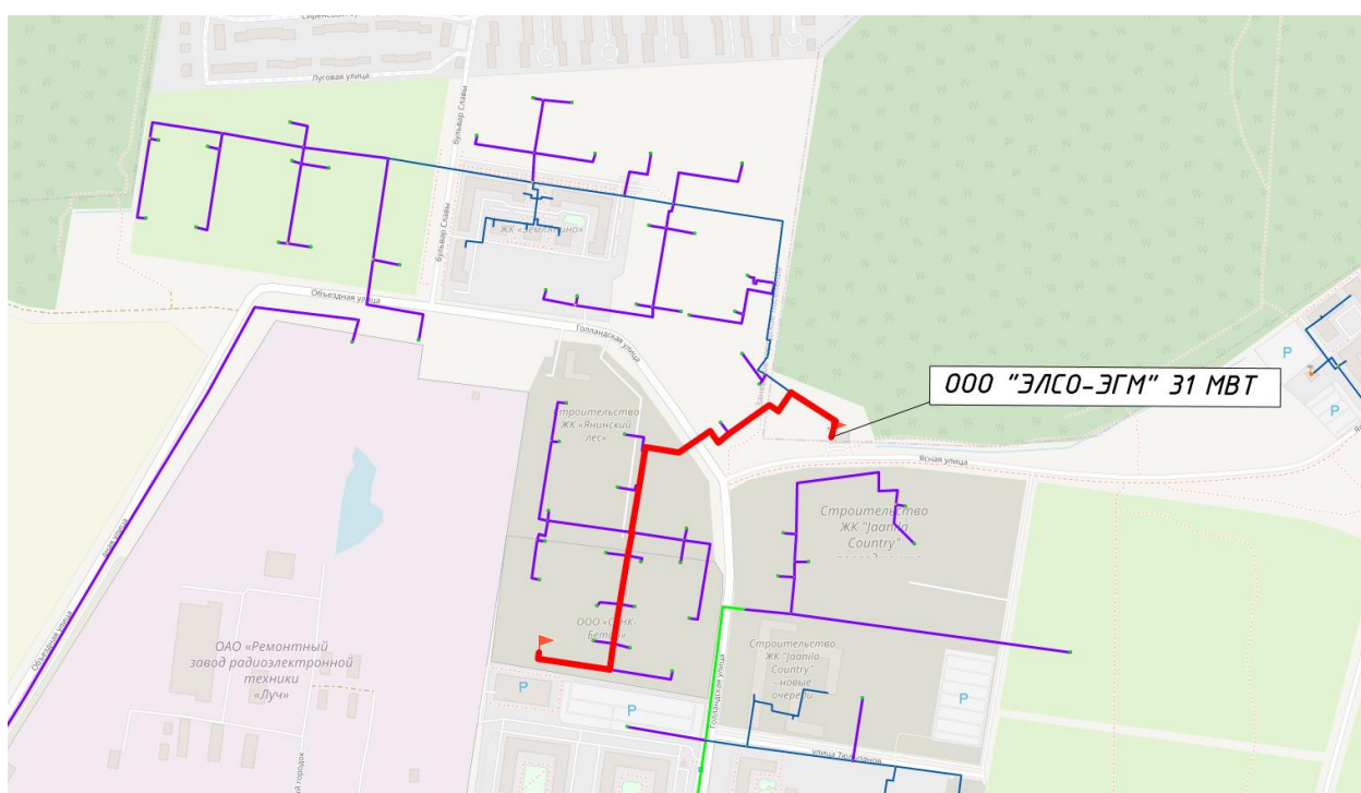
Рисунок 25. Путь построения №2 пьезометрического графика от котельной ООО «ЭЛСО-ЭГМ» 31 МВт
