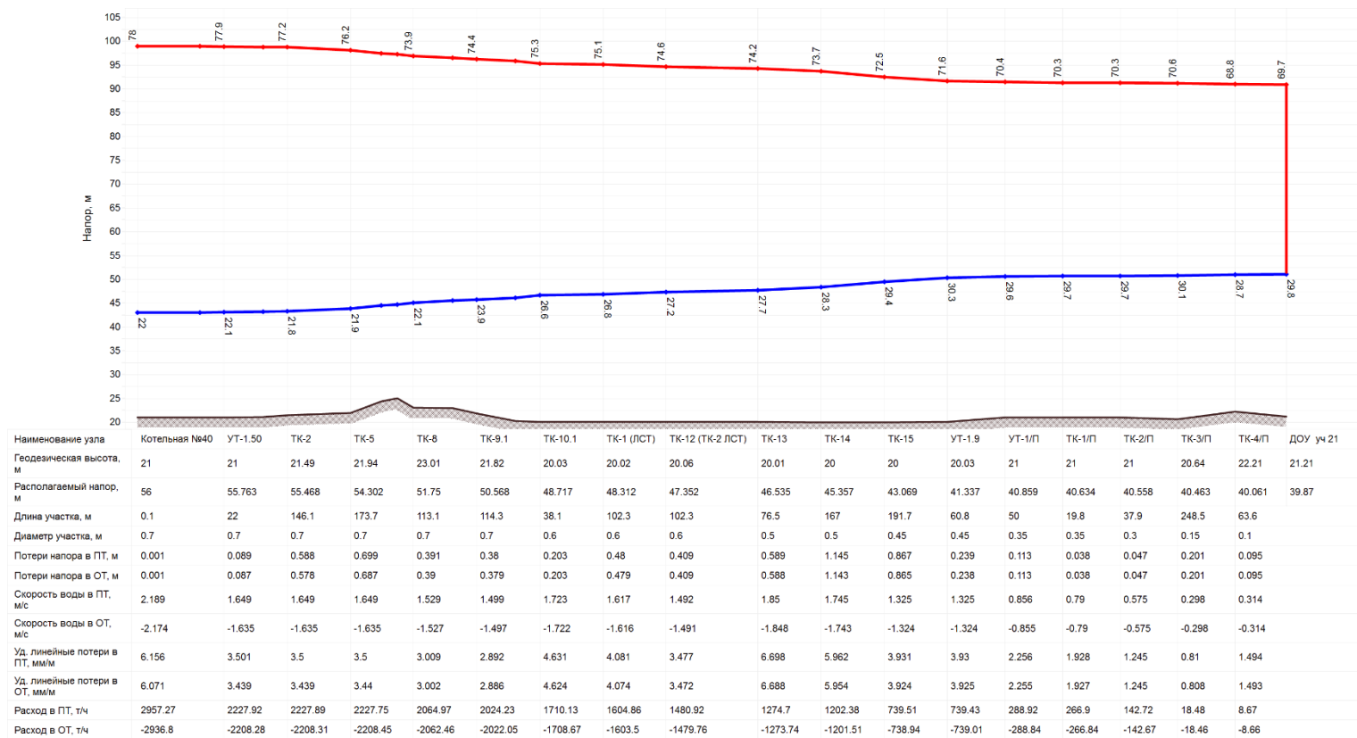
Рисунок 1. Пьезометрический график №1 от котельной № 40 ООО «СМЭУ «Заневка»
