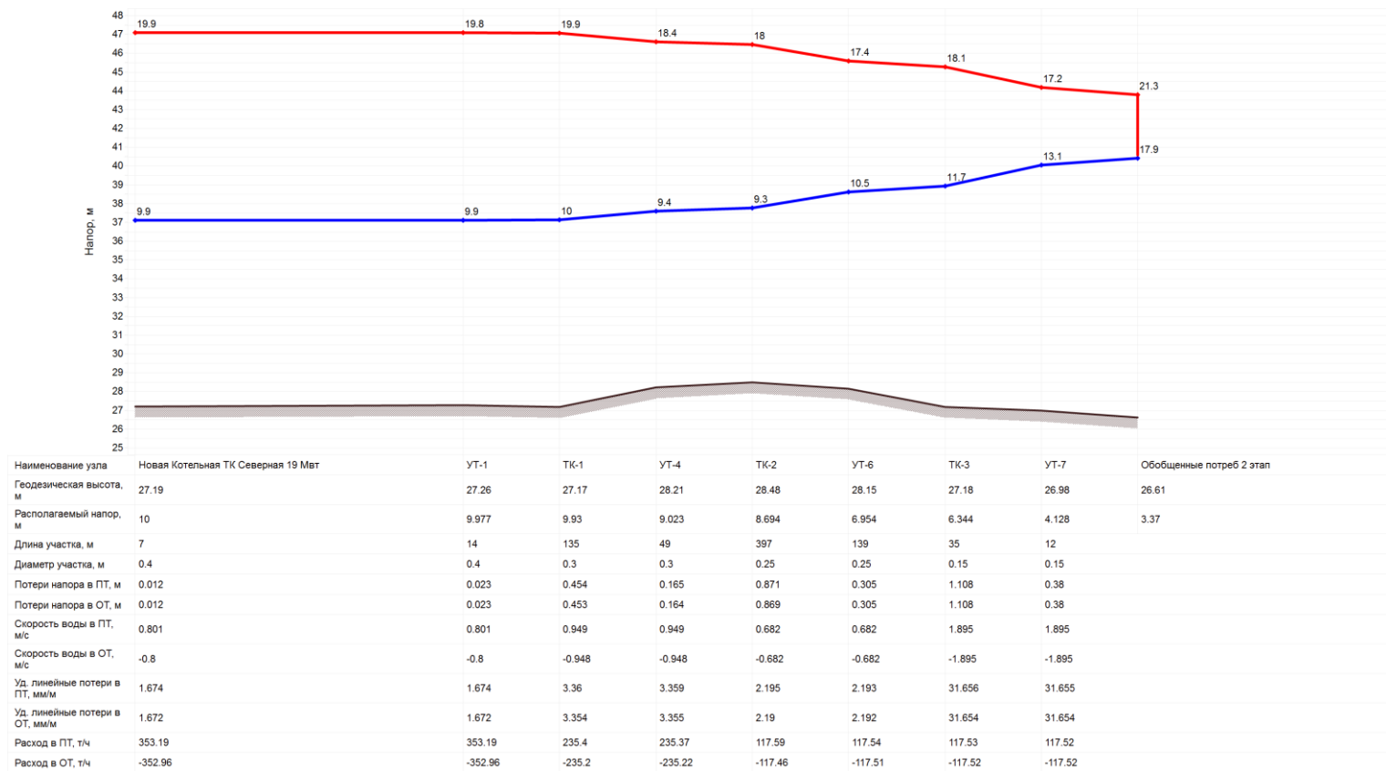
Рисунок 8. Пьезометрический график от новой котельной 19 МВт ООО «Тепловая Компания Северная»
